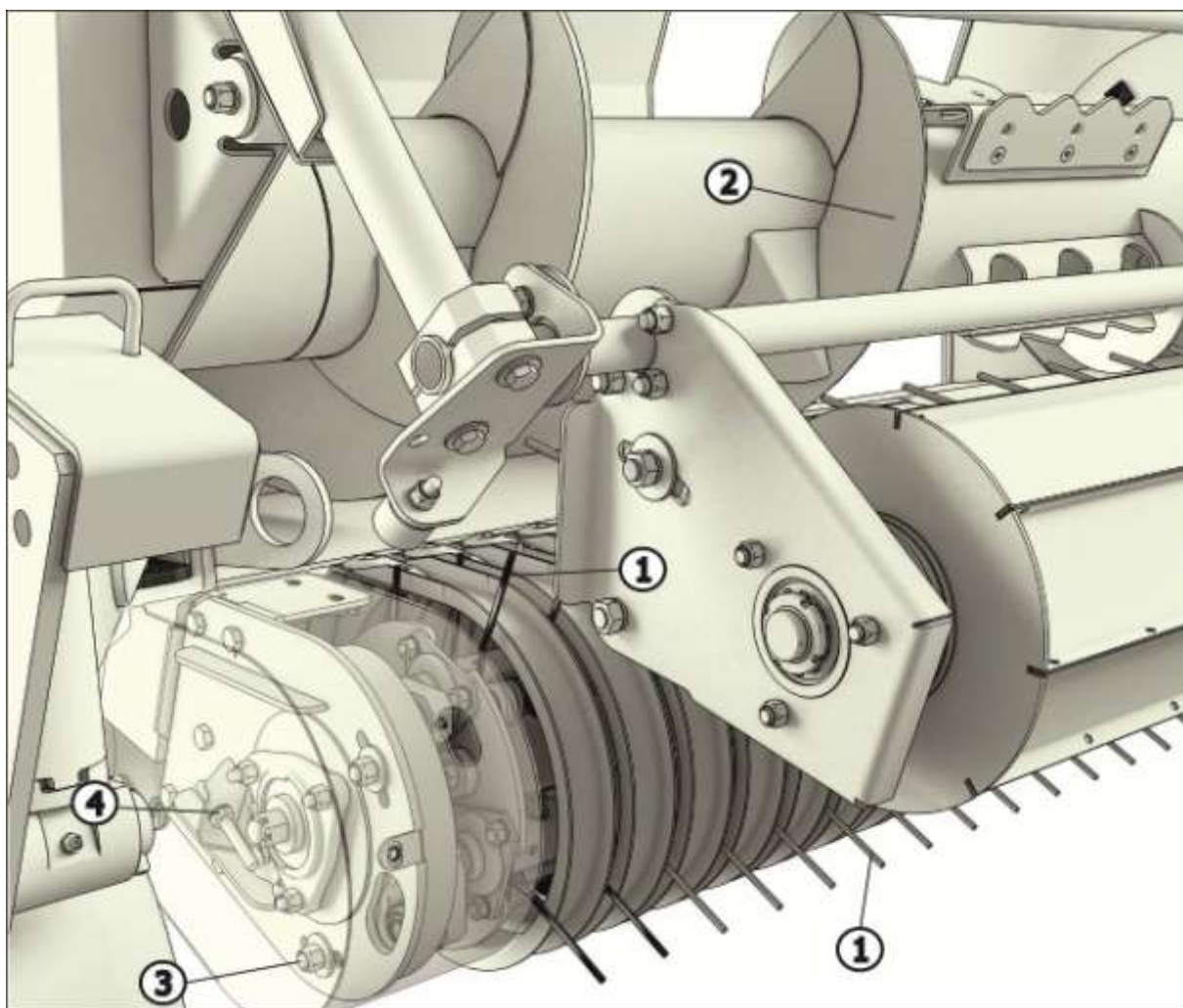
1- палец подбирающий; 2 - виток шнека; 3 – болт крепеж; 4-гайка
