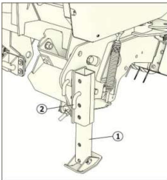
1-опора; 2-фиксатор;
