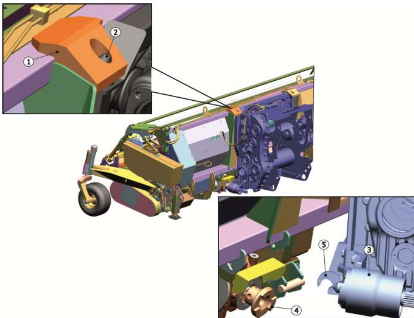
Рисунок 5.1- Навеска ППК-403 на комбайн F2650
