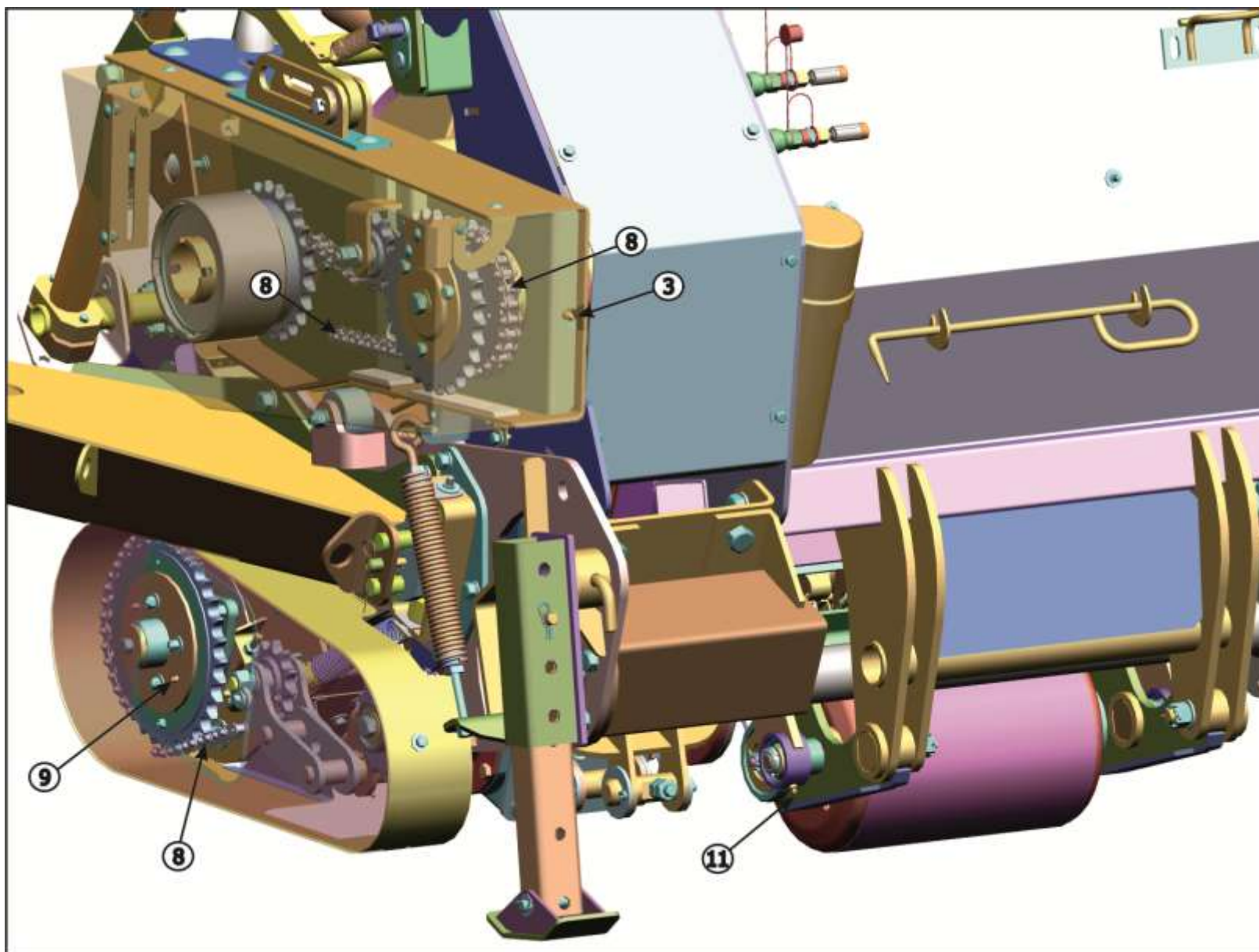
Риунок 7.3 – Смазка подборщика
