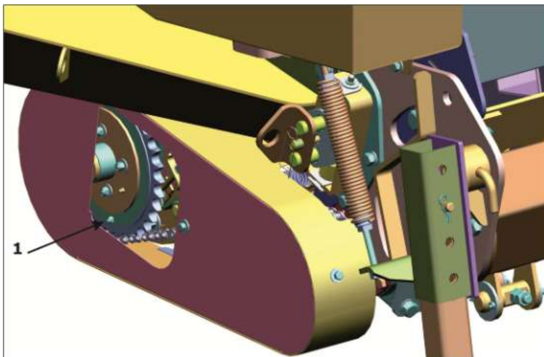
1-срезной болт
