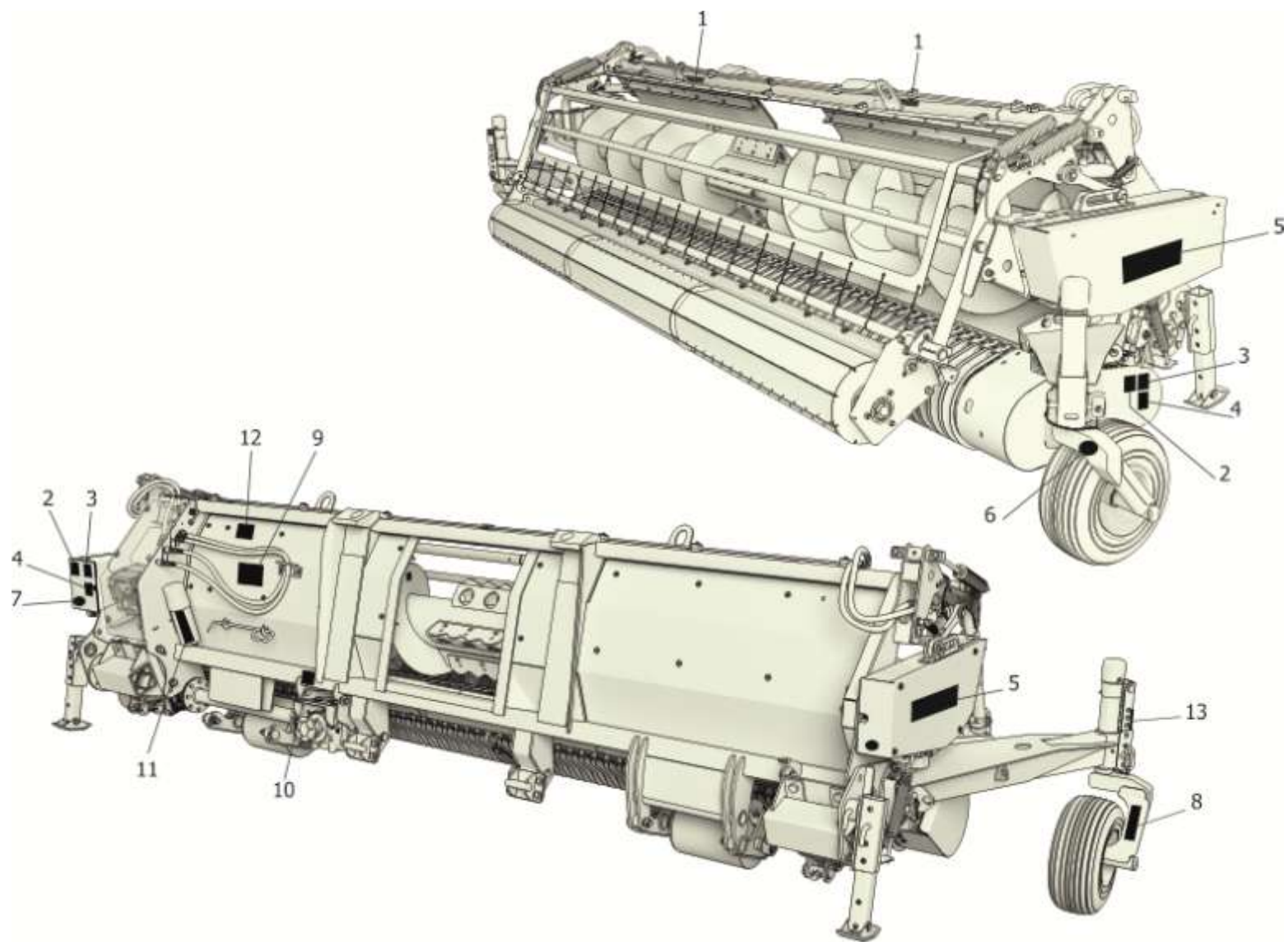
Рисунок 4.2 – Места расположения табличек на ПК-403
