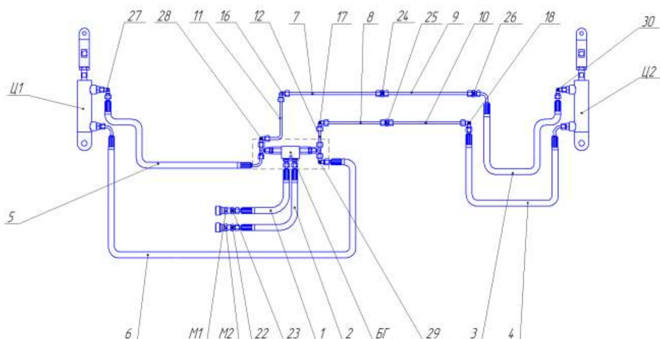
Рисунок В.1 – Схема гидравлических соединений ПК-403
