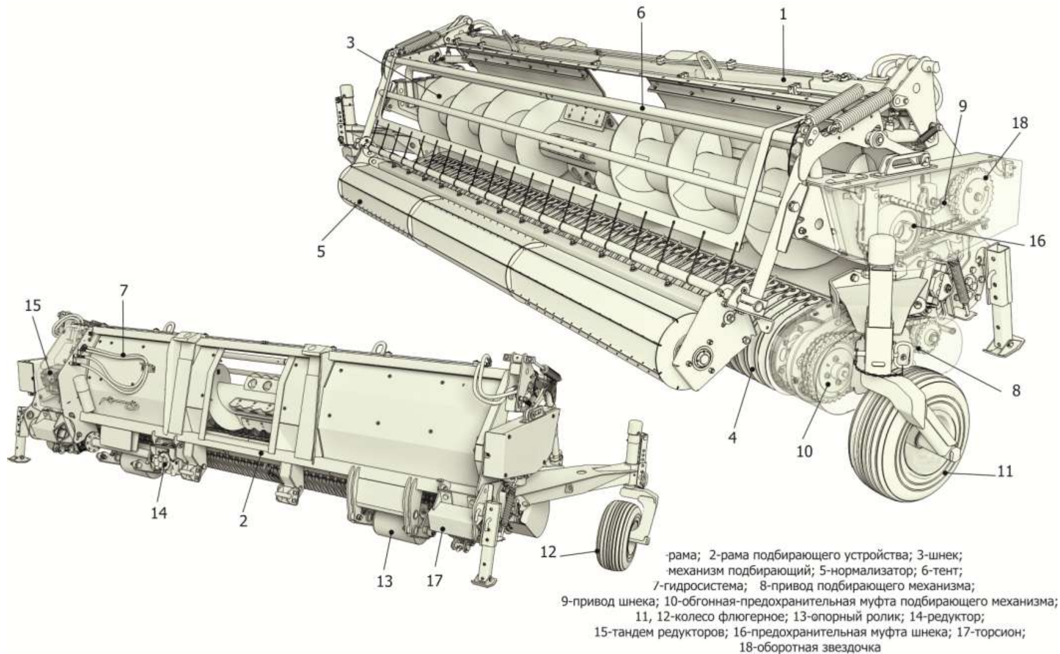
Рисунок 1.1 - Общий вид подборщика ПК-403
