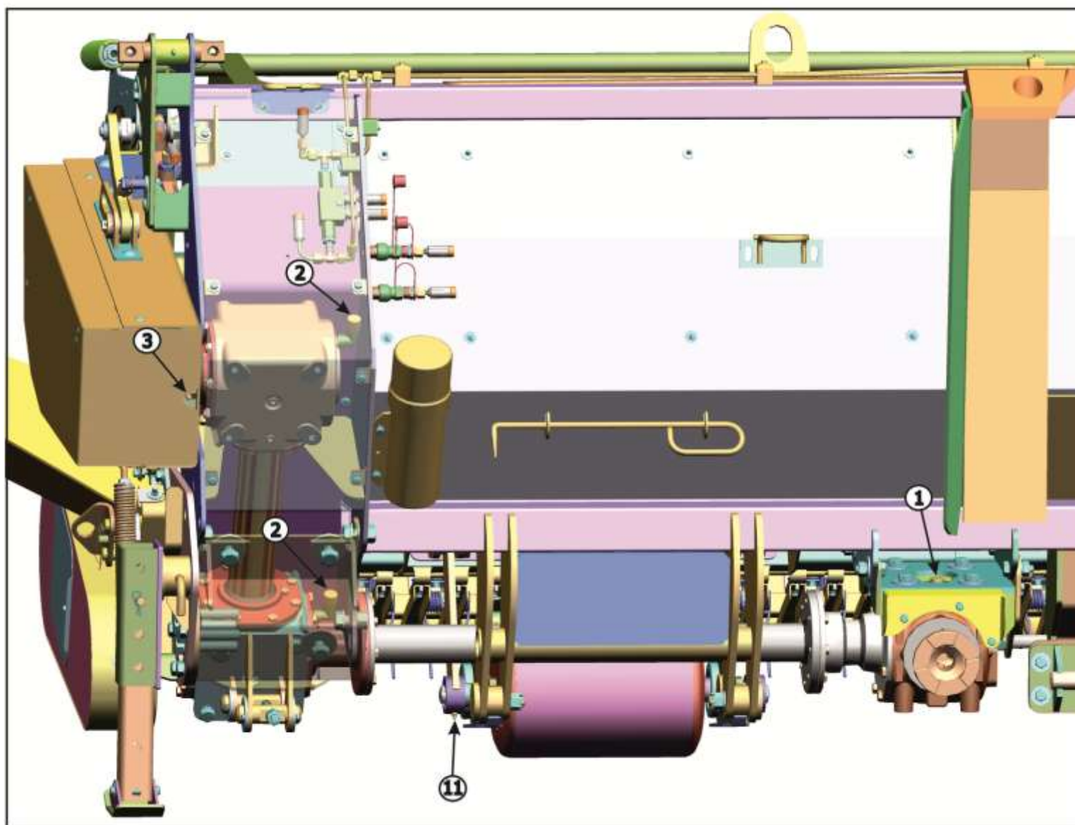
Рисунок 7.4 – Смазка подборщика
