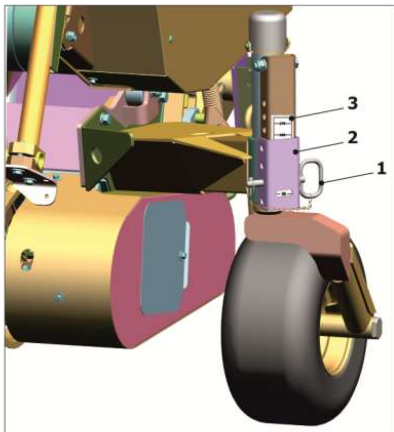
1-фиксатор; 2-кронштейн; 3-шкала
