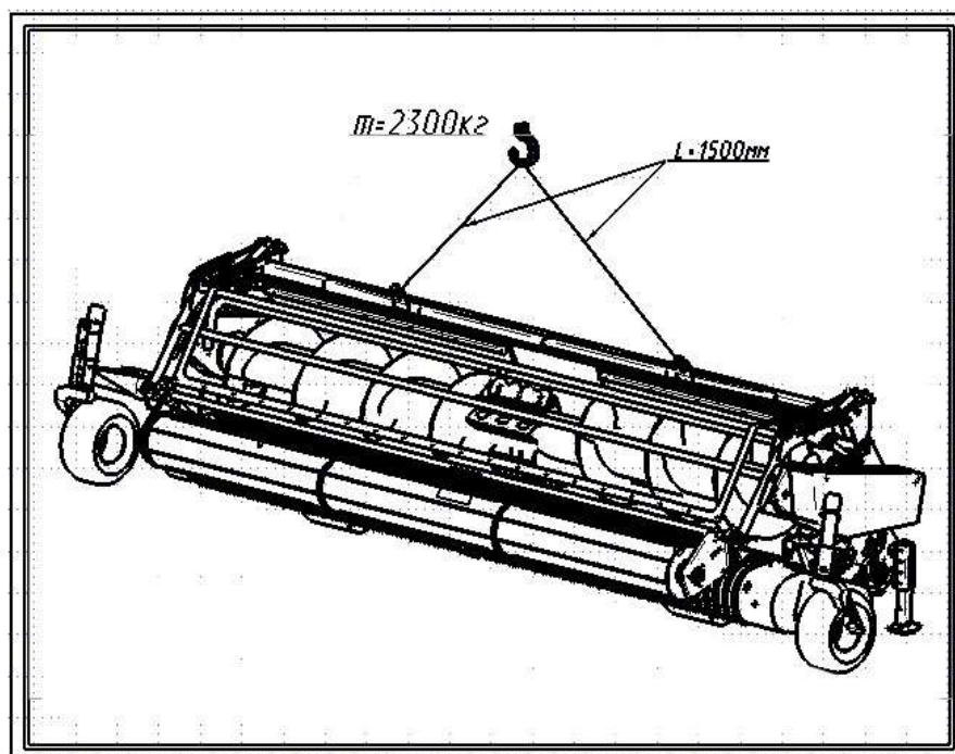
Рисунок 8.1 - Схема строповки ПК-403
