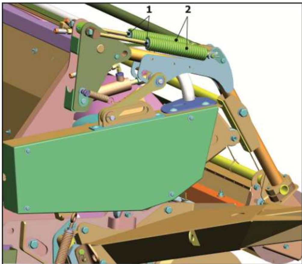
1-гайка; 2-пружина
