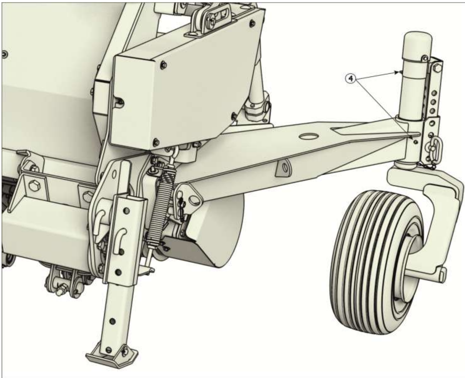
Рисунок 7.7 – Смазка подборщика
