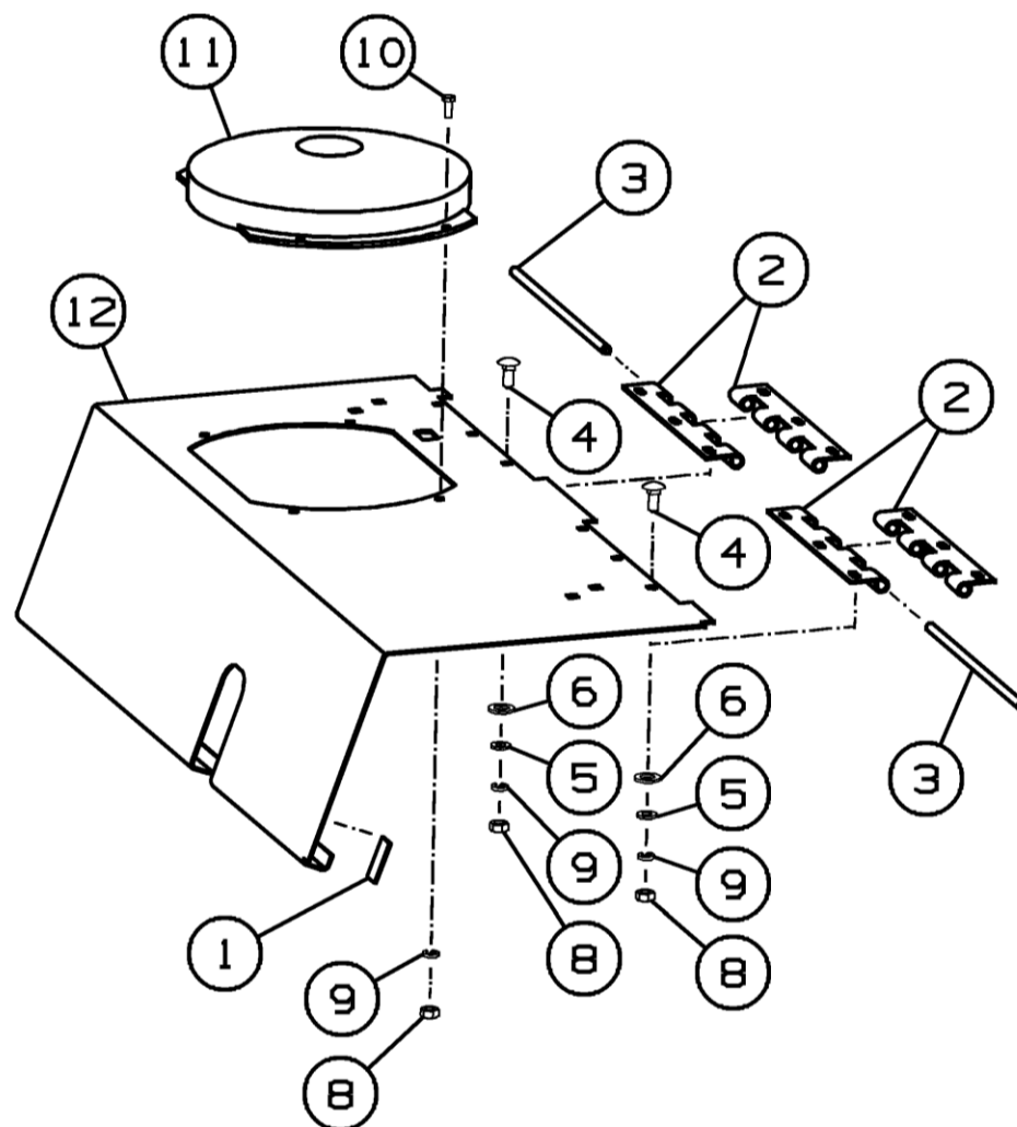
Рисунок 15 – Щиток ППТ-041.10.170 (для ППТ-041«Тукал»), ППТ-041.10.170-01 (для ППТ-041«Тукал Luxe»)
