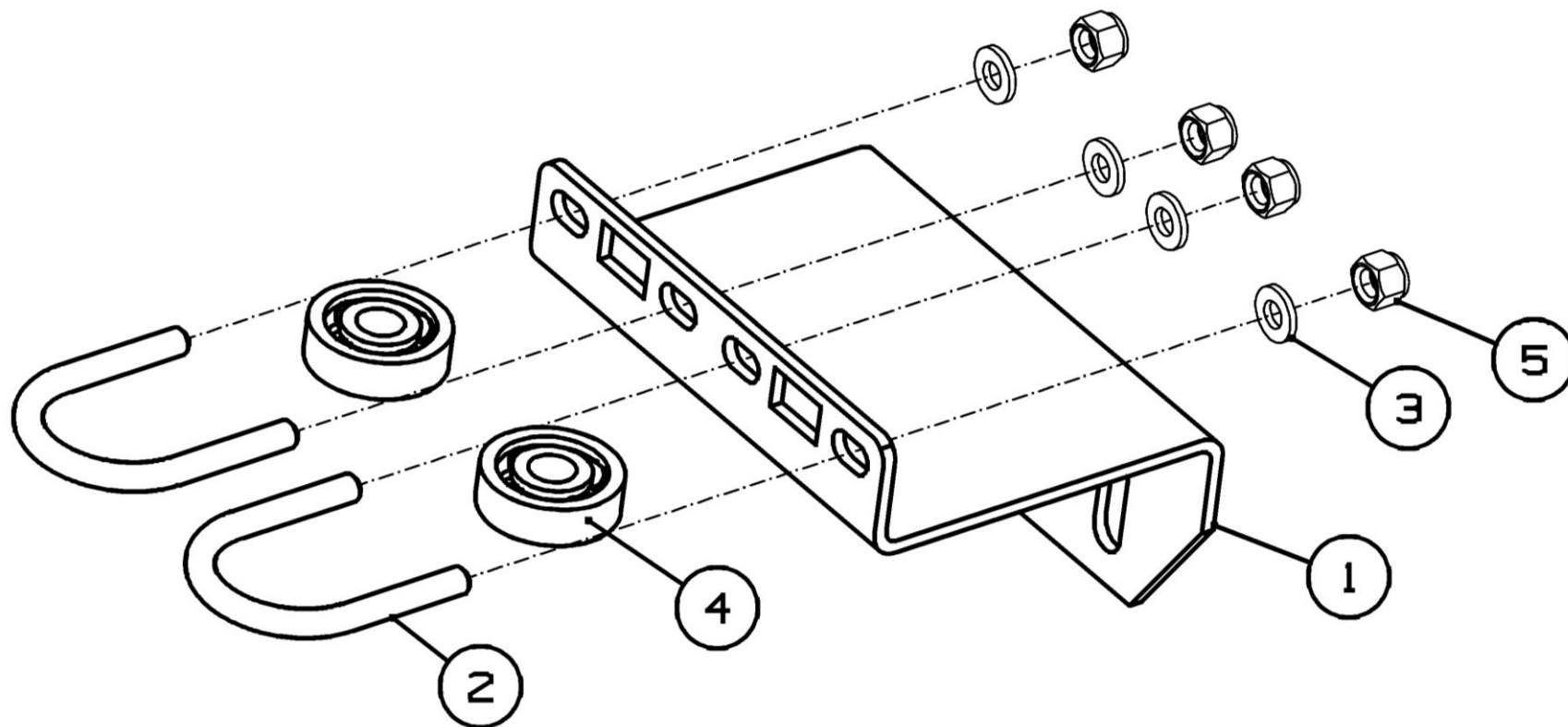
Рисунок 52 - Кронштейн глазков ППТ-041.01.030 «Tukan Luxe»
