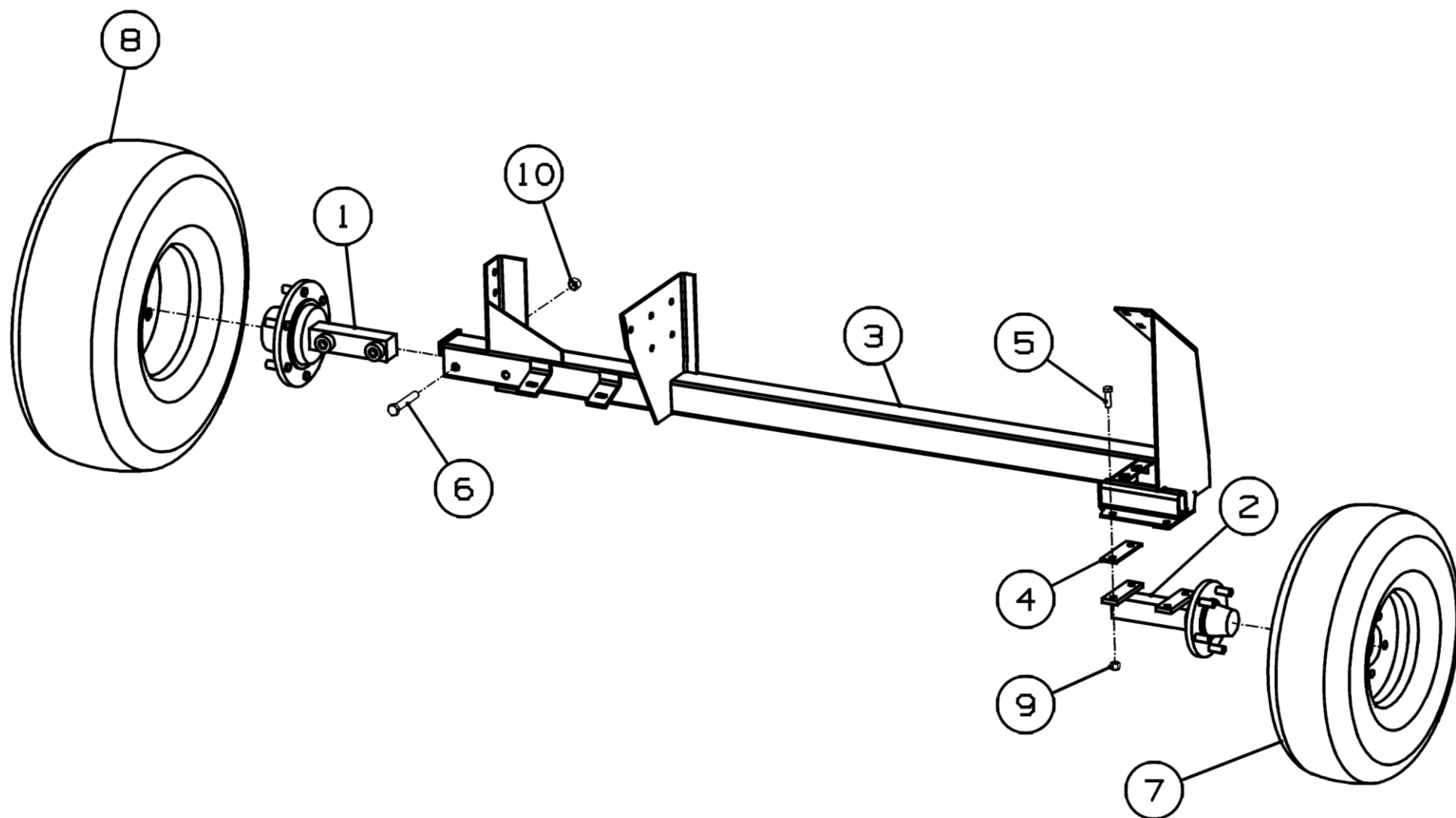
Рисунок 38 – Шасси ППТ-041.02.100
