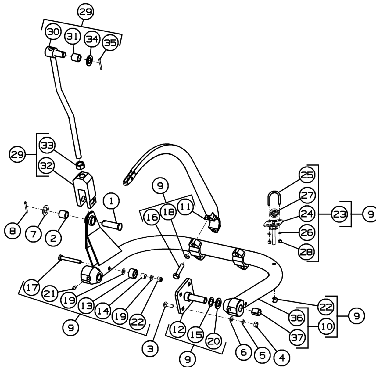
Рисунок 27 - Установка игл ППТ-041.01.200
