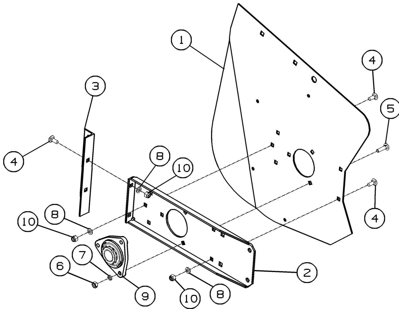
Рисунок 6 – Боковина левая ППТ-041.16.080
