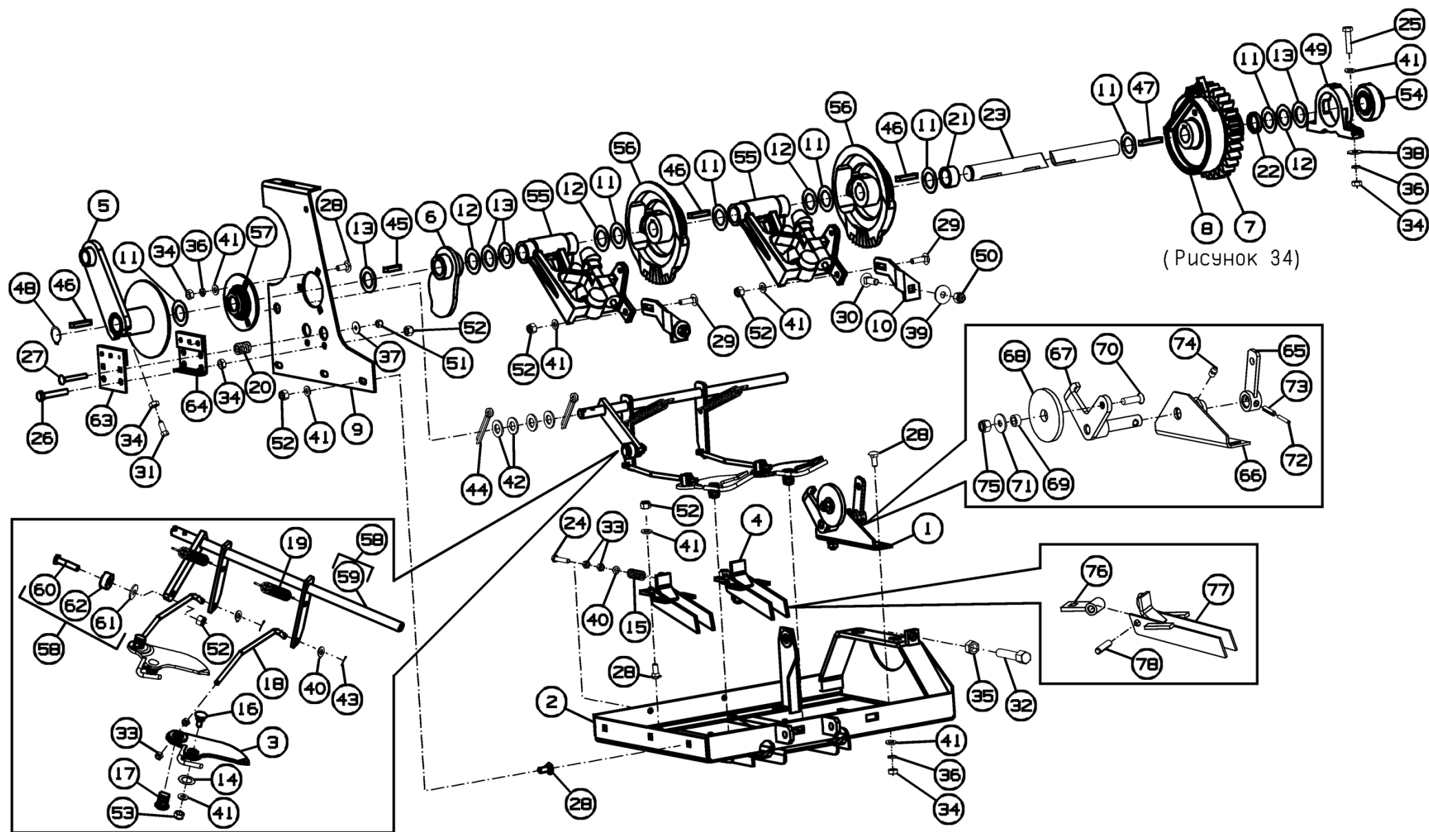
Рисунок 32 – Механизм обвязывающий ППТ-041.07.000
