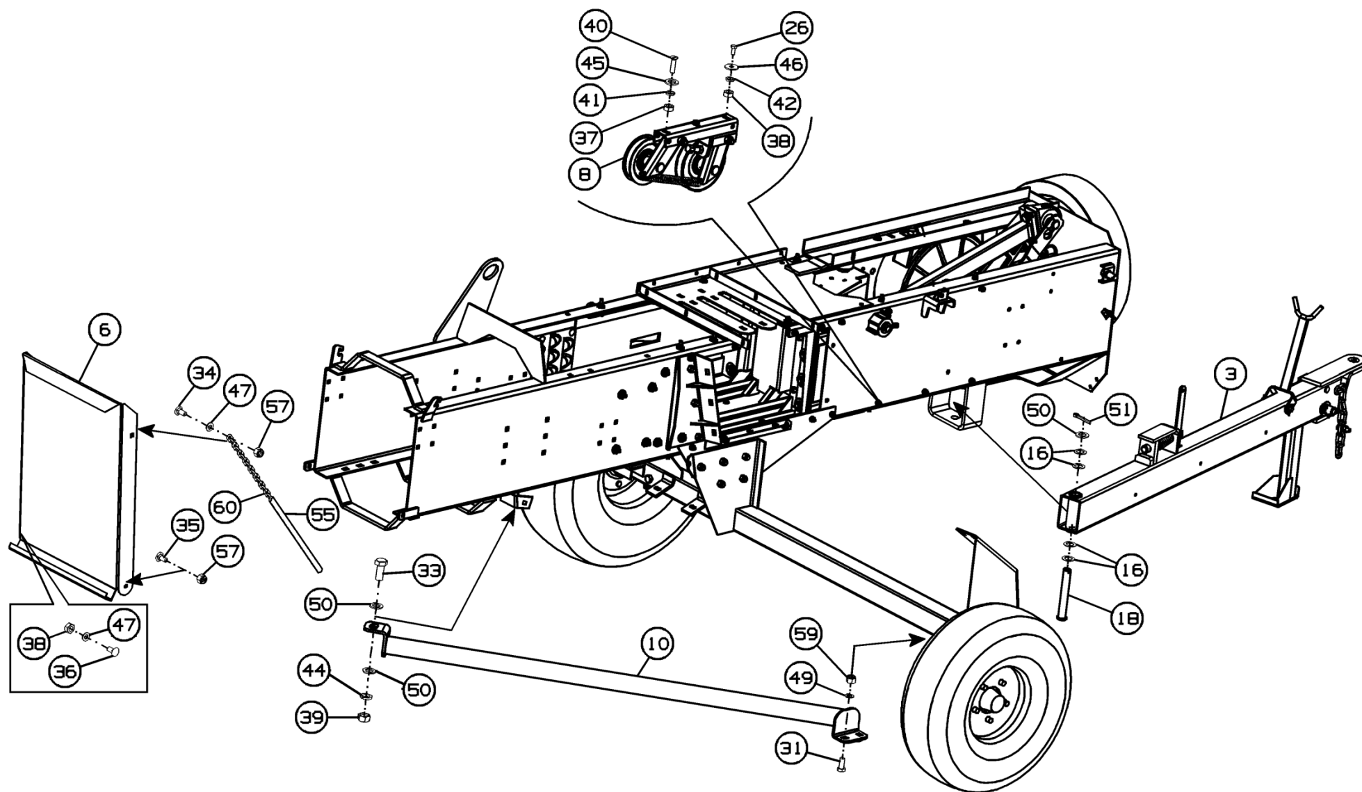
Рисунок 35 – Камера прессующая ППТ-041.12.000
