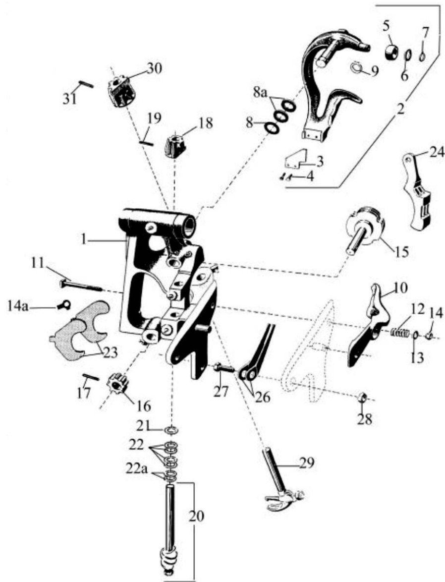
Рисунок 33 – Узловязатель 200.3770.21/51994
