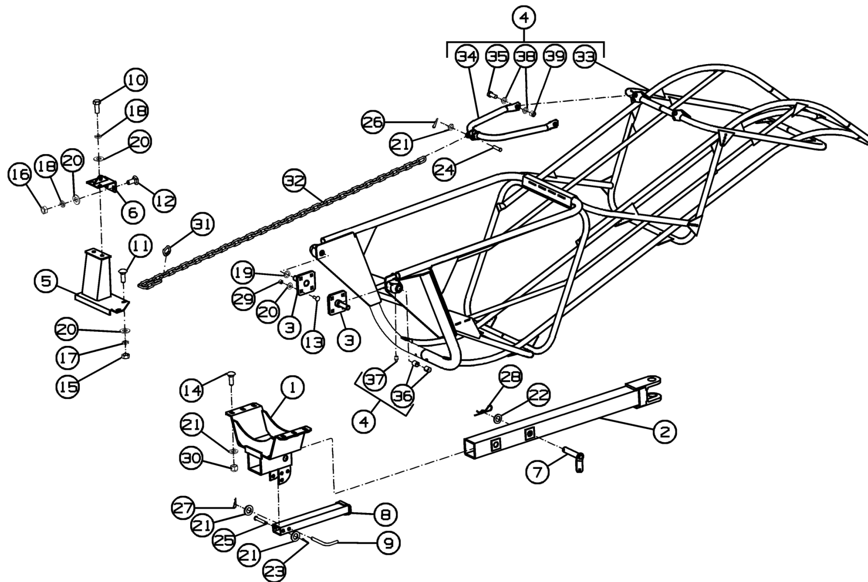
Рисунок 55 – Установка выгрузного устройства ППТ-041.40.000
