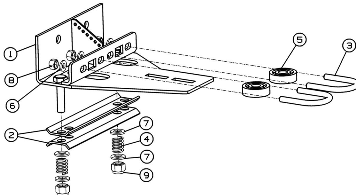
Рисунок 53 - Механизм натяжения шпата ППТ-041.01.040 «Tukan Luxe»
