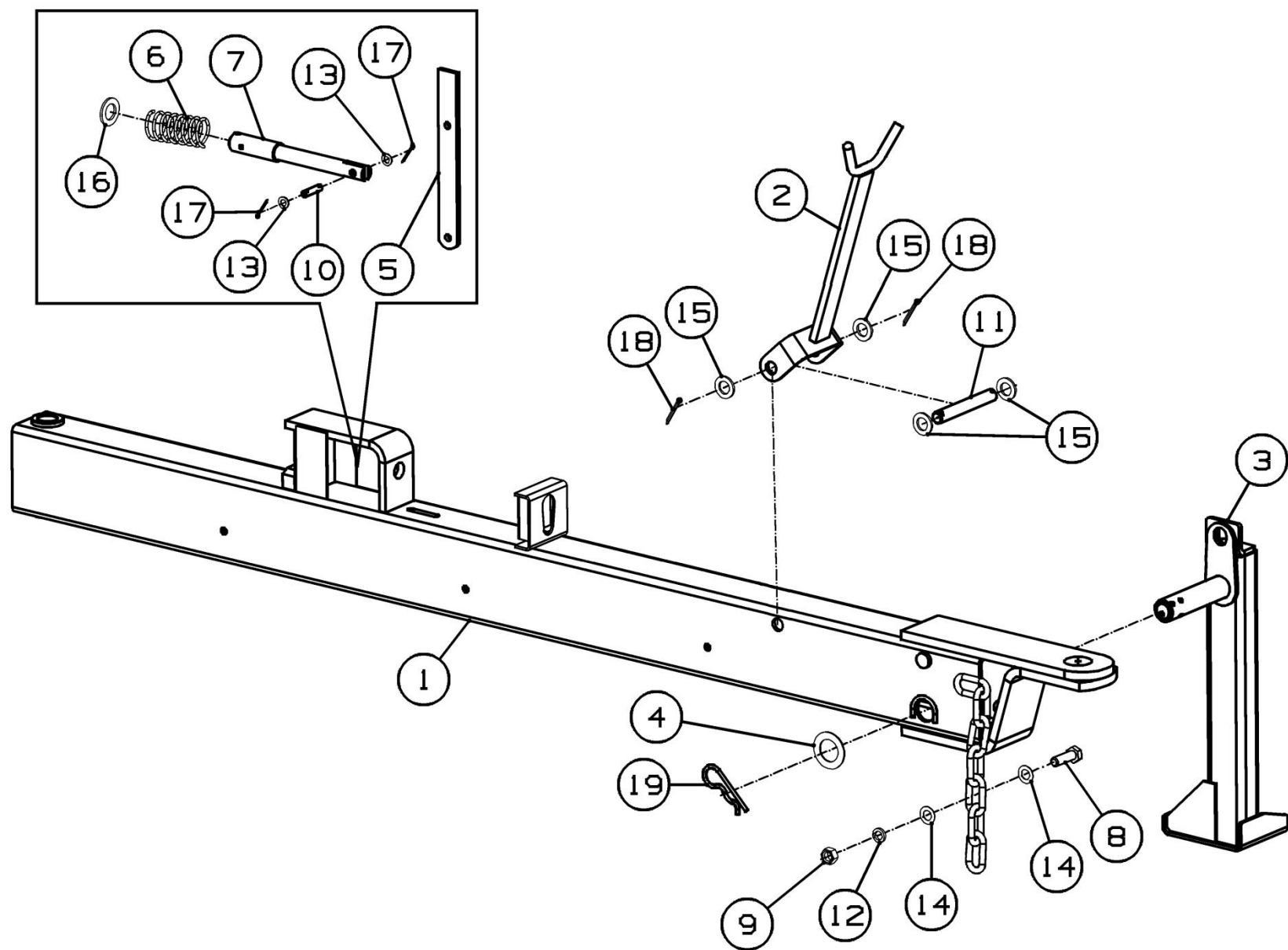
Рисунок 39 – Сница ППТ-041.02.300
