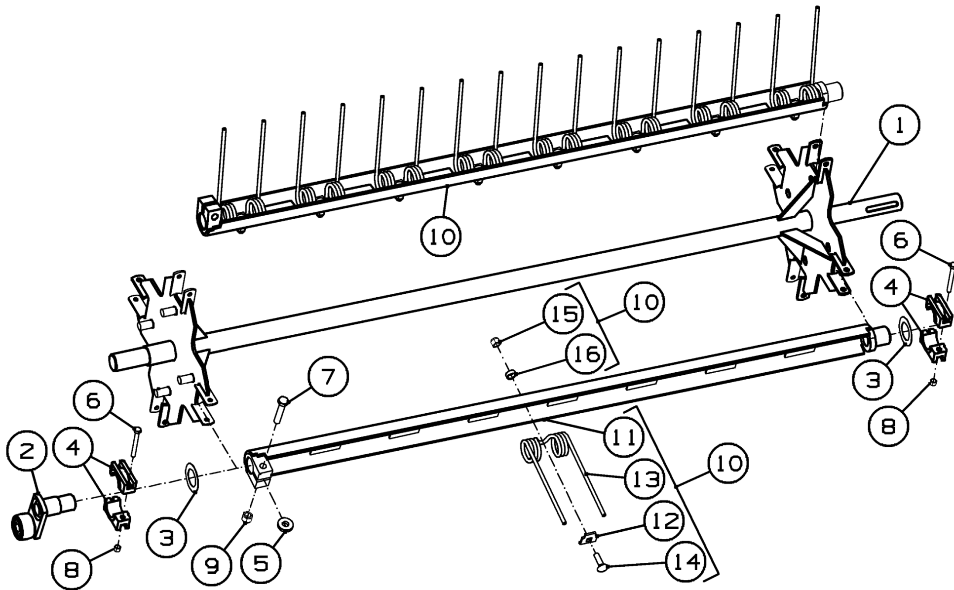
Рисунок 8 – Механизм подбирающий ППТ-041.16.010
