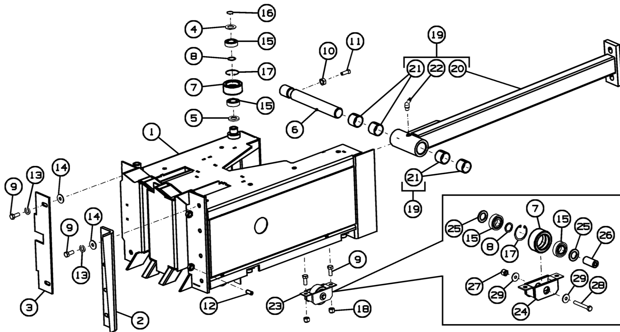
Рисунок 43 - Поршень ППТ-041.03.000
