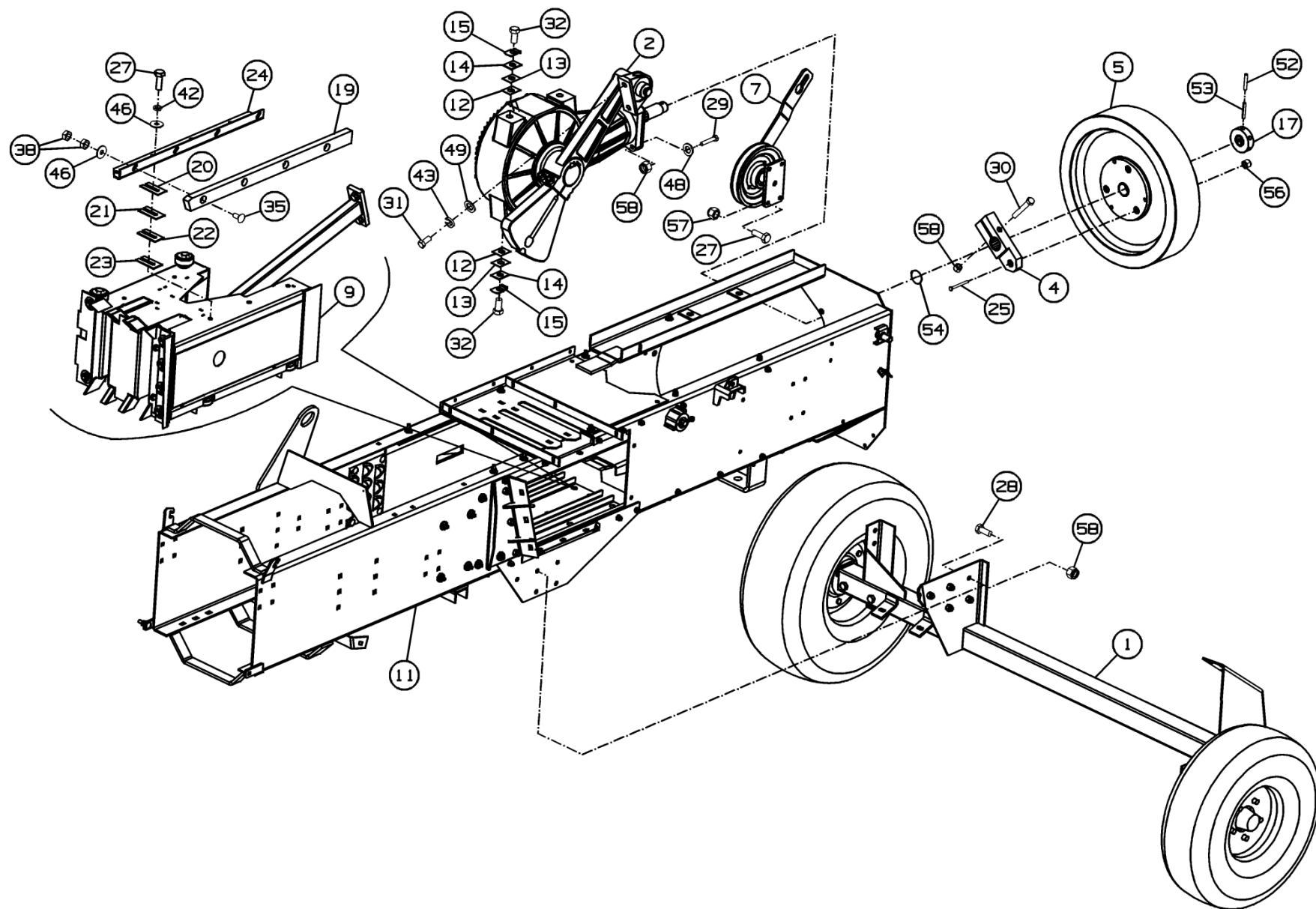
Рисунок 36 – Камера прессующая ППТ-041.12.000
