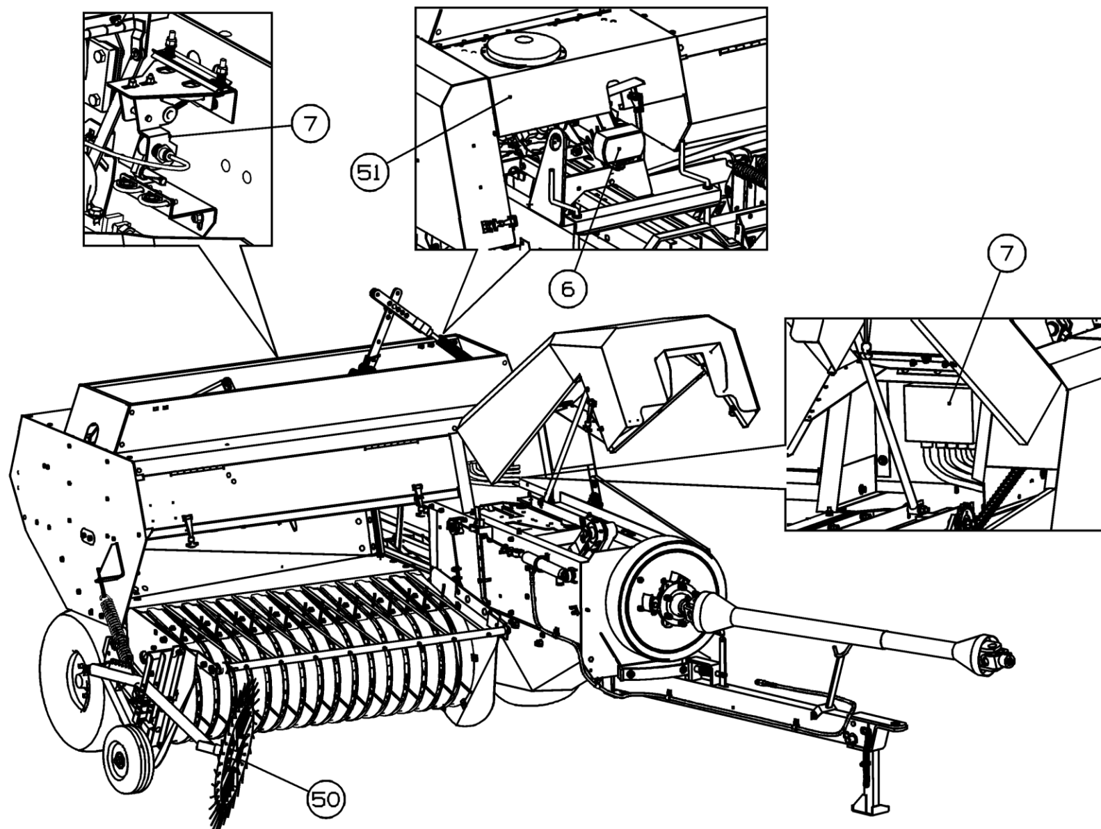
Рисунок 3 - Пресс-подборщик тюковый ПРТ-041.00.000-04 «Tukan Luxe»
