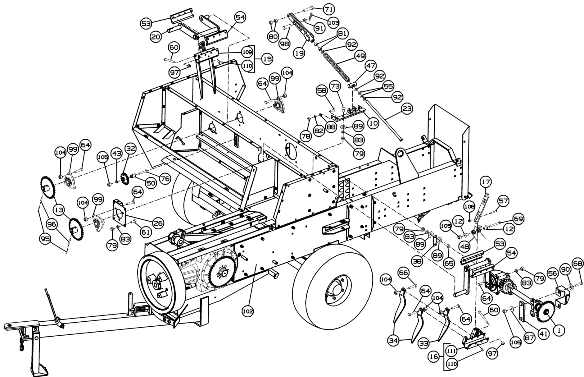
Рисунок 20 – Агрегат прессующий ППТ-041.01.000-01
