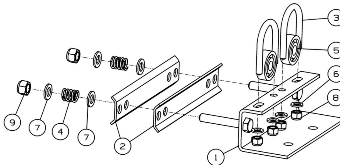
Рисунок 31 - Механизм натяжения шпагата ППТ-041.01.450
