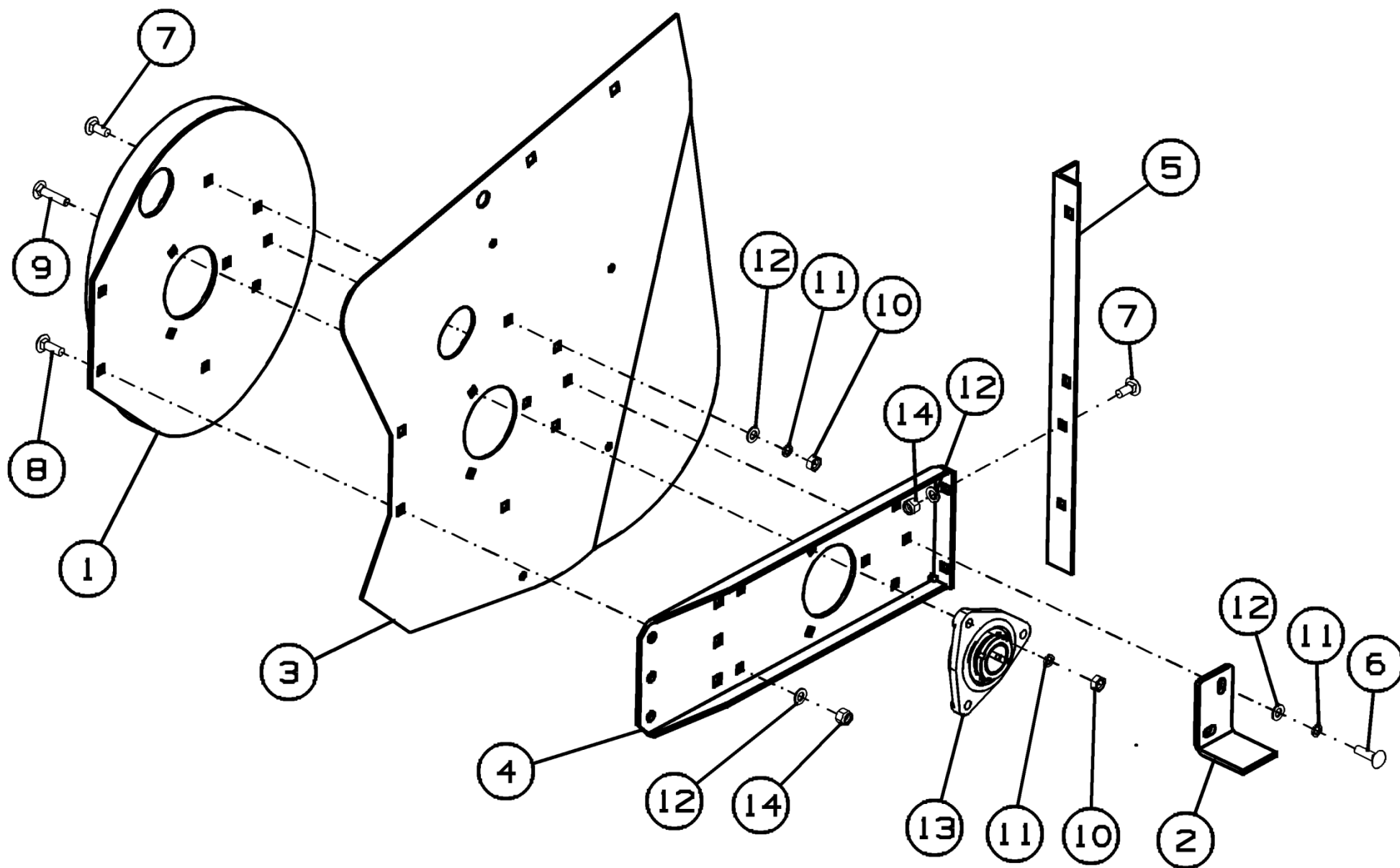
Рисунок 5 – Боковина правая ППТ-041.16.060
