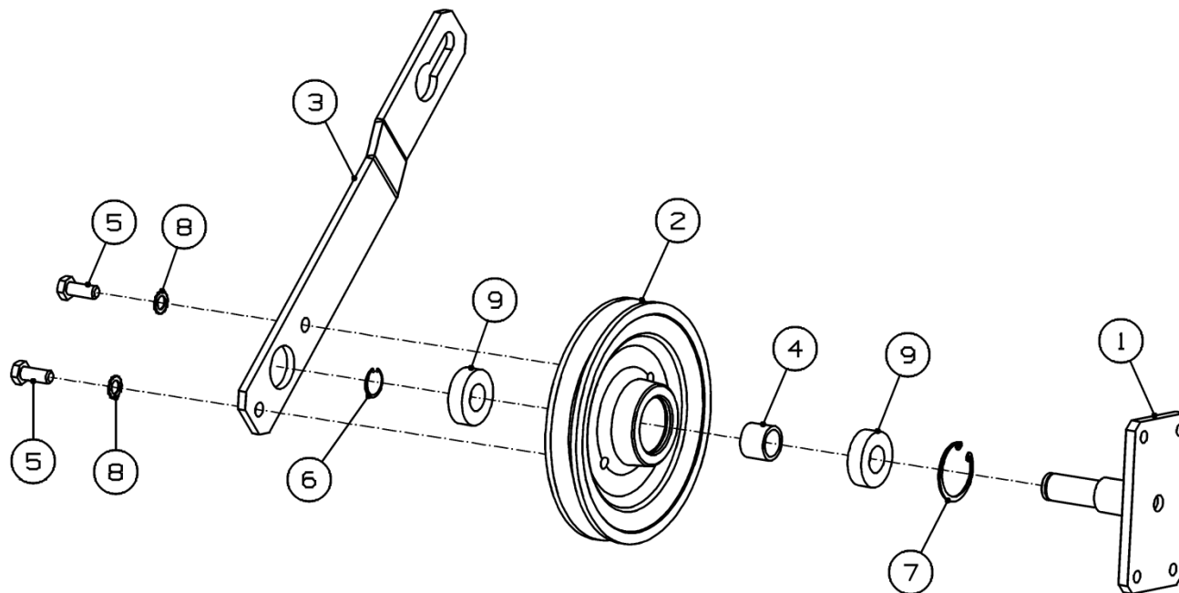
Рисунок 41 - Шкив ведущий ППТ-041.02.400
