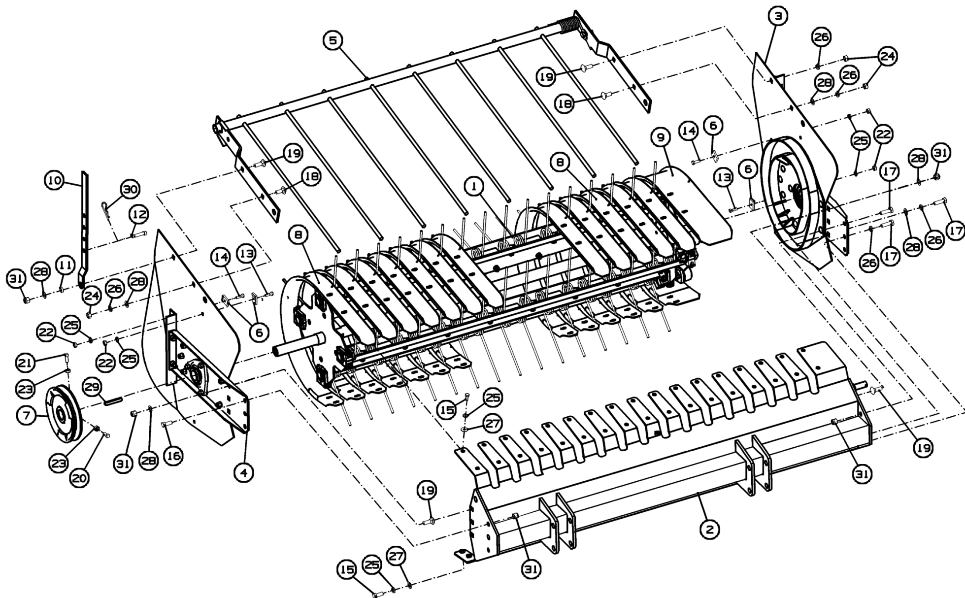
Рисунок 4 – Подборщик ППТ-041.16.000
