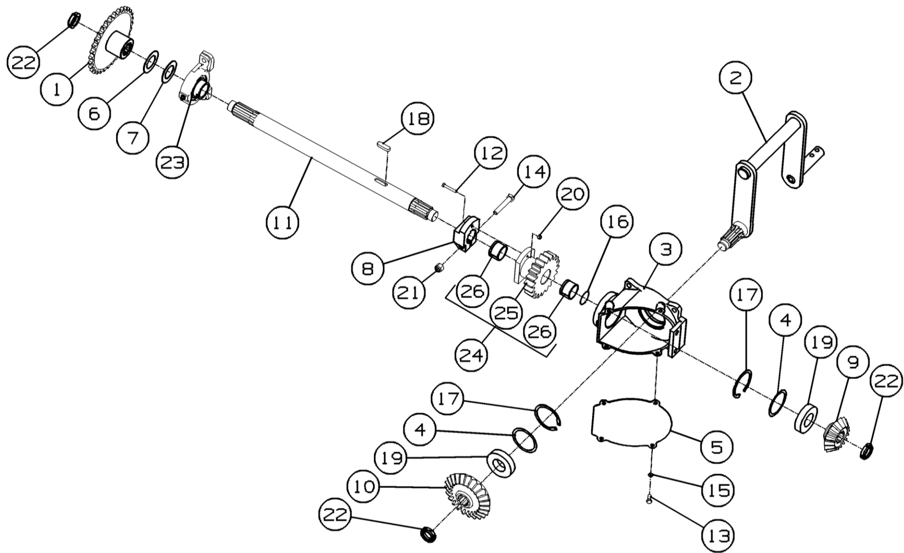
Рисунок 30 - Вал приводной ППТ-041.01.100А
