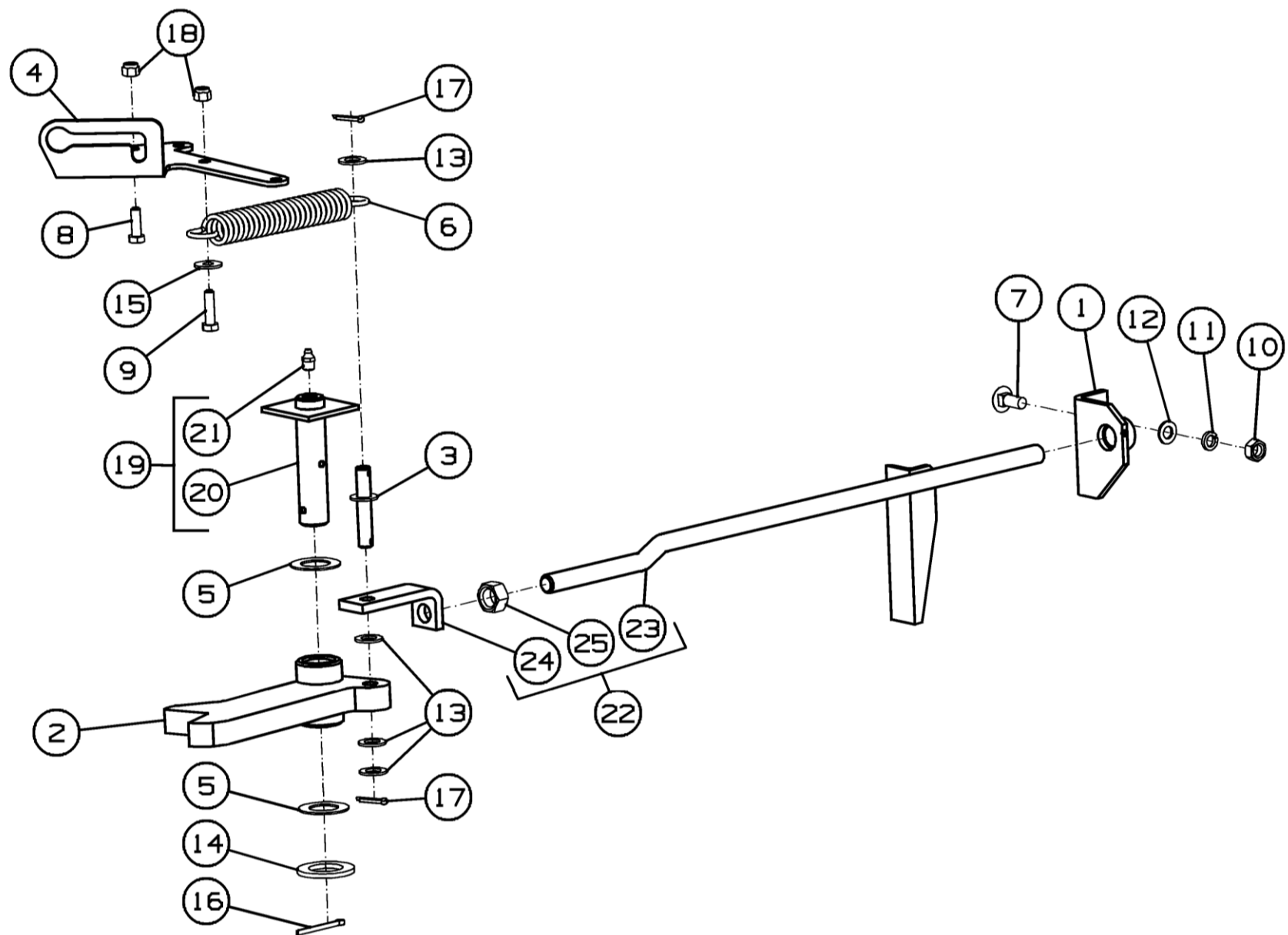
Рисунок 28 - Установка предохранителя ППТ-041.01.300
