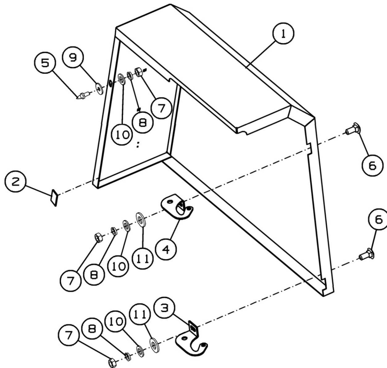
Рисунок 17 – Щиток ППТ-041.10.510
