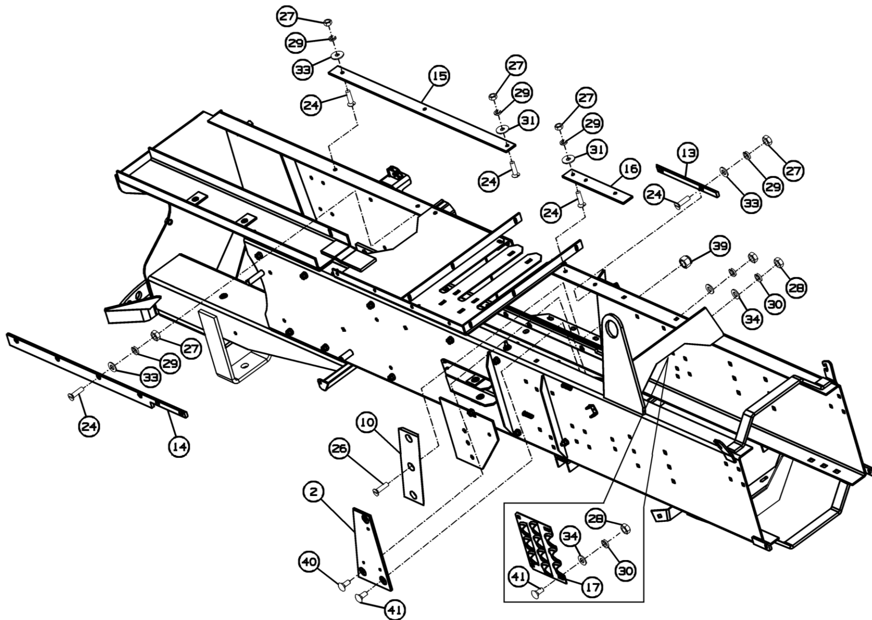
Рисунок 44 - Камера прессующая ППТ-041.14.000
