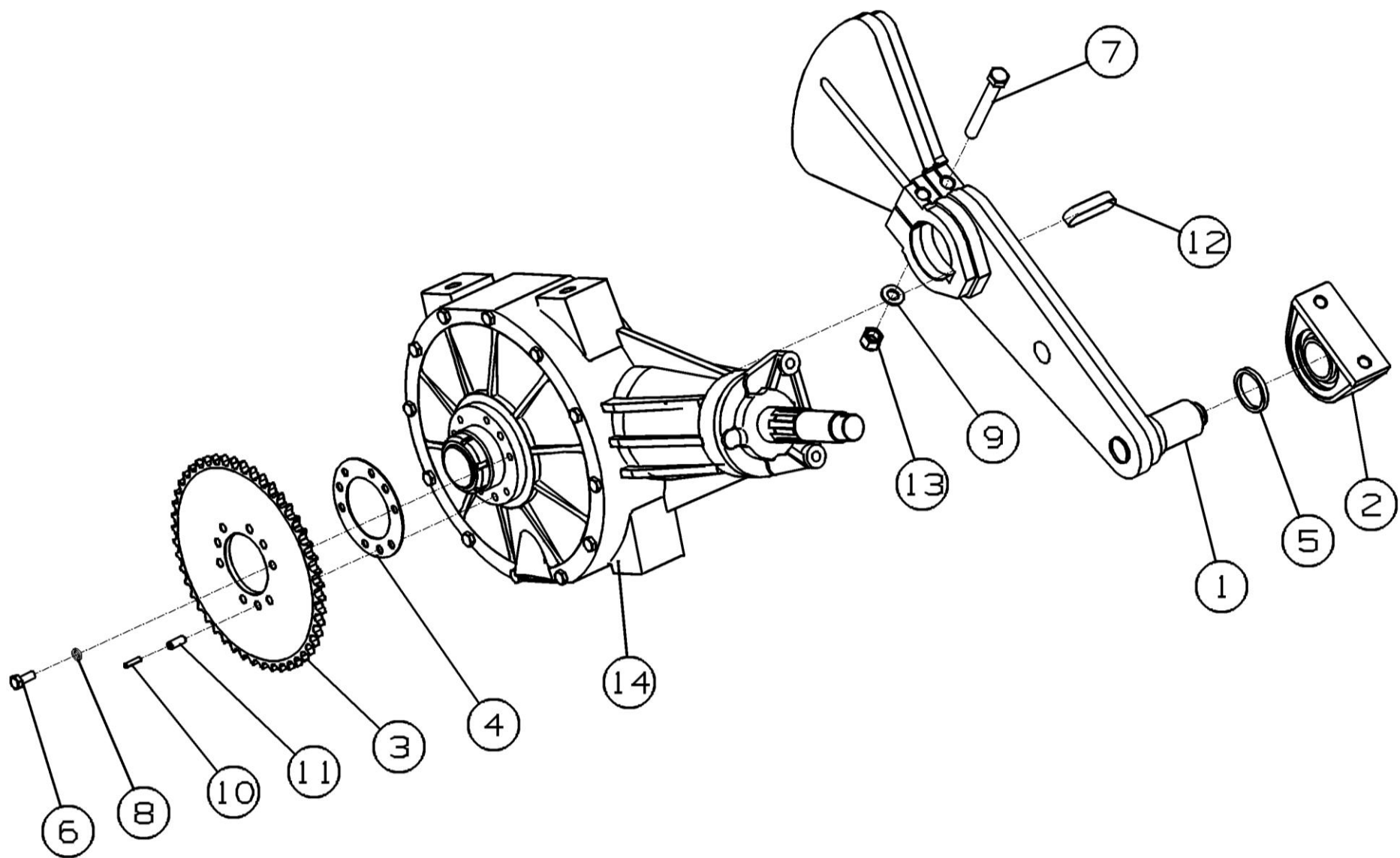
Рисунок 37 - Редуктор ППТ-041.02.530
