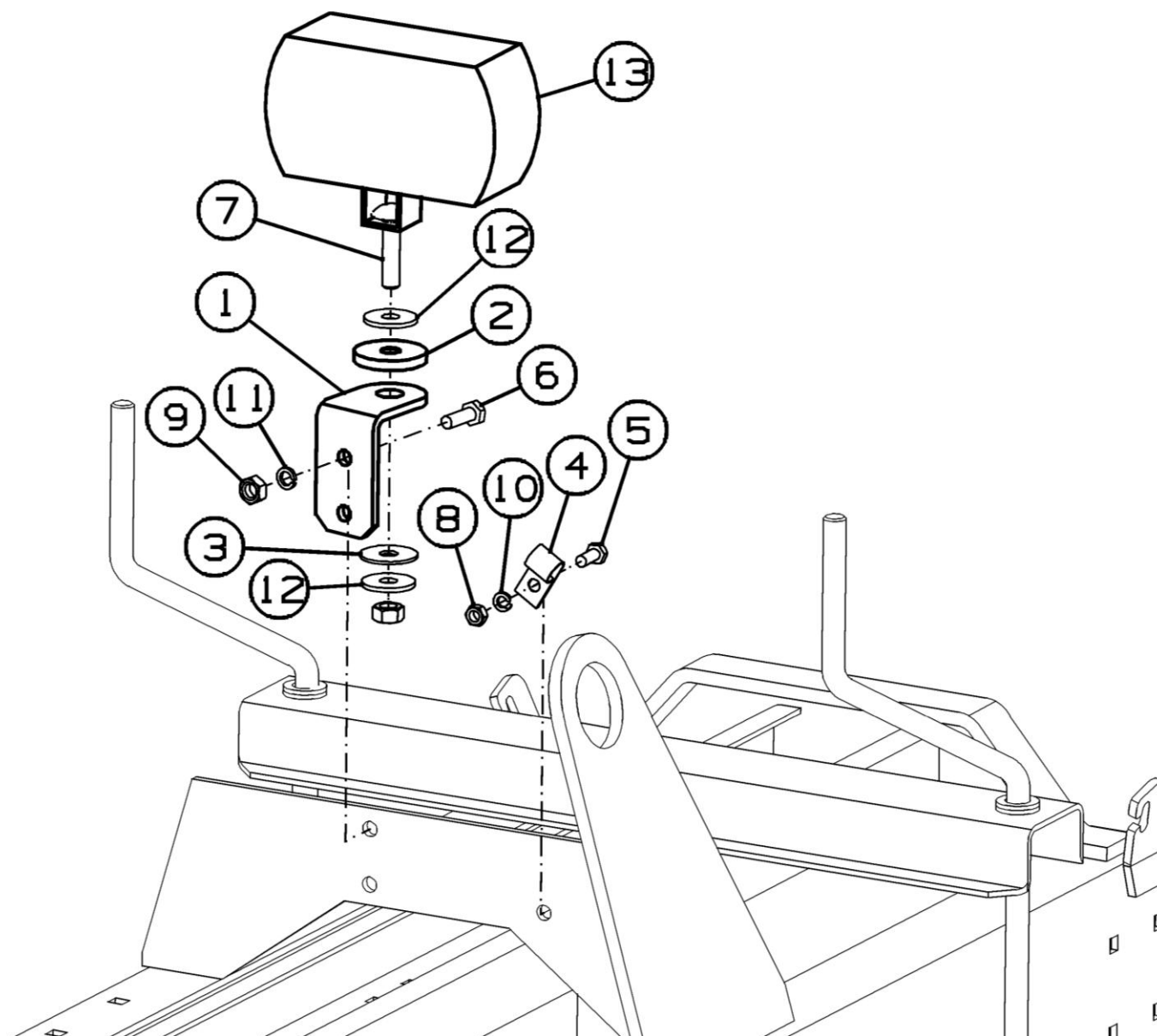
Рисунок 49 - Установка фонаря ППТ-041.00.250 «Tukan Luxe»
