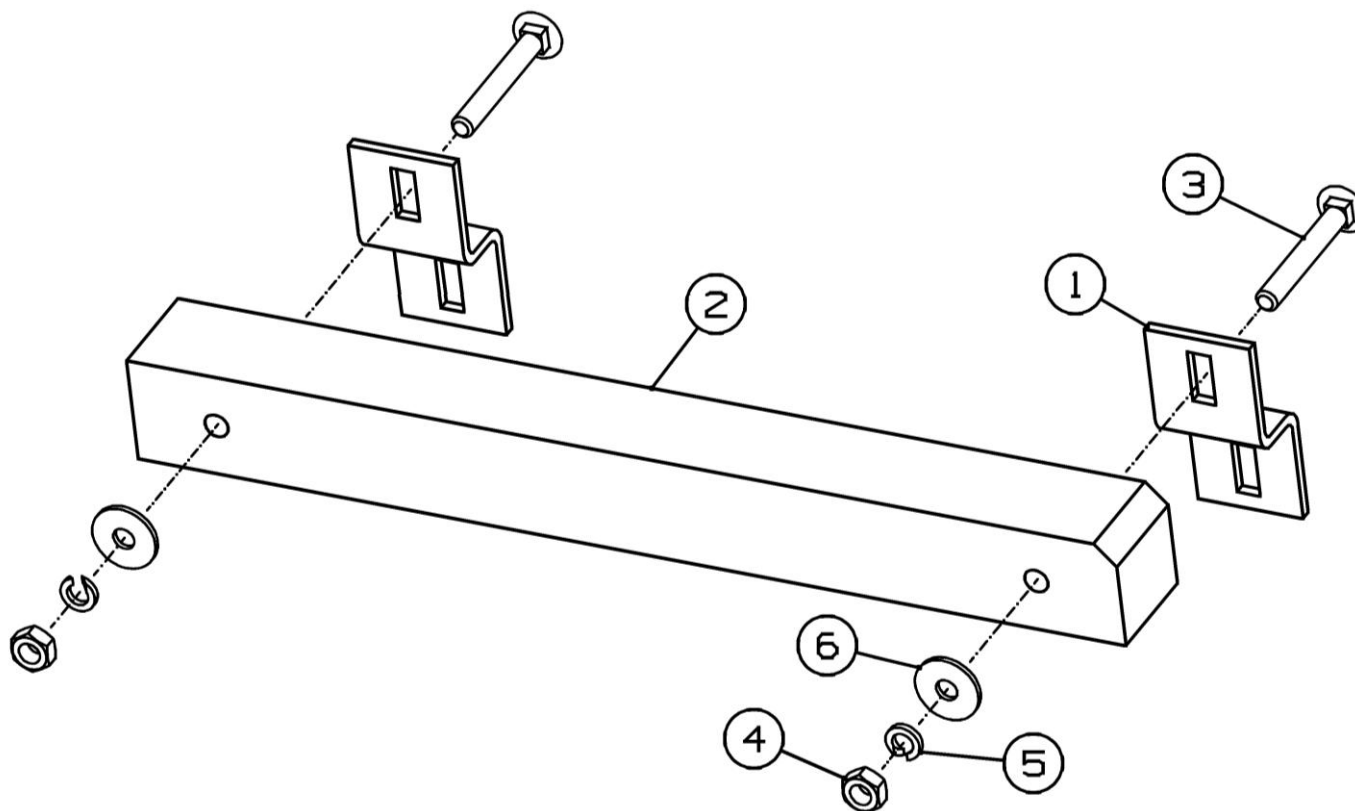
Рисунок 22 – Успокоитель ППТ-041.01.900
