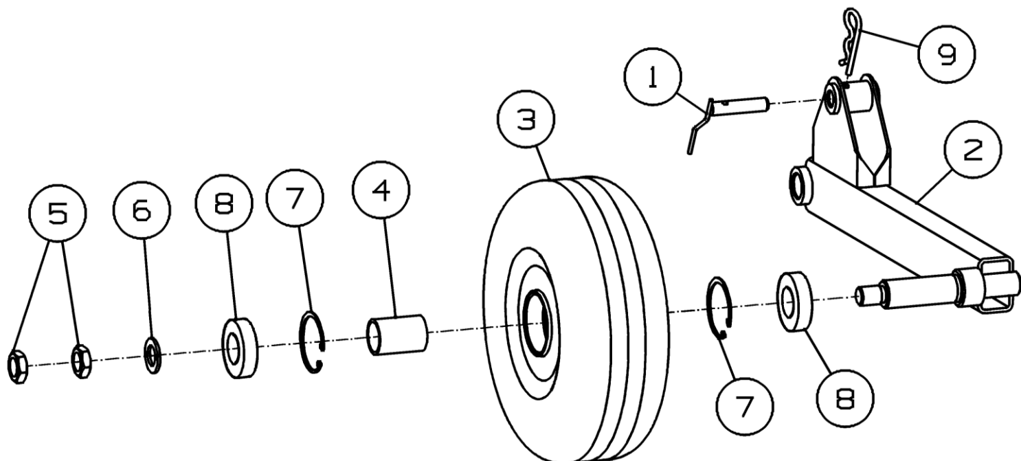
Рисунок 47 - Колесо ППР-122.06.100А
