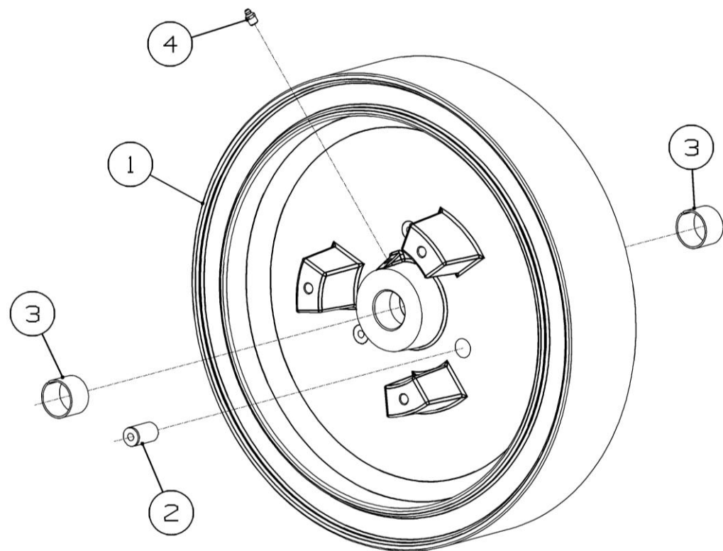
Рисунок 40 – Маховик ППТ-041.02.360
