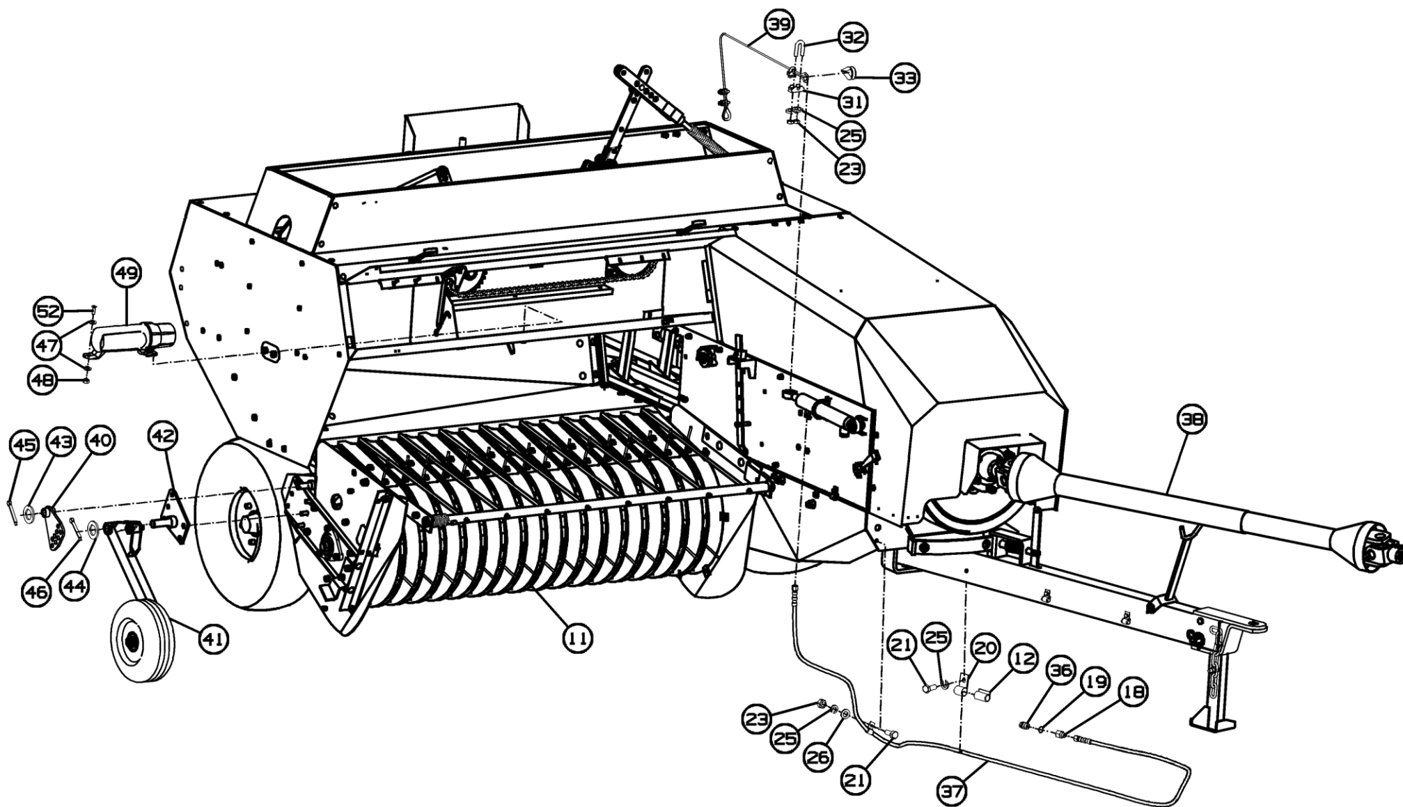
Рисунок 1 - Пресс-подборщик тюковый ППТ-041.00.000 «Тукап»
