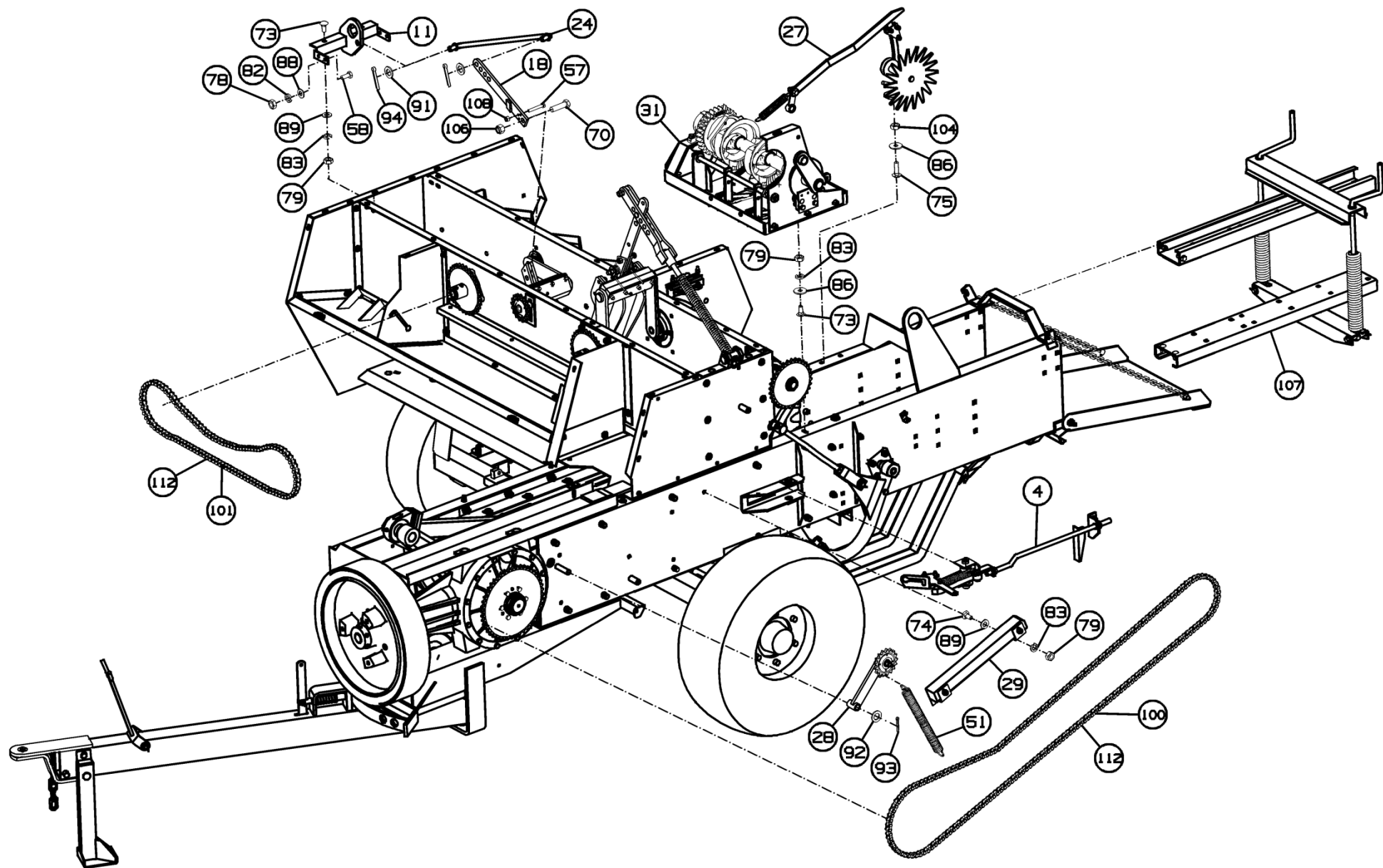
Рисунок 18 – Агрегат прессующий ППТ-041.01.000-01
