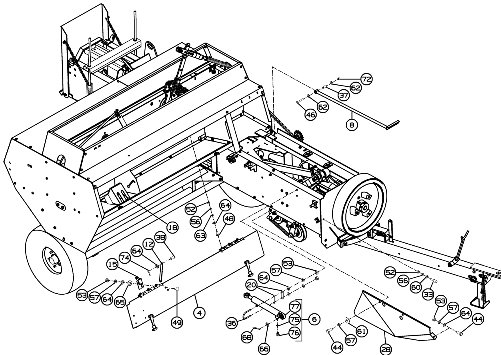
Рисунок 10 – Пресс ППТ-041.10.000-01
