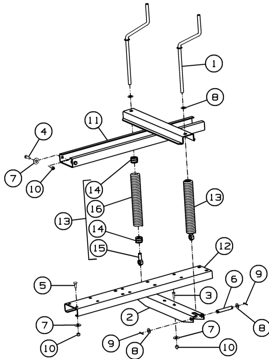
Рисунок 23 - Механизм увеличения плотности прессования ППТ-041.01.700-01
