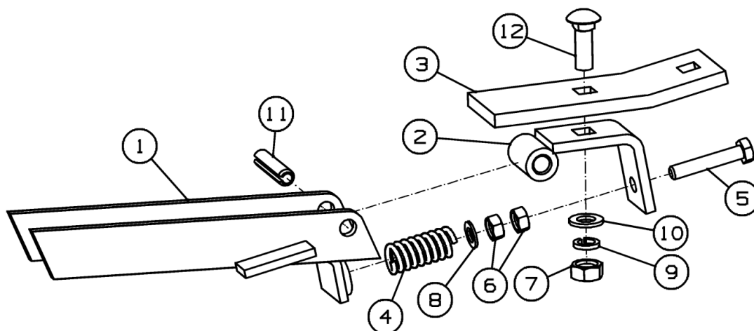
Рисунок 46 - Упор ППТ-041.04.180
