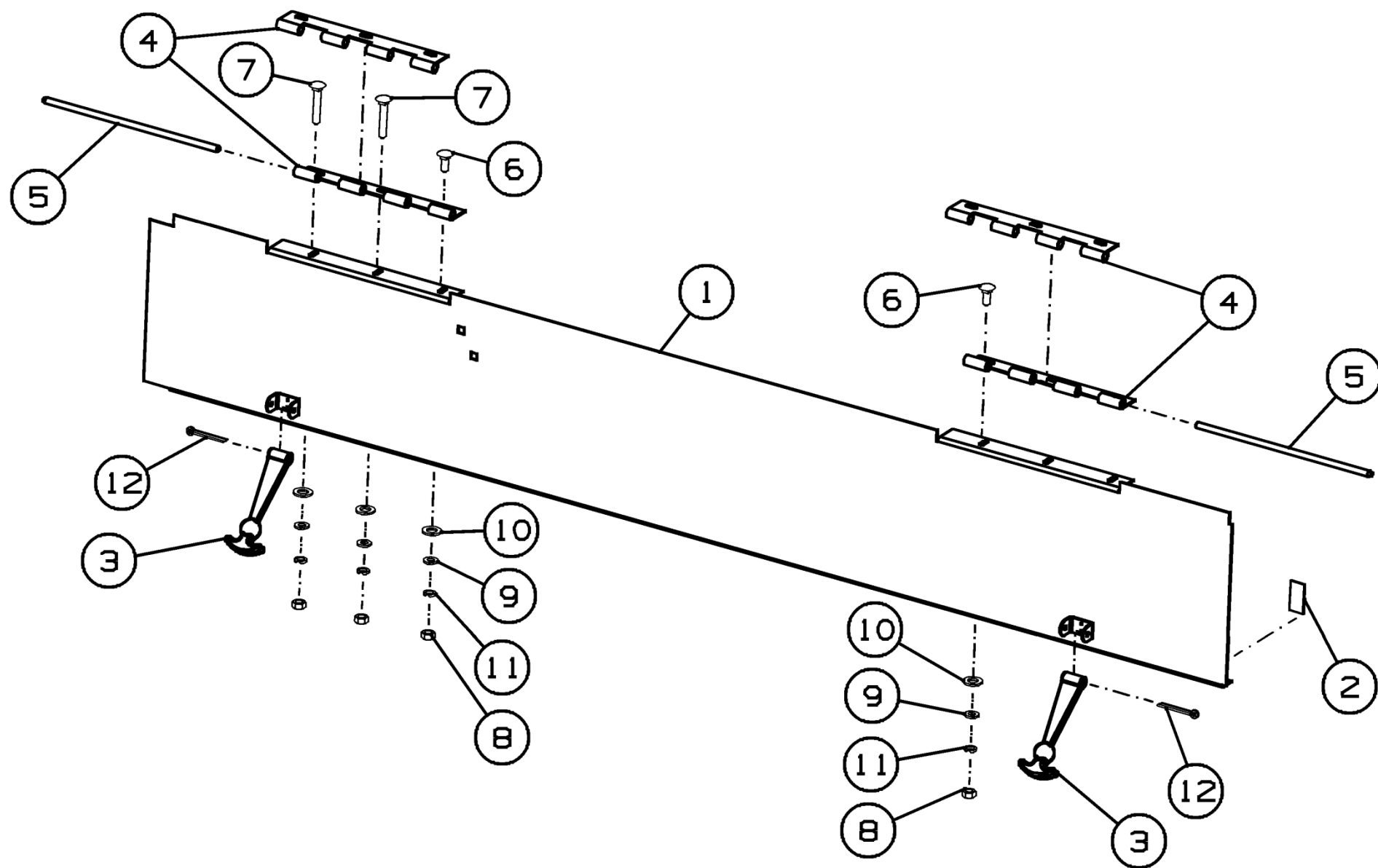
Рисунок 14 – Крышка ППТ-041.10.130
