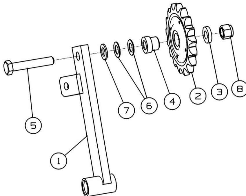
Рисунок 29 – Натяжник ППТ-041.01.880
