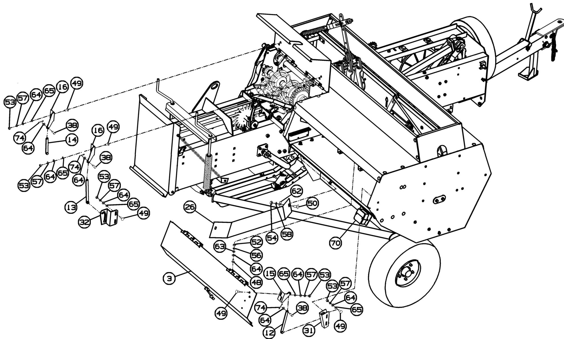
Рисунок 11 – Пресс ППТ-041.10.000-01
