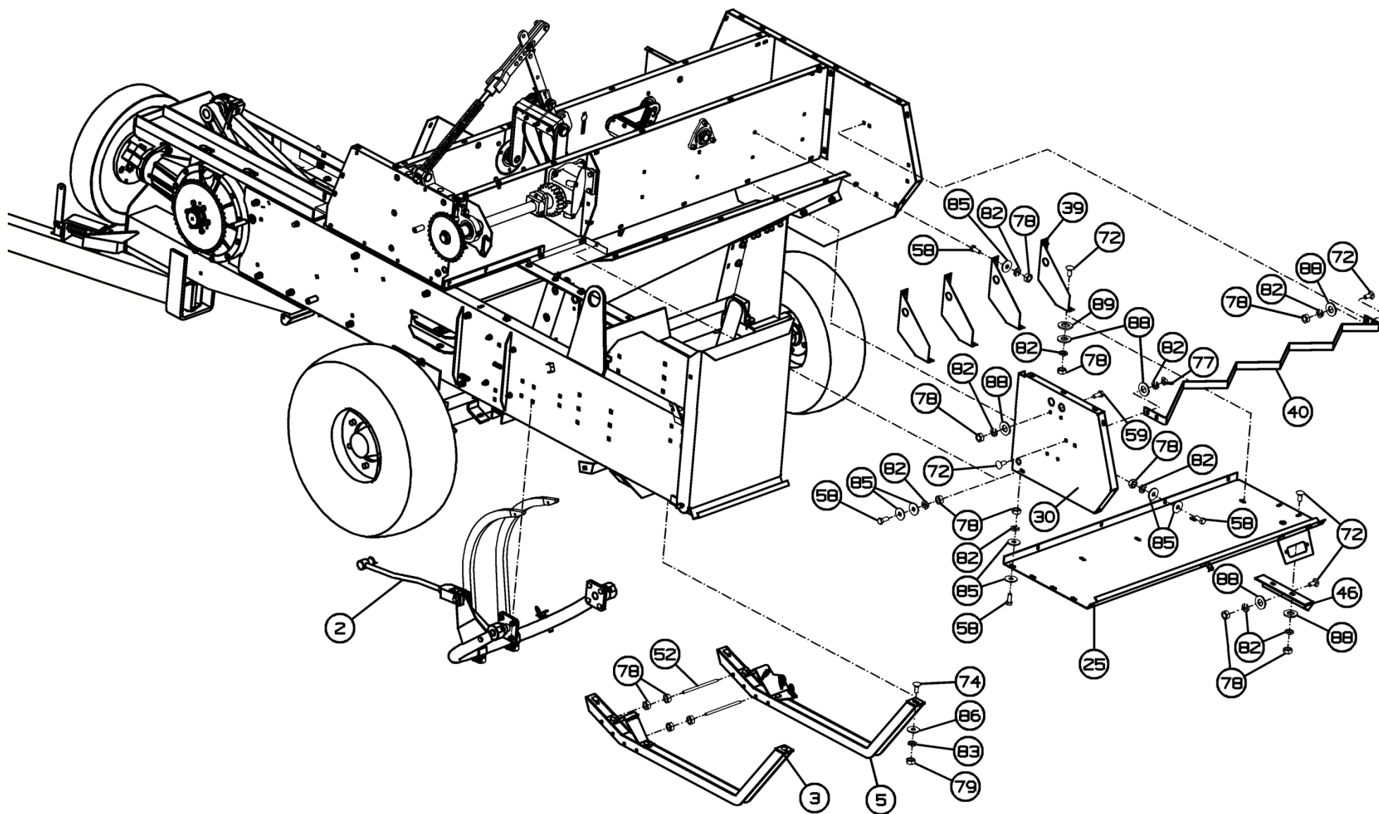
Рисунок 19 – Агрегат прессующий ППТ-041.01.000-01
