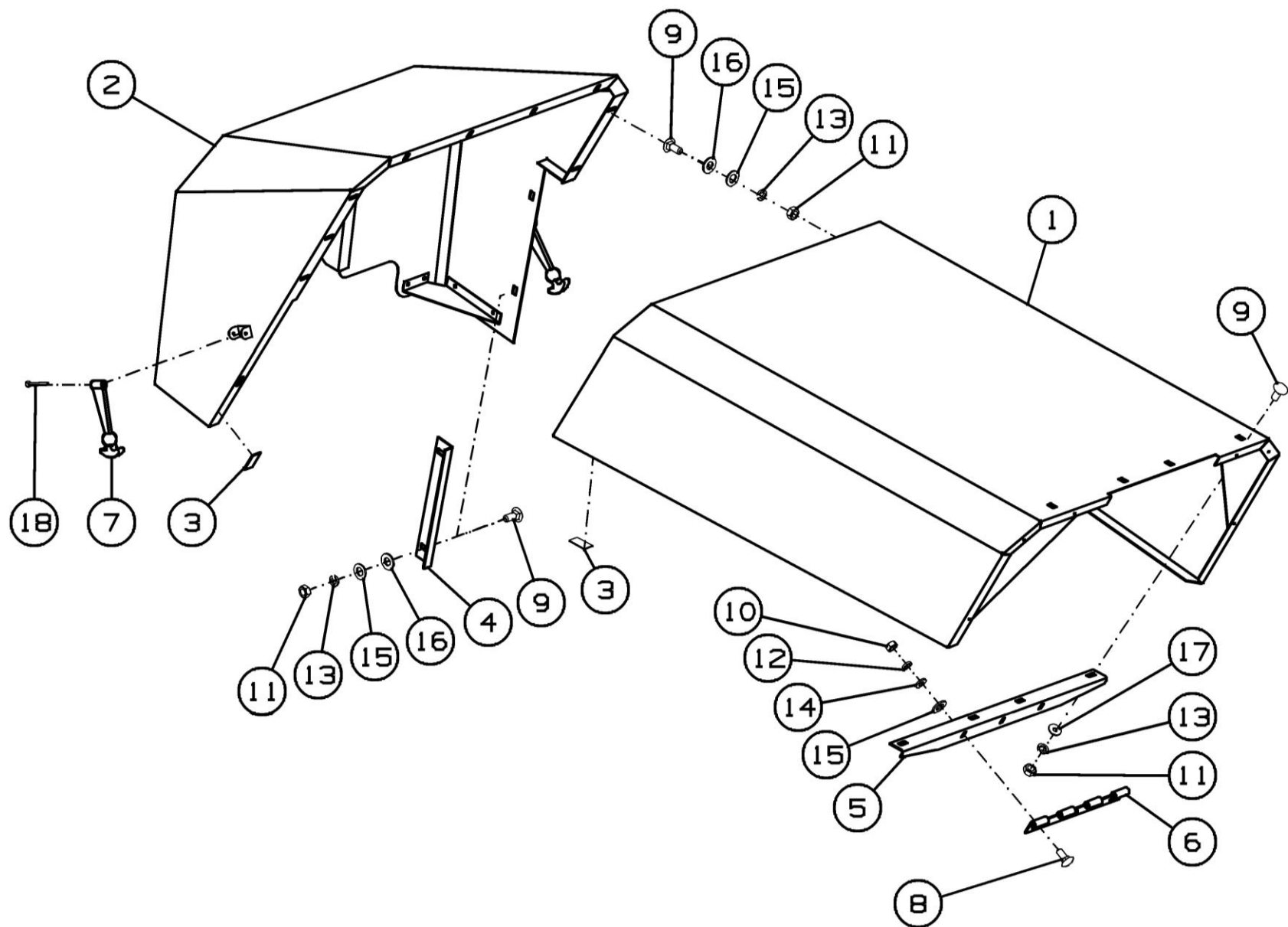
Рисунок 16 – Щит ППТ-041.10.400
