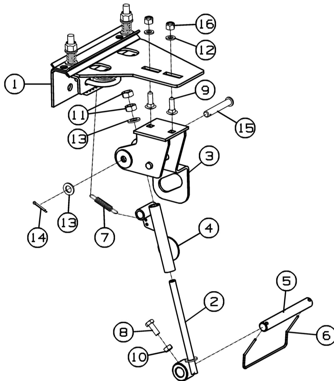
Рисунок 51 - Датчик обрыва шпагата ППТ-041.01.020 «Tukan Luxe»
