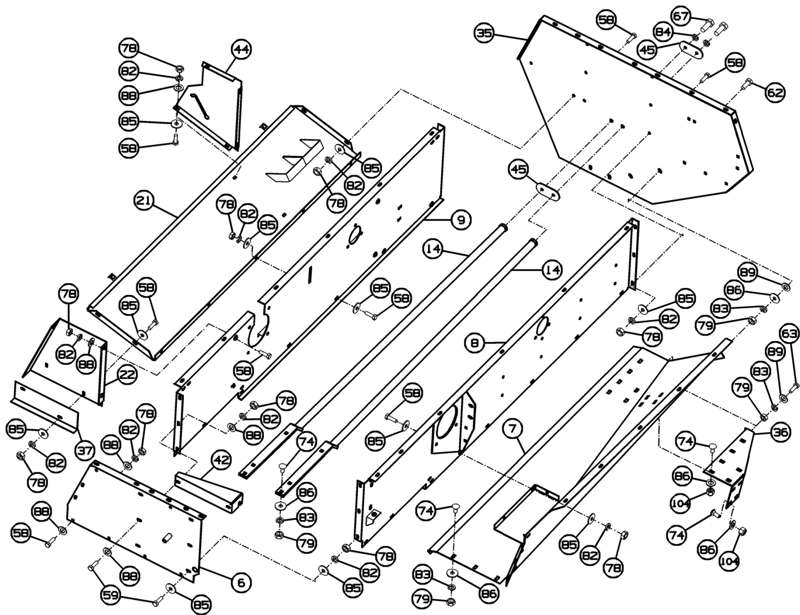
Рисунок 21 – Агрегат прессующий ППТ-041.01.000-01
