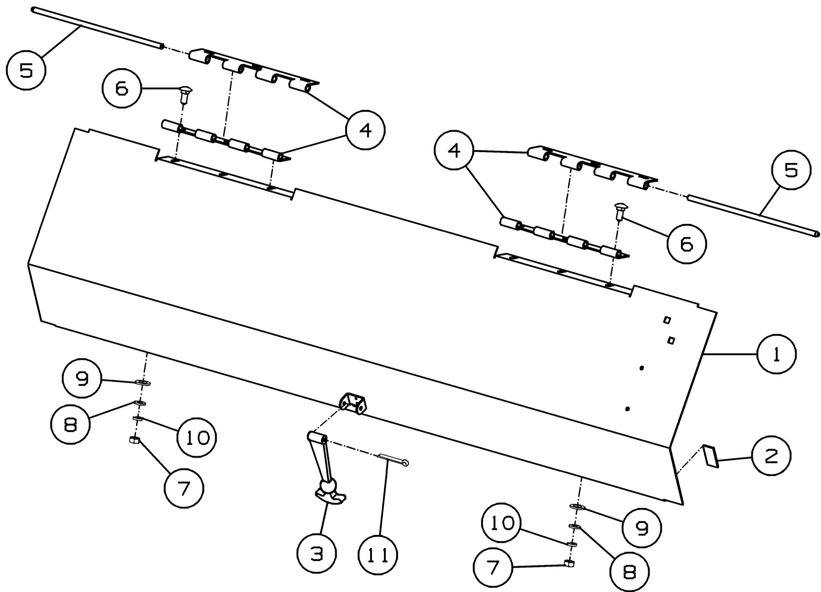
Рисунок 13 – Крышка ППТ-041.10.110
