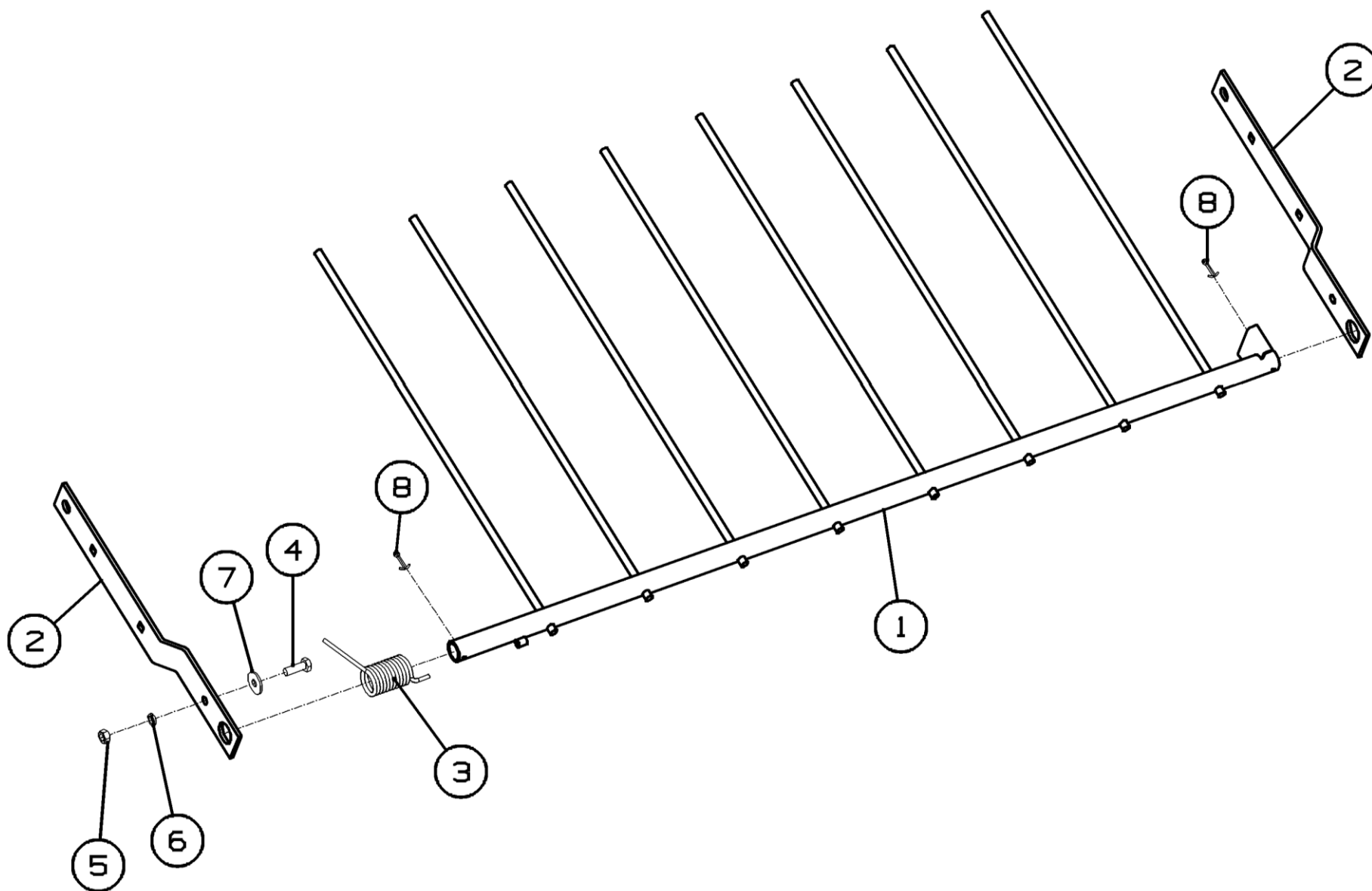
Рисунок 7 – Нормализатор ППТ-041.06.090
