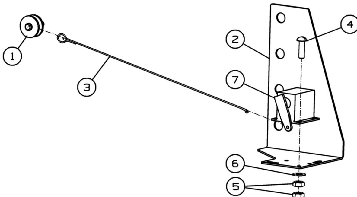
Рисунок 48 - Счетчик тьюков ППТ-041.00.130
