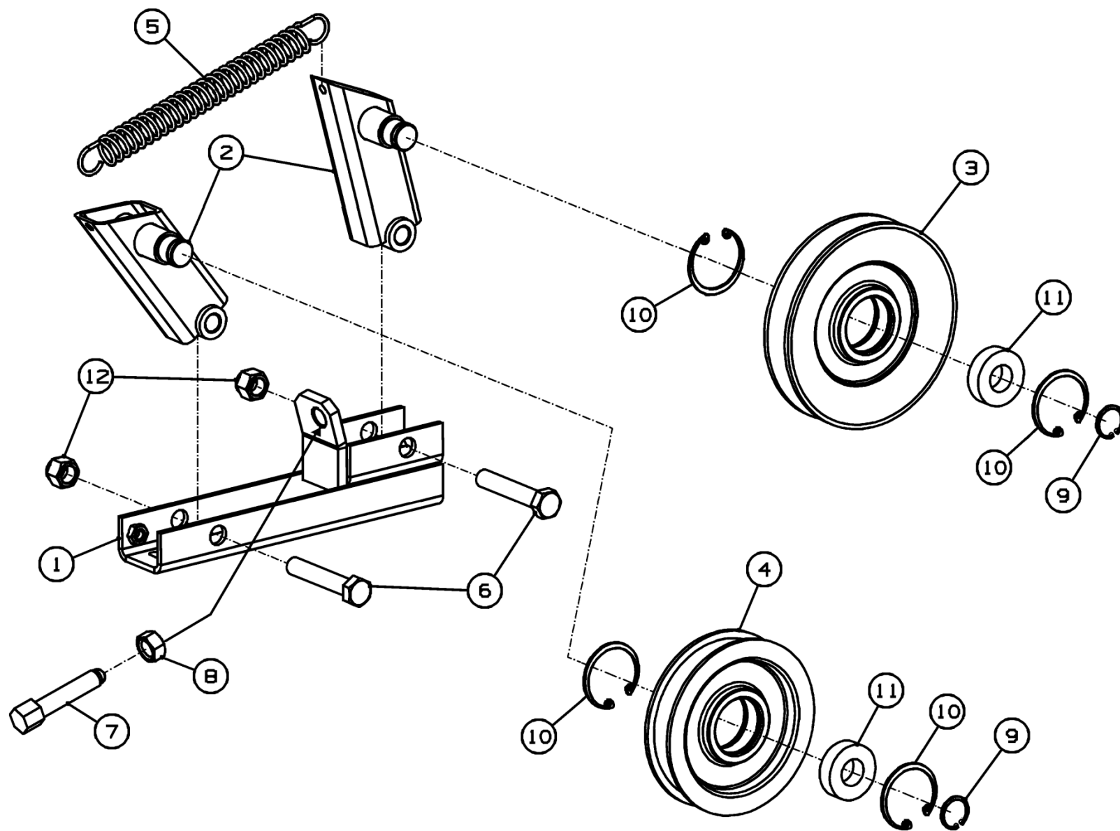
Рисунок 42 - Шкив обводной ППТ-041.02.440
