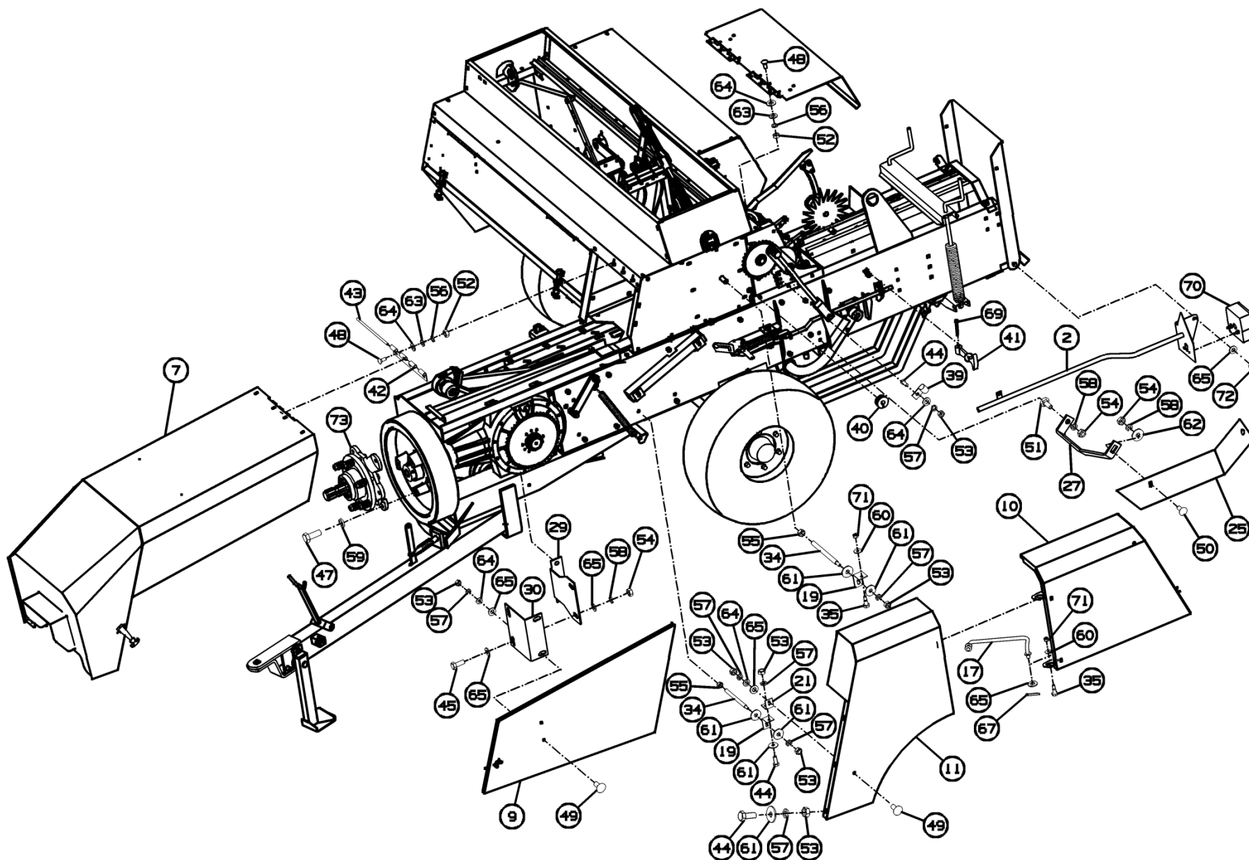
Рисунок 9 – Пресс ППТ-041.10.000-01
