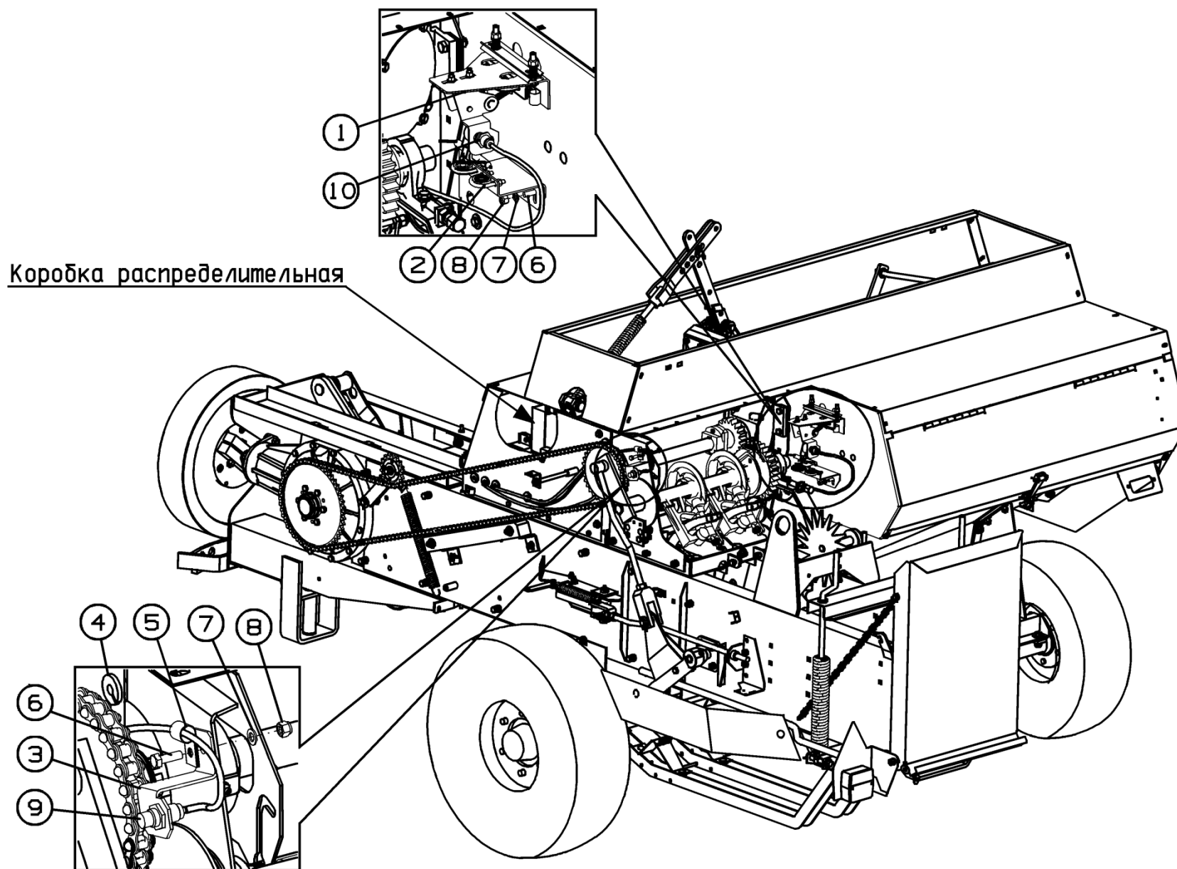
Рисунок 50 - Установка пульта с датчиками ППТ-041.01.010 «Tukan Luxe»
