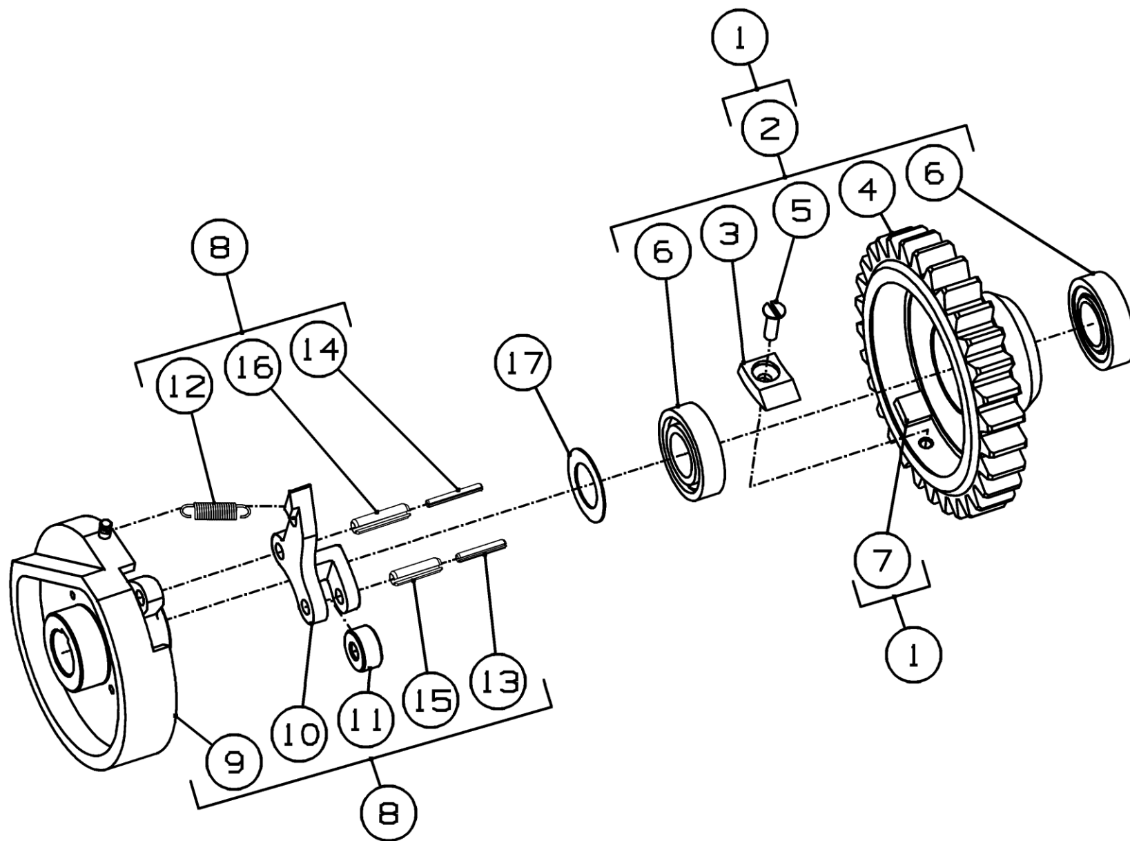
Рисунок 34 – Полумуфта ППТ-041.07.250, Полумуфта ППТ-041.07.270А
