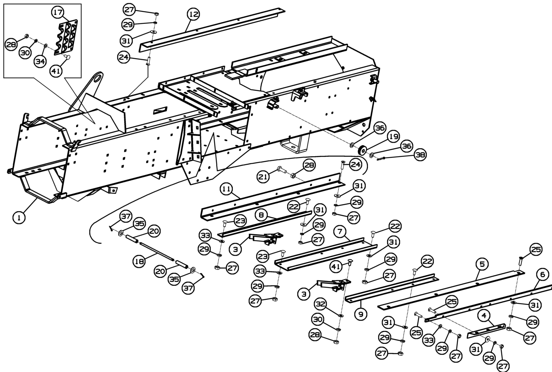
Рисунок 45 - Камера прессующая ППТ-041.14.000
