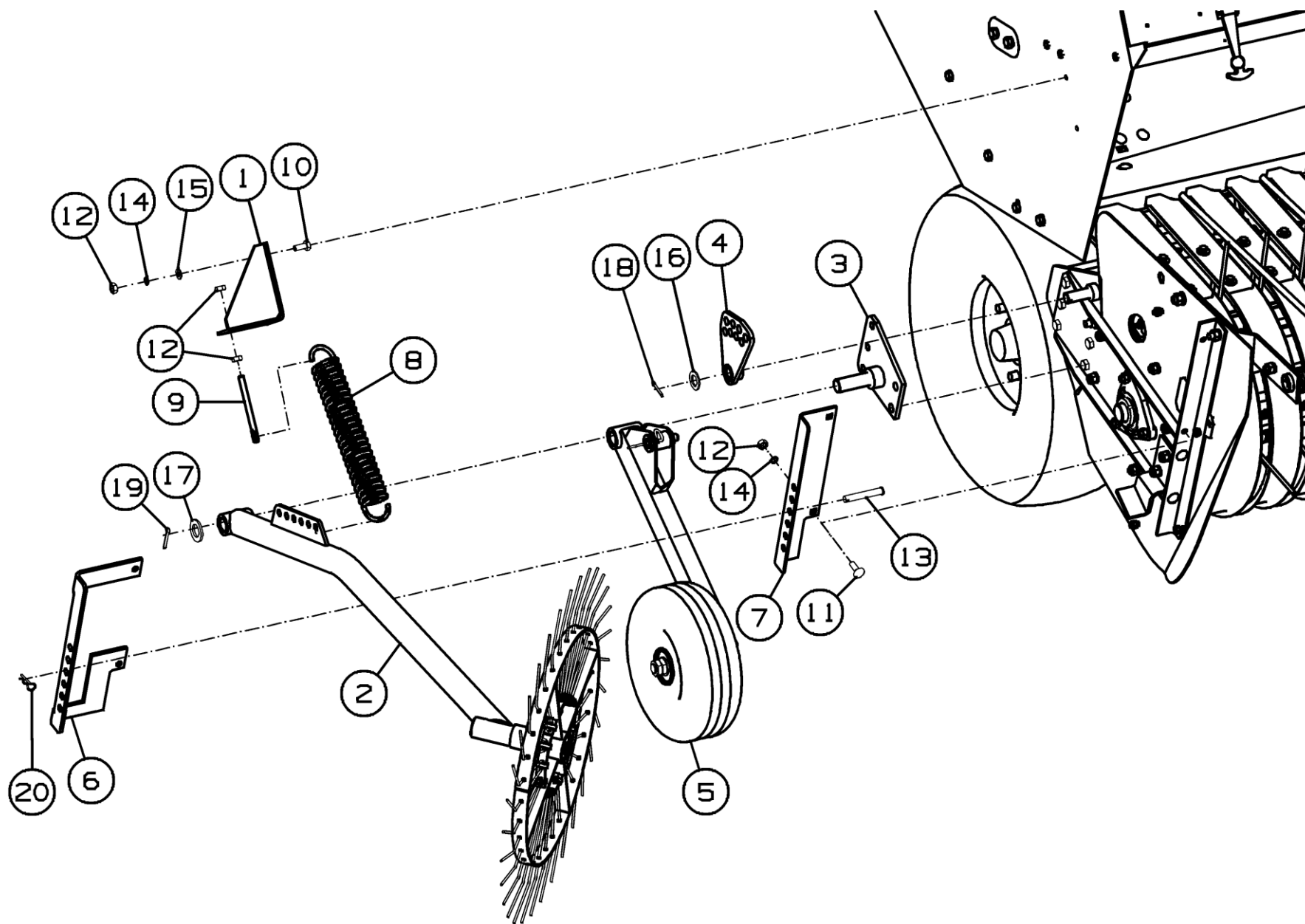
Рисунок 54 - Схема установки копирующего колеса и колеса пальцевого ППТ-041.00.190 «Tukan Luxe»
