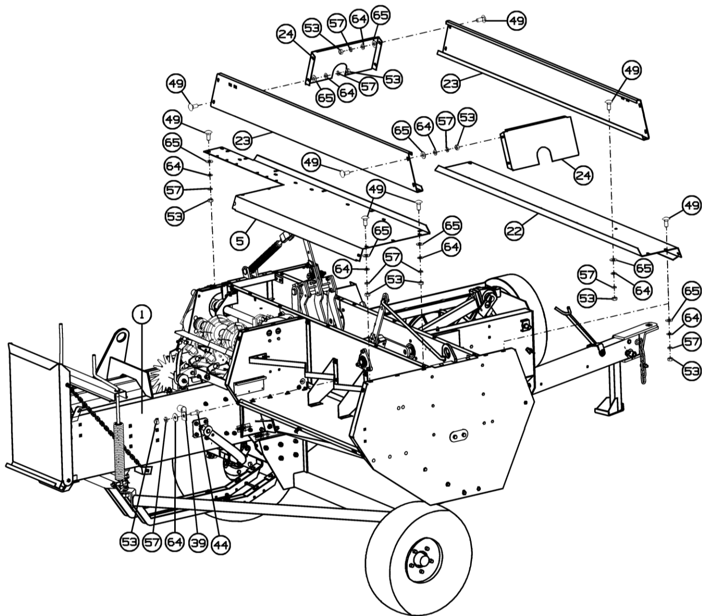
Рисунок 12 – Пресс ППТ-041.10.000-01
