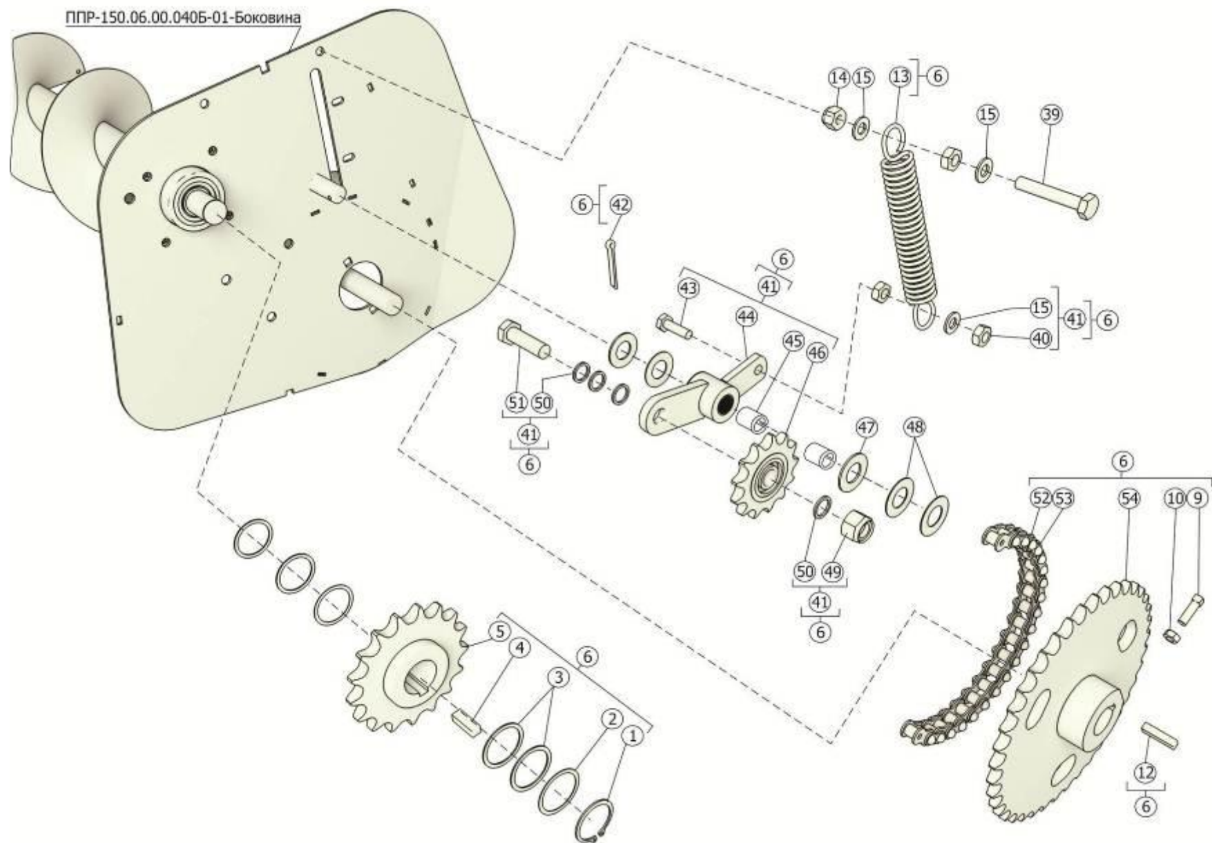
Рисунок 46- Установка привода ППР-150.06.00.160А
