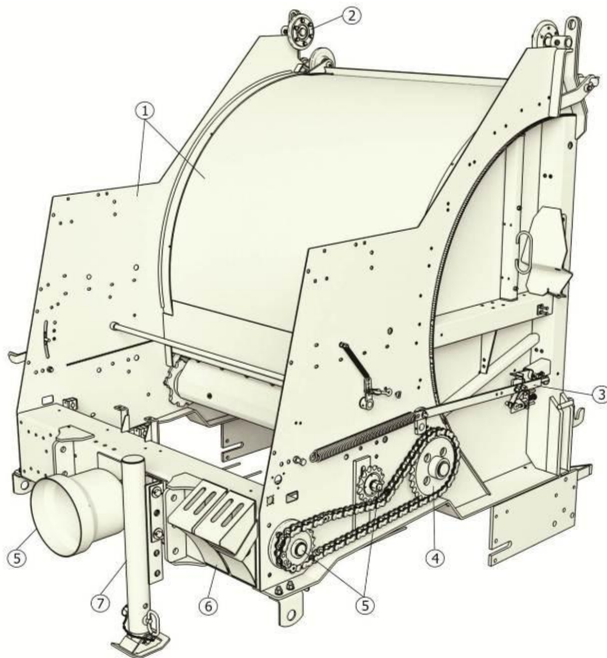
Рисунок 2 – Камера передняя ППР-150.01.00.000А
