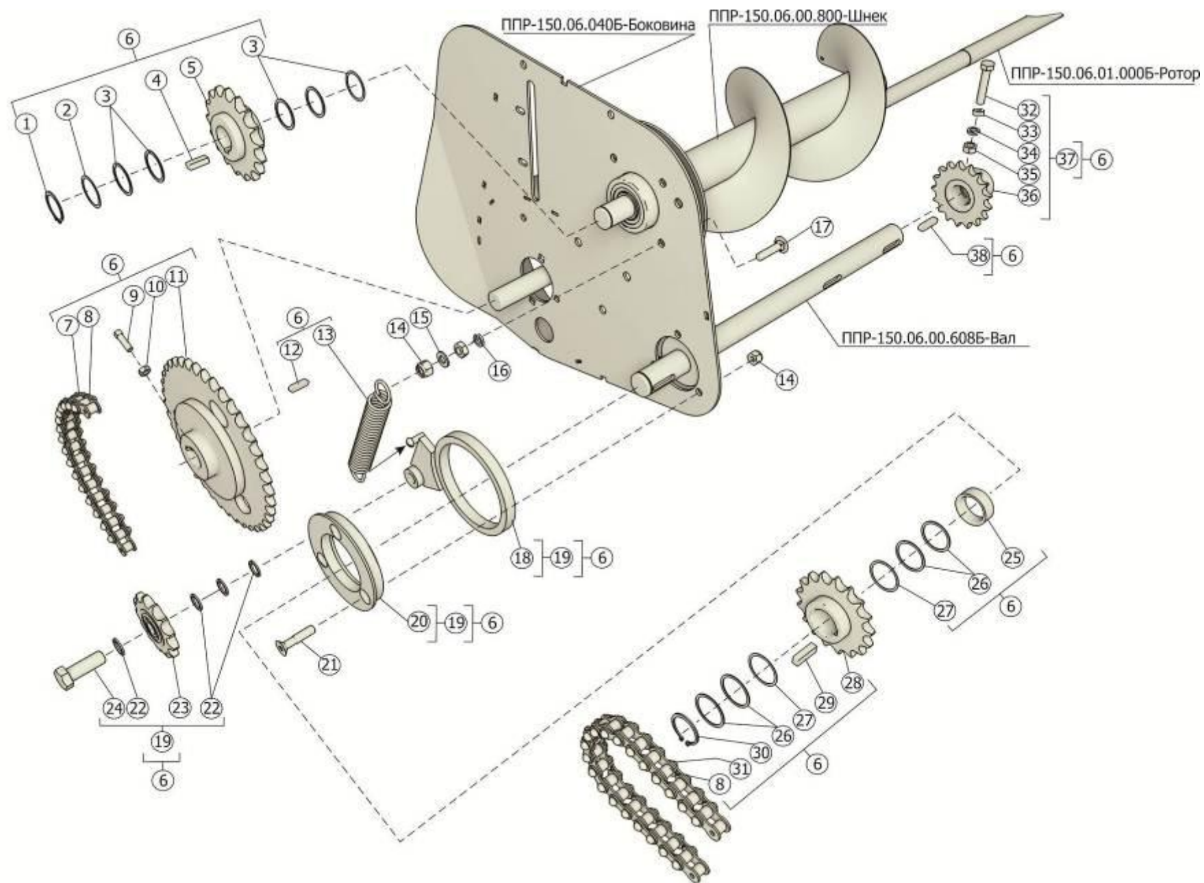
Рисунок 45- Установка привода ППР-150.06.00.160А
