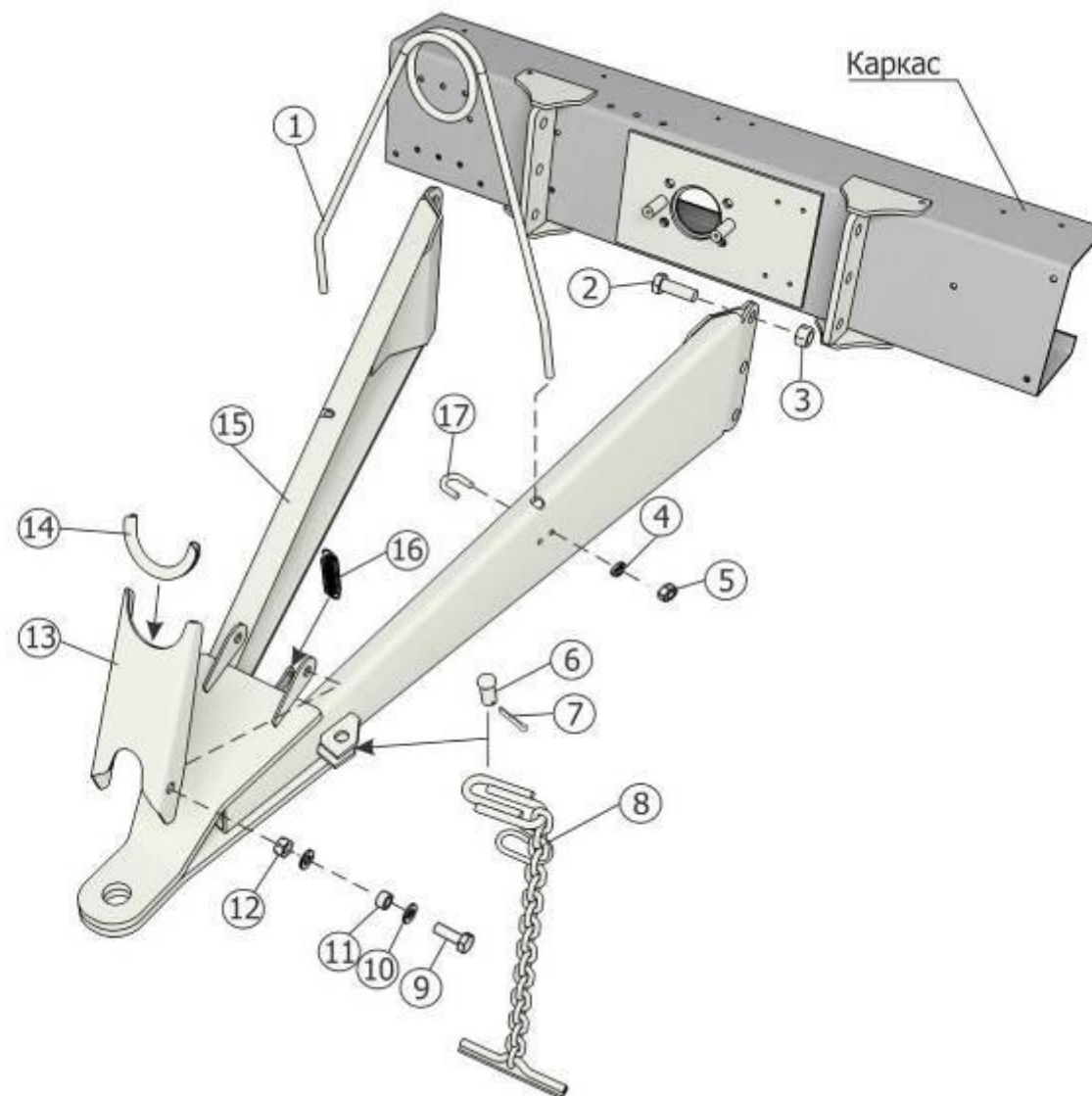
Рисунок 22 – Установка сннца ППР-150.07.00.000А
