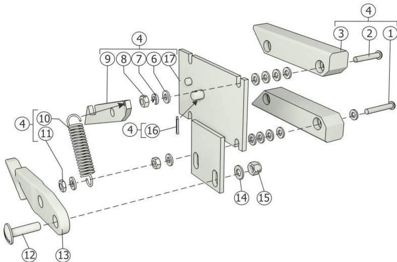
Рисунок 27 – Каретка ППР-150.10.03.000А-01
