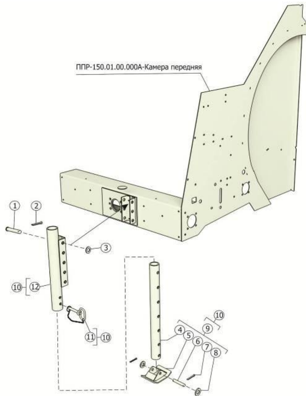
Рисунок 6 – Установка опоры ППР-150.01.00.200
