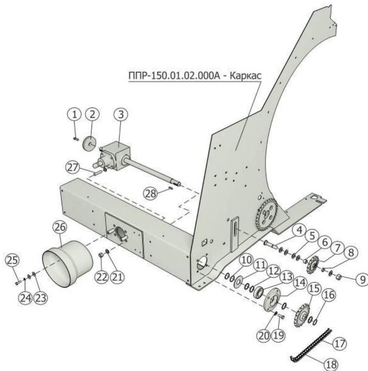
Рисунок 7 – Установка главного привода ППР-150.01.03.000А
