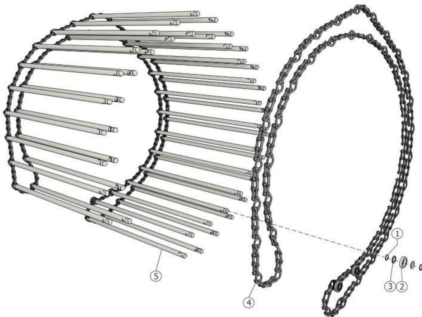
Рисунок 18 – Транспортер цепной ППР-150.03.03.000Б
