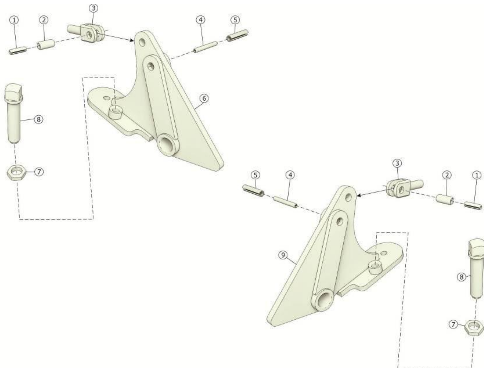
Рисунок 16 – Коромысло ППР-150.03.07.010Б. Коромысло ППР-150.03.07.010Б-01
