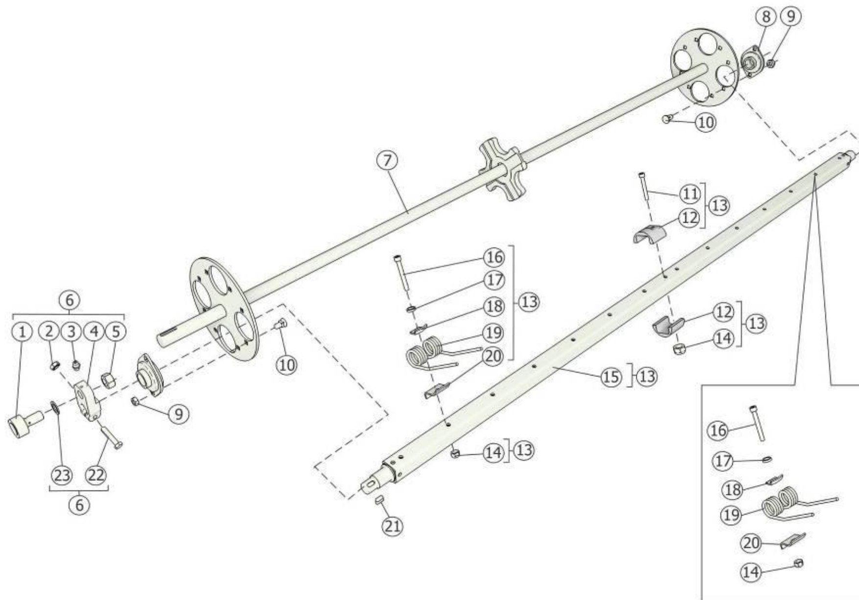
Рисунок 49 – Ротор ППР-150.06.01.000А
