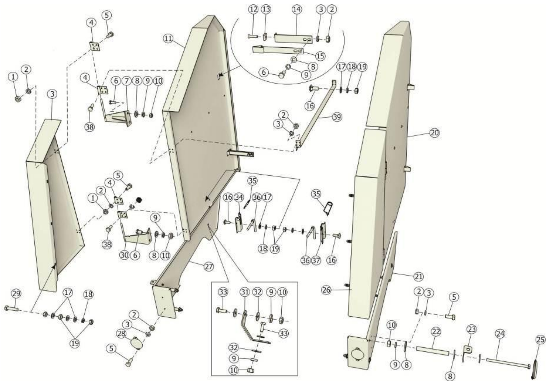
Рисунок 35 – Установка щитков боковых ППР-150.11.01.2005
