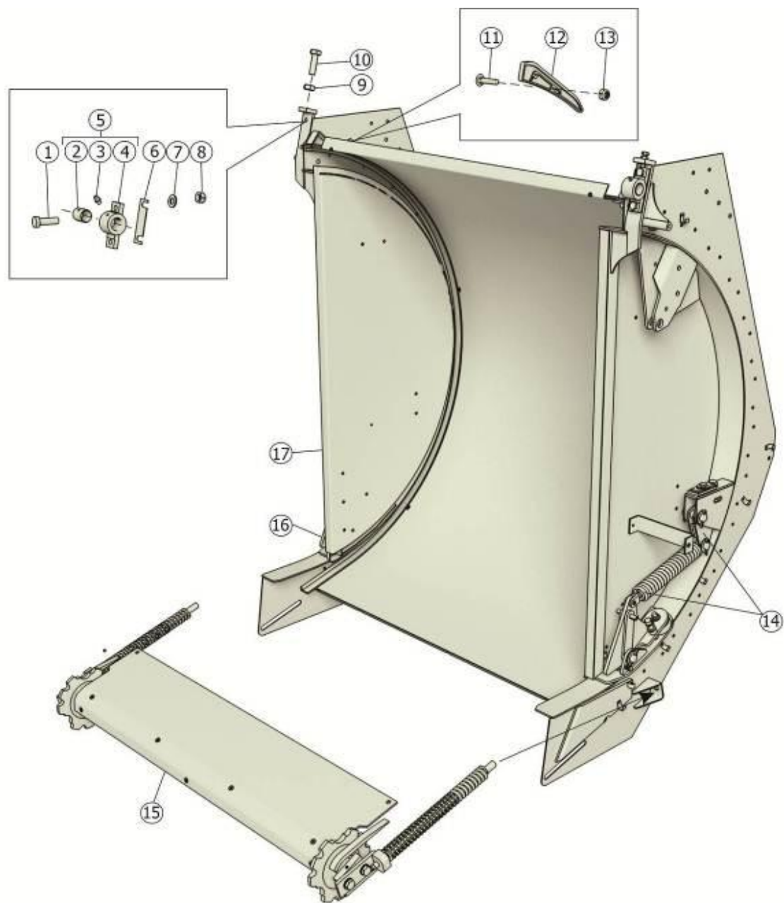
Рисунок 13 - Камера задняя ППР-150.03.00.000А
