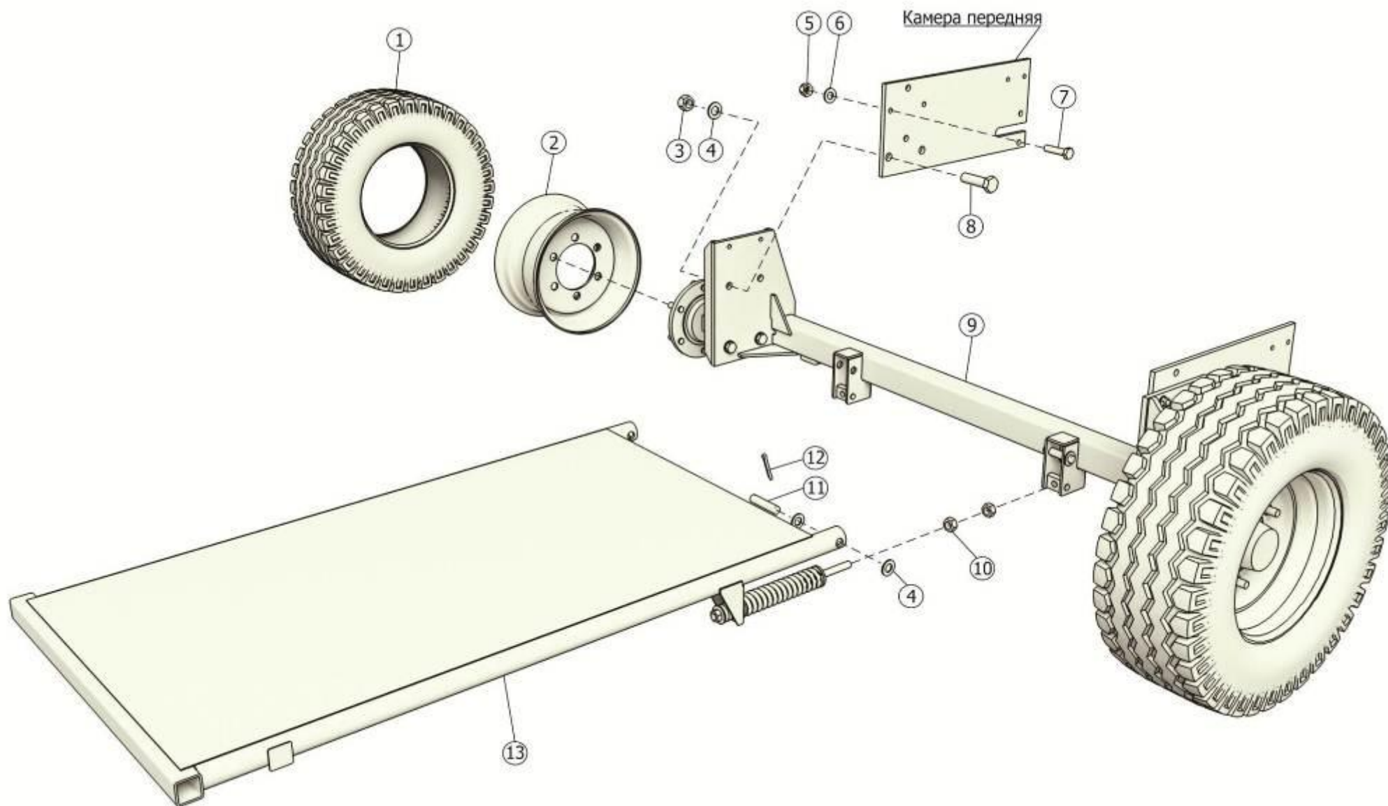
Рисунок 19 – Шасси ППР-150.02.00.000Б
