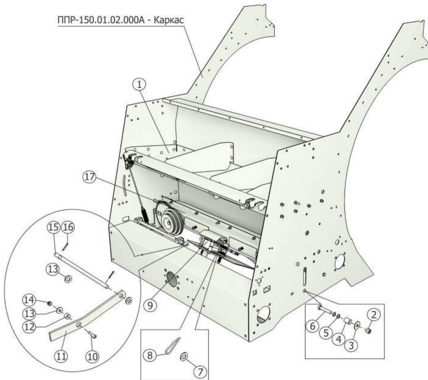
Рисунок 23 - Установка механизма обматывающего ППР-150.10.00.000А
