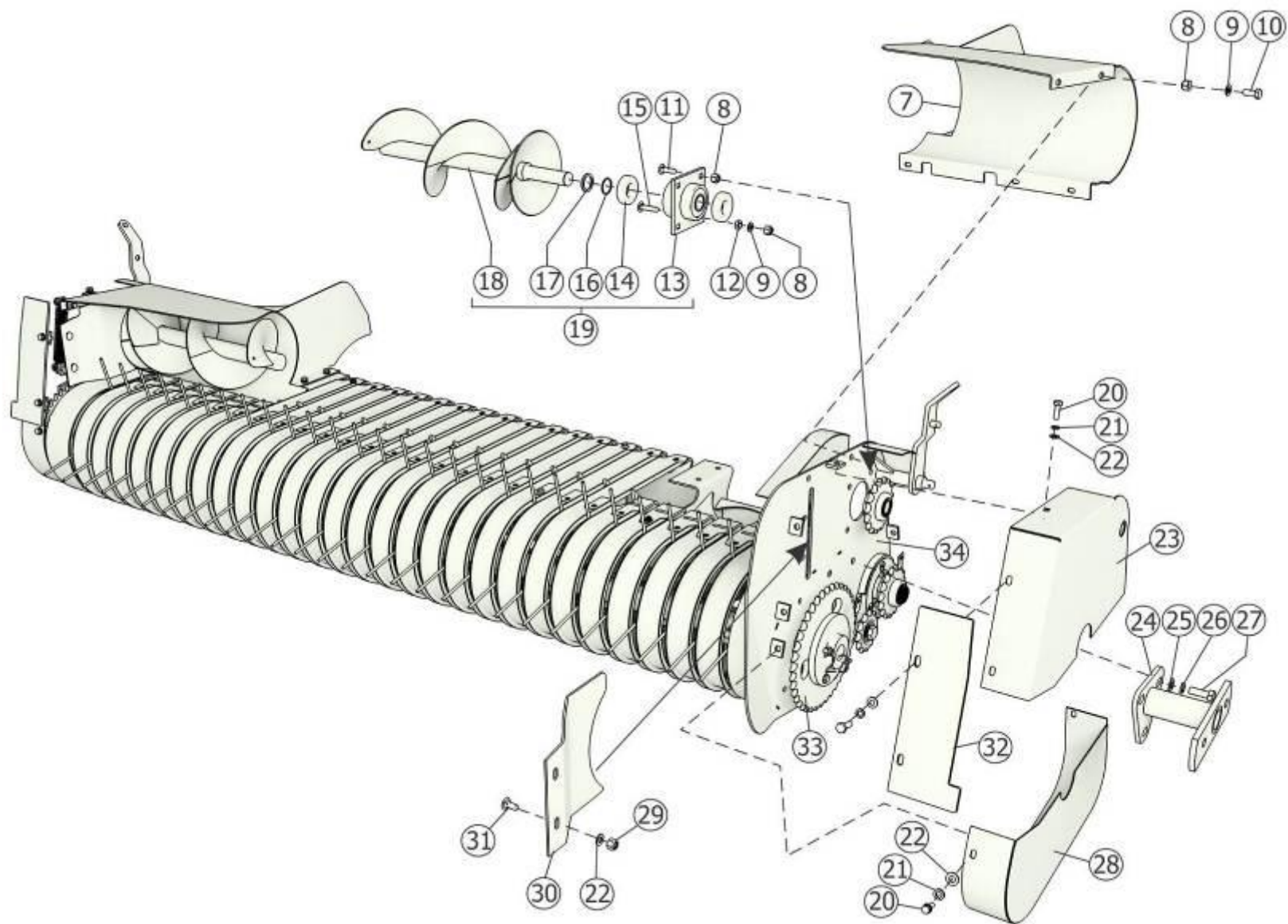
Рисунок 41 – Механизм подбирающий ППР-150.06.00.000Б
