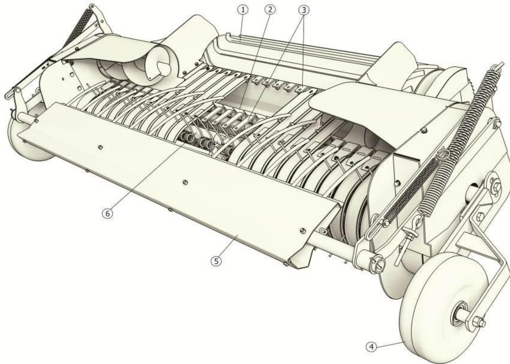
Рисунок 40 – Механизм подбирающий ППР-150.06.00.000Б
