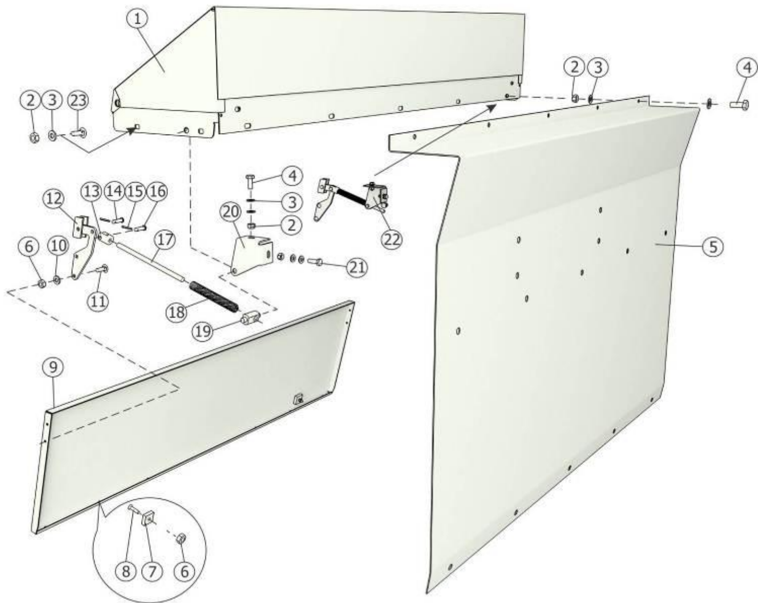
Рисунок 34 – Установка щитков передних ППР-150.11.01.100А
