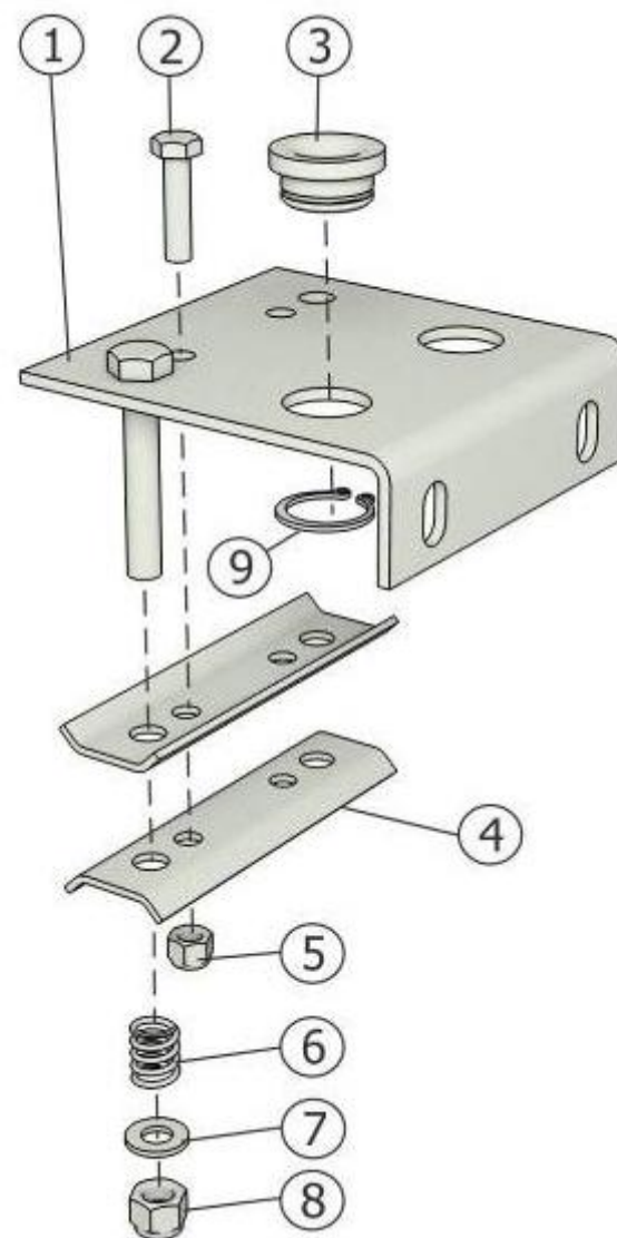
Рисунок 28 - Механизм натяжения шпегата ППР-150.10.00.160А
