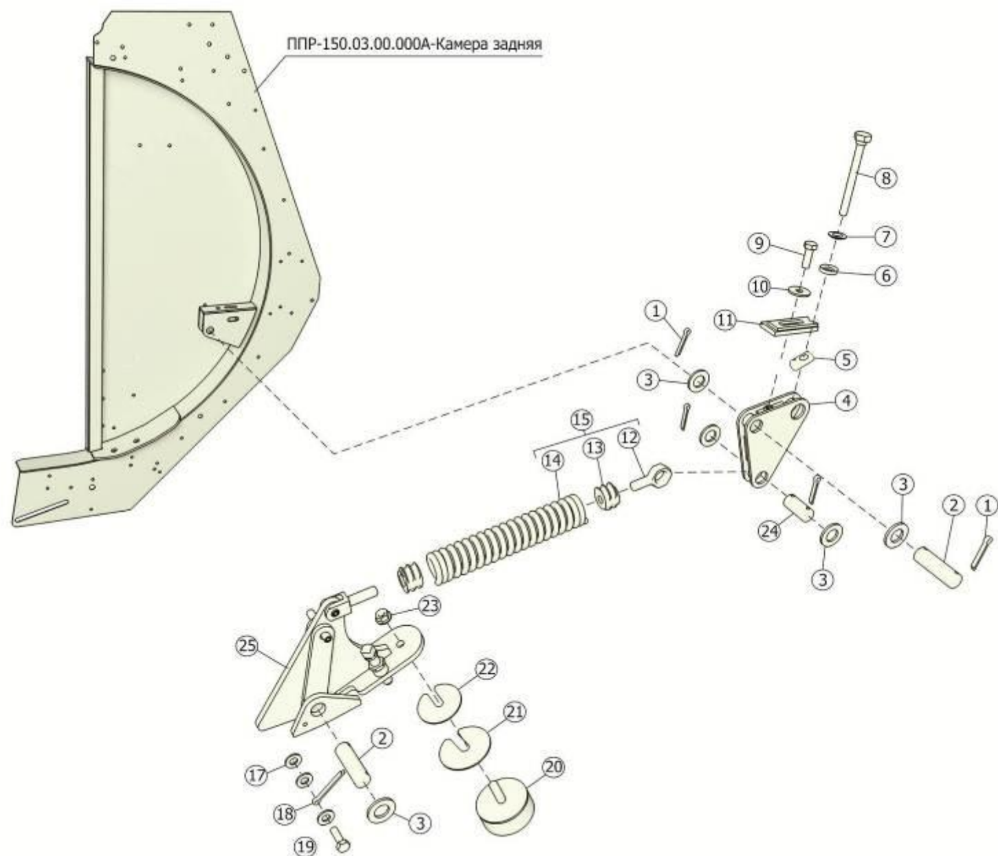
Рисунок 15 – Установка механизма закрывания задней камеры ППР-150.03.07.000В-01
