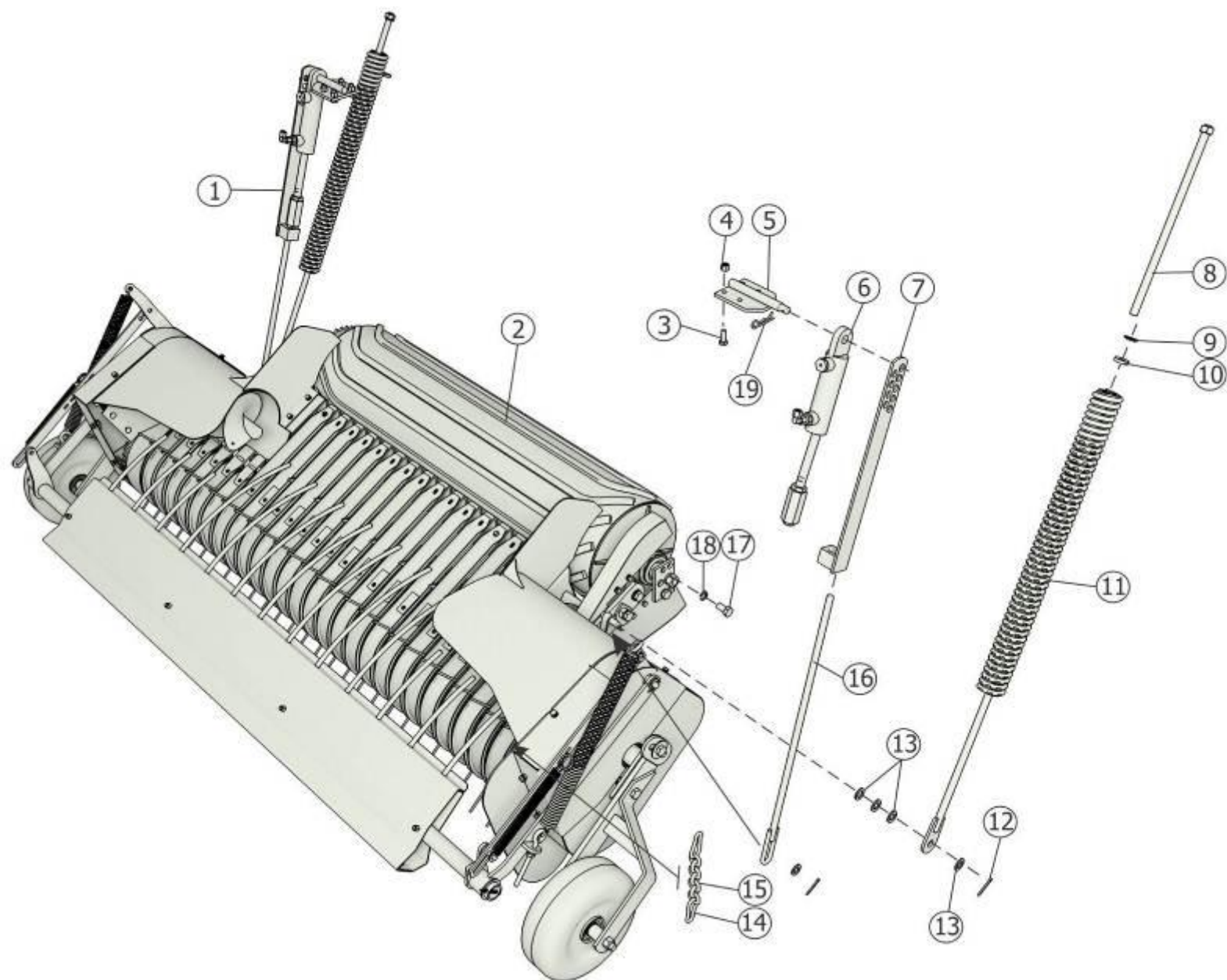
Рисунок 39 – Установка механизма подбирающего ППР-150.16.00.000А
