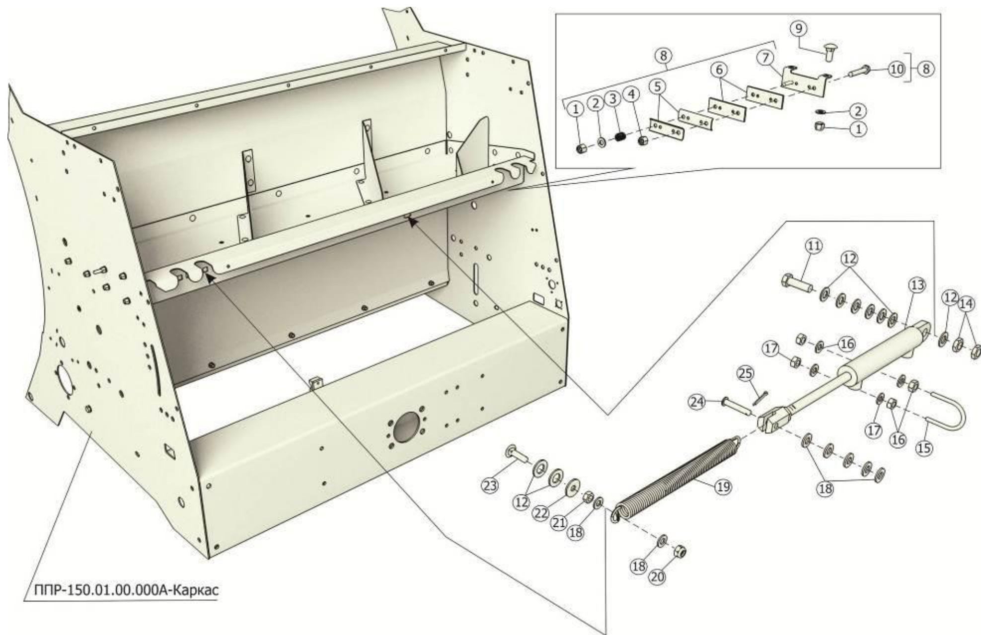
Рисунок 31 - Установка гидроцилиндра механизма обматывающего ППР-150.10.05.000А
