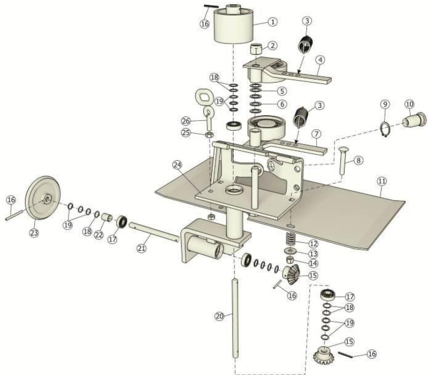
Рисунок 29 - Привод механизма обматывающего ППР-150.10.02.000А
