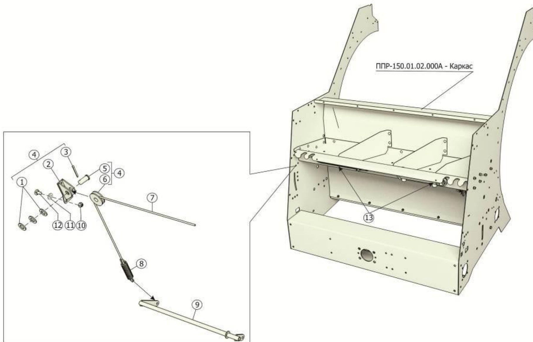
Рисунок 30 - Установка шпегата механизма обматывающего ППР-150.10.00.020А
