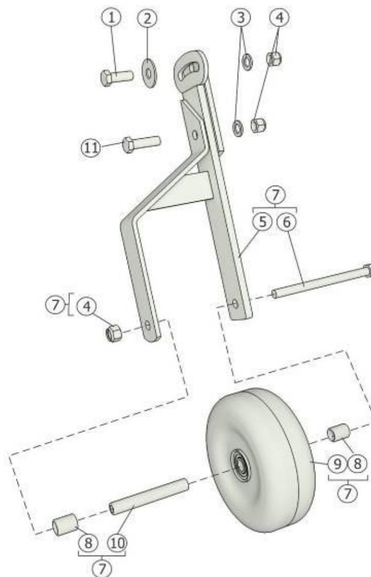
Рисунок 48 –Колесо ППР-150.06.06.000А
