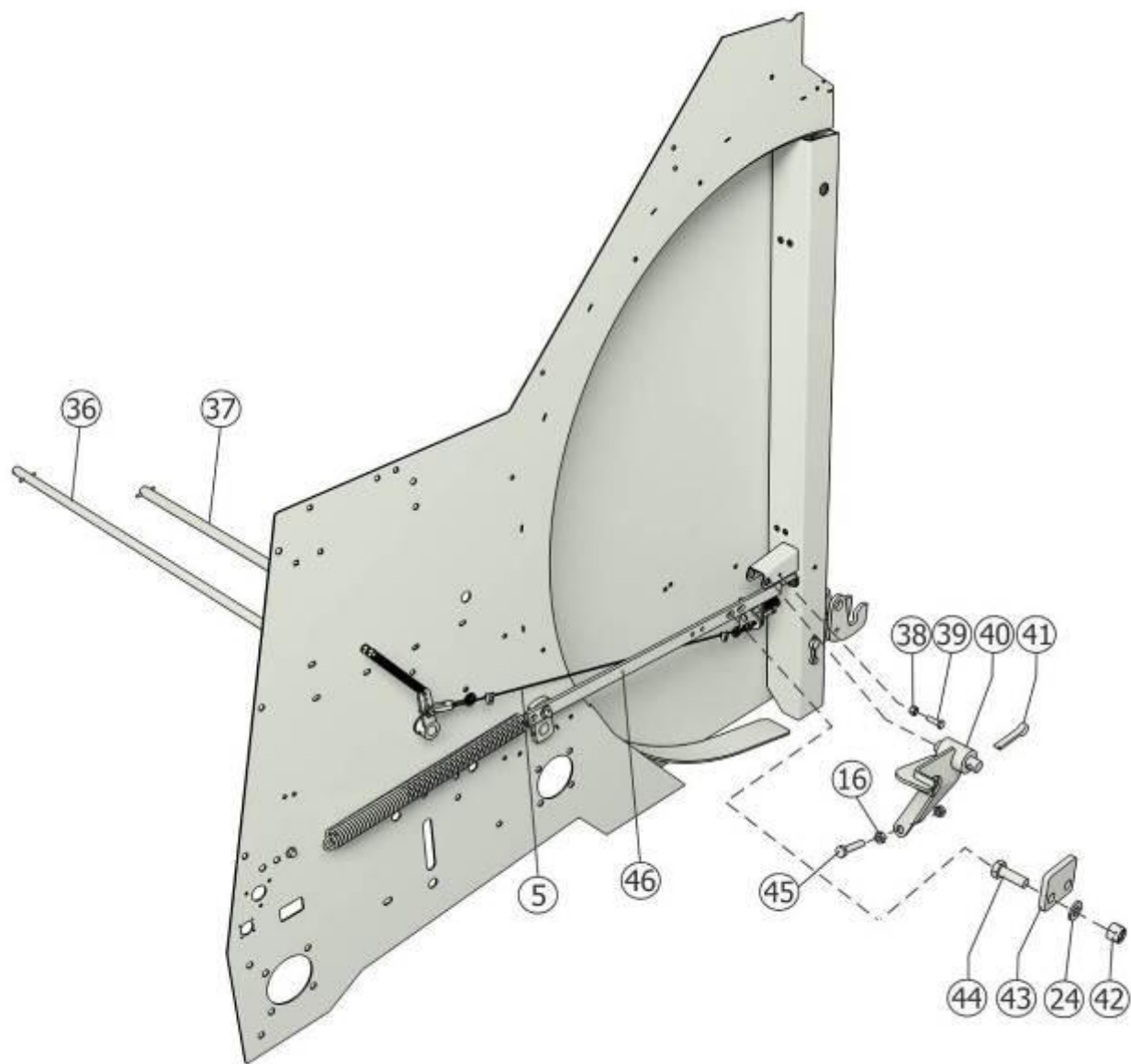
Рисунок 12 – Механизм регулирования плотности прессования ППР-150.01.06.000А. Вид слева
