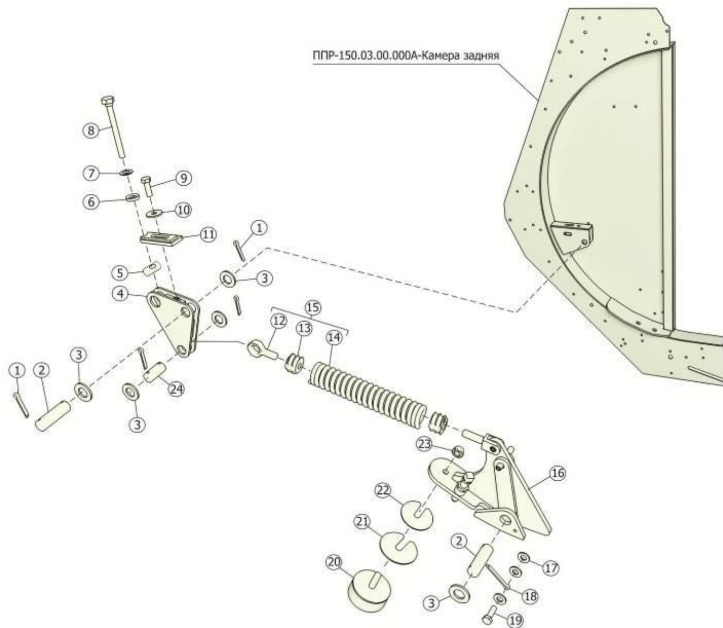
Рисунок 14 – Установка механизма закрывания задней камеры ППР-150.03.07.000В
