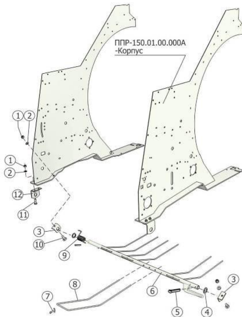
Рисунок 5 – Нормализатор ППР-150.01.00.150А
