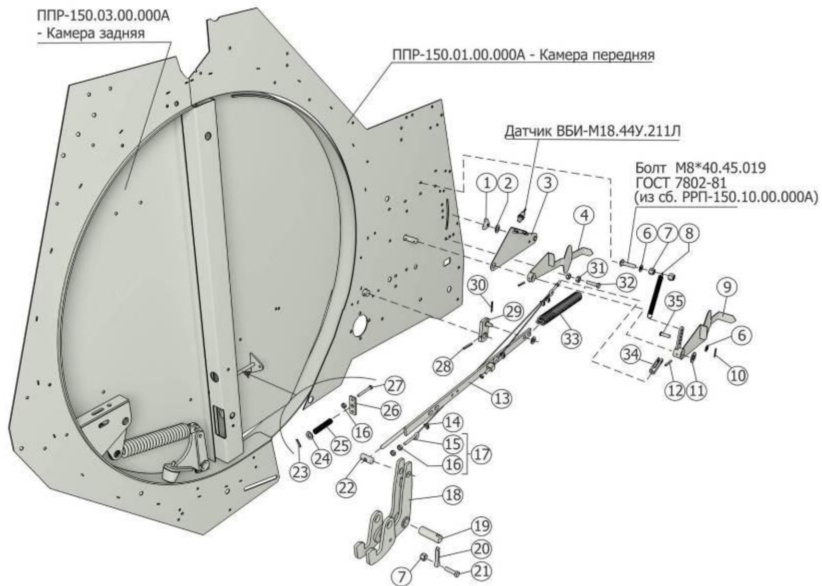
Рисунок 11 – Механизм регулирования плотности прессования ППР-150.01.06.000А. Вид справа
