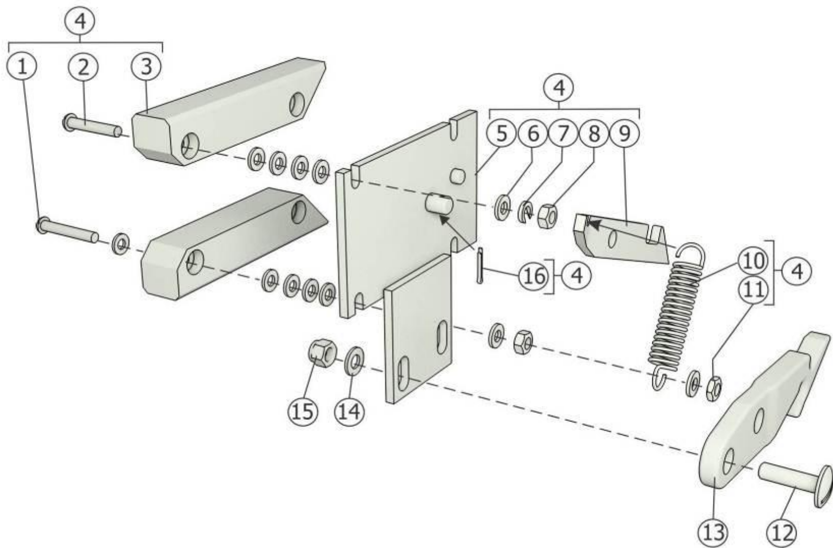
Рисунок 26 – Каретка ППР-150.10.03.000А
