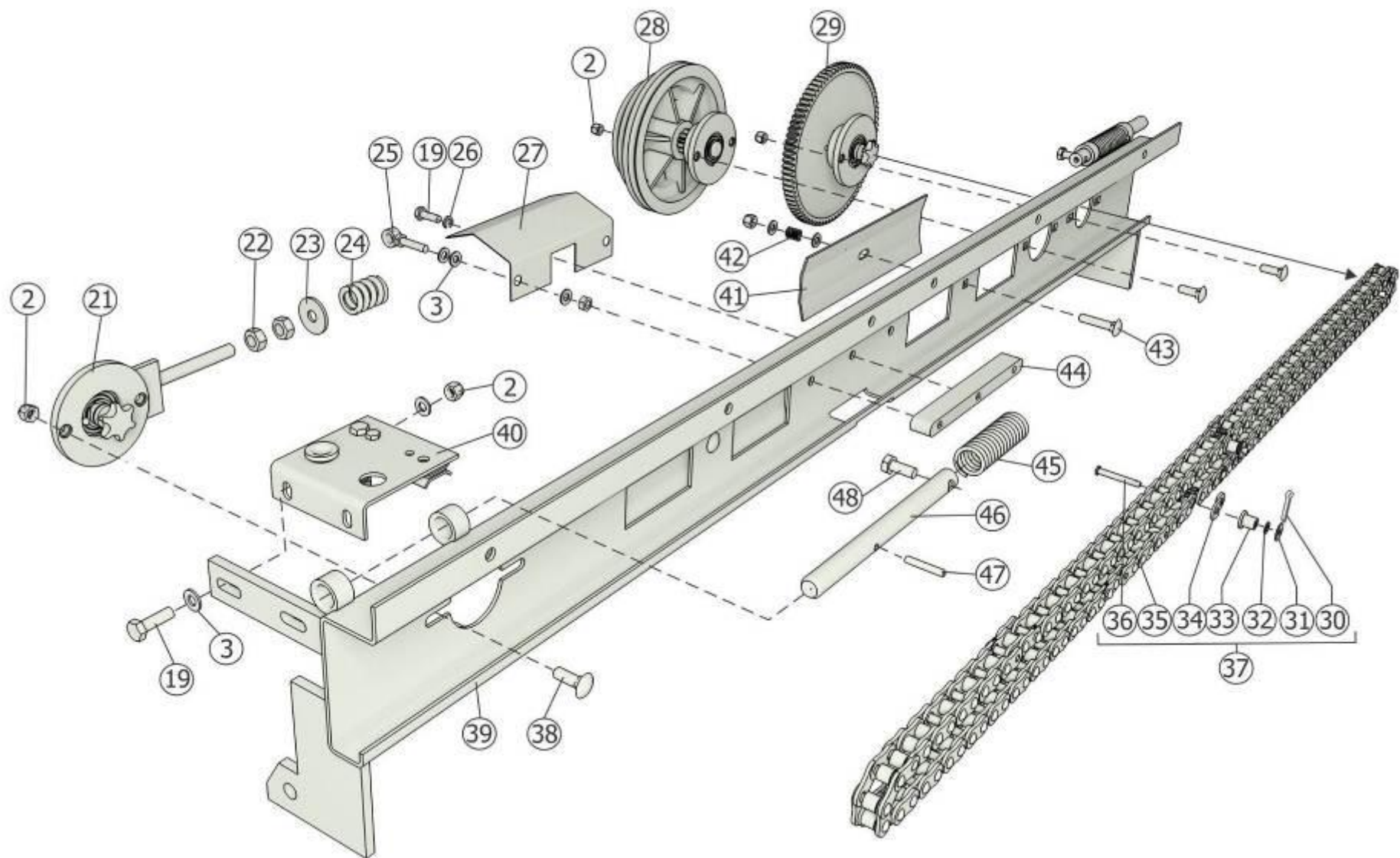
Рисунок 25 – Механизм обматывающий ППР-150.10.00.010А. Вид справа
