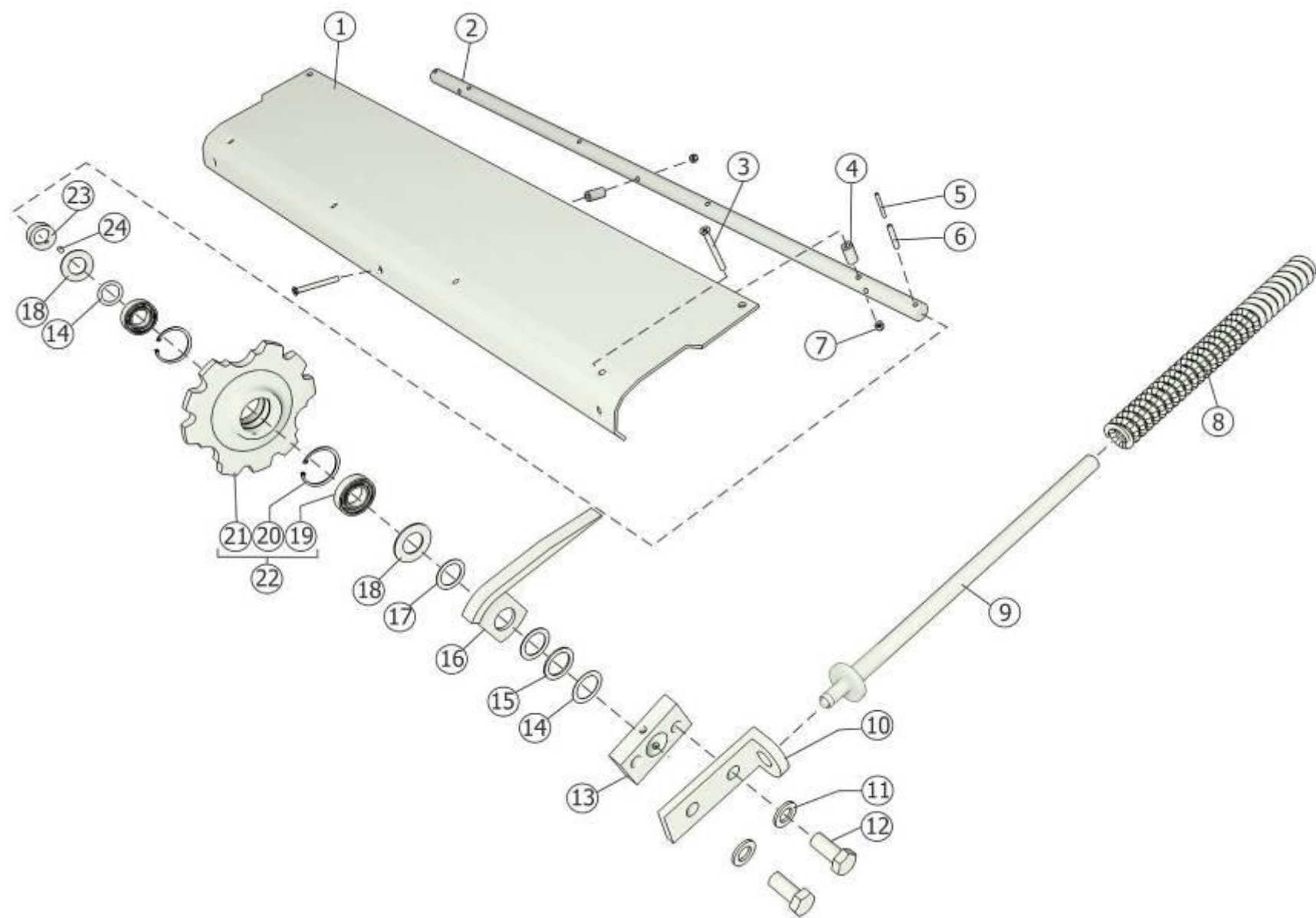
Рисунок 17 – Вал транспортера нижний 150.03.04.000А
