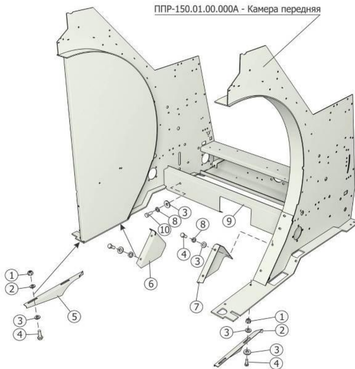
Рисунок 36 – Установка щитков внутренних ППР-150.11.01.300
