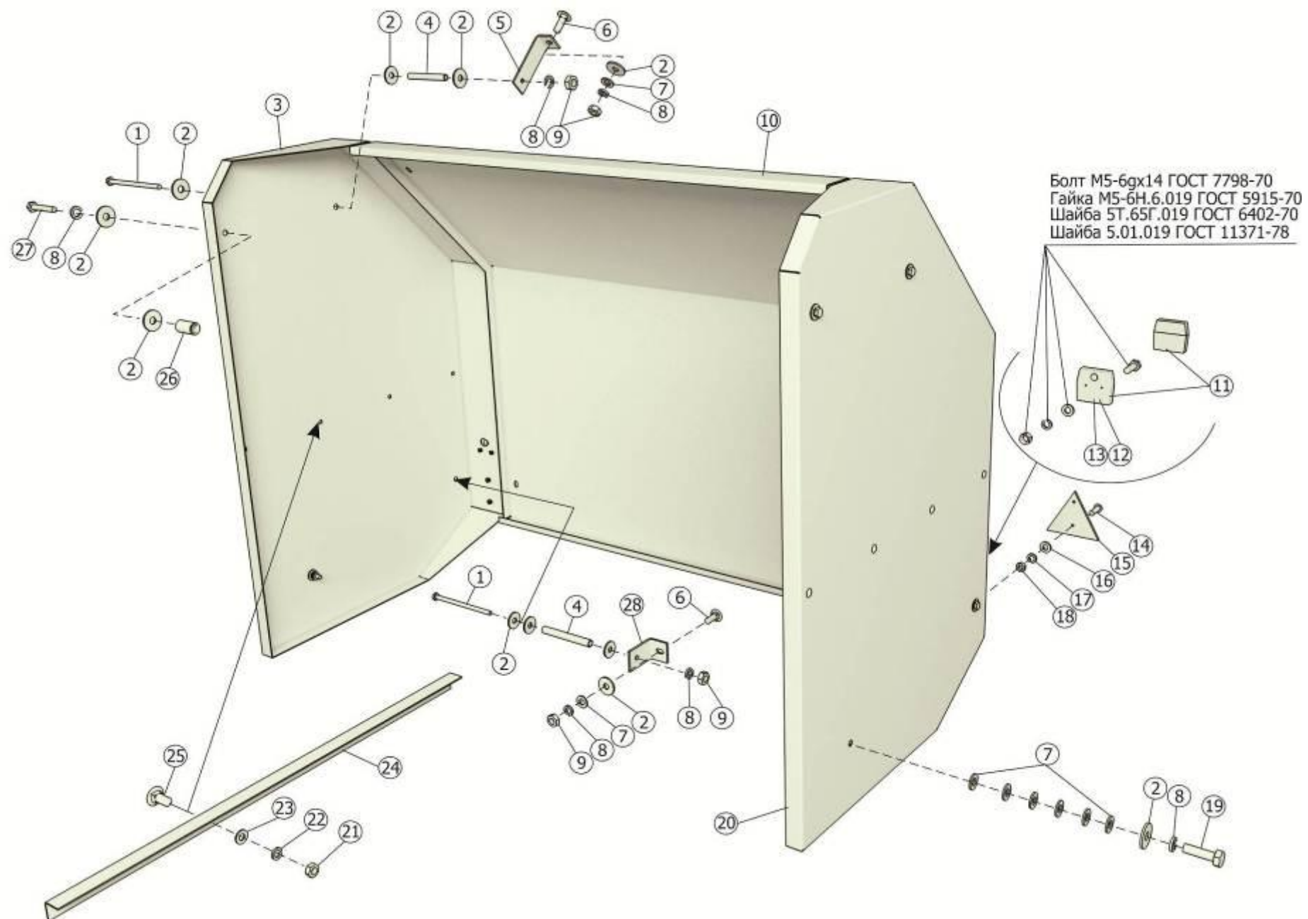
Рисунок 37 – Установка щитков задних ППР-150.11.03.000А
