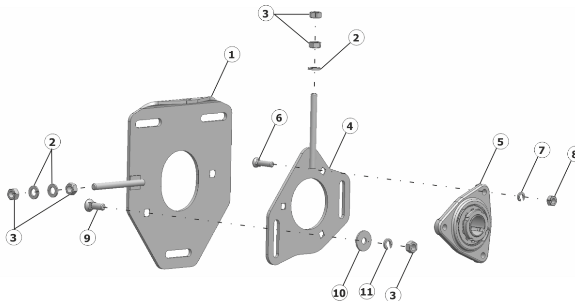
Рисунок 13 – Плита в сборе SS-1050.01.01.690A
