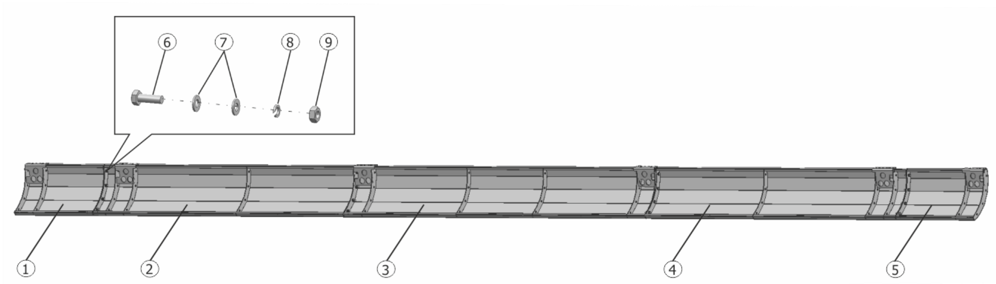
Рисунок 21 – Щиток SS-780.01.11.100
