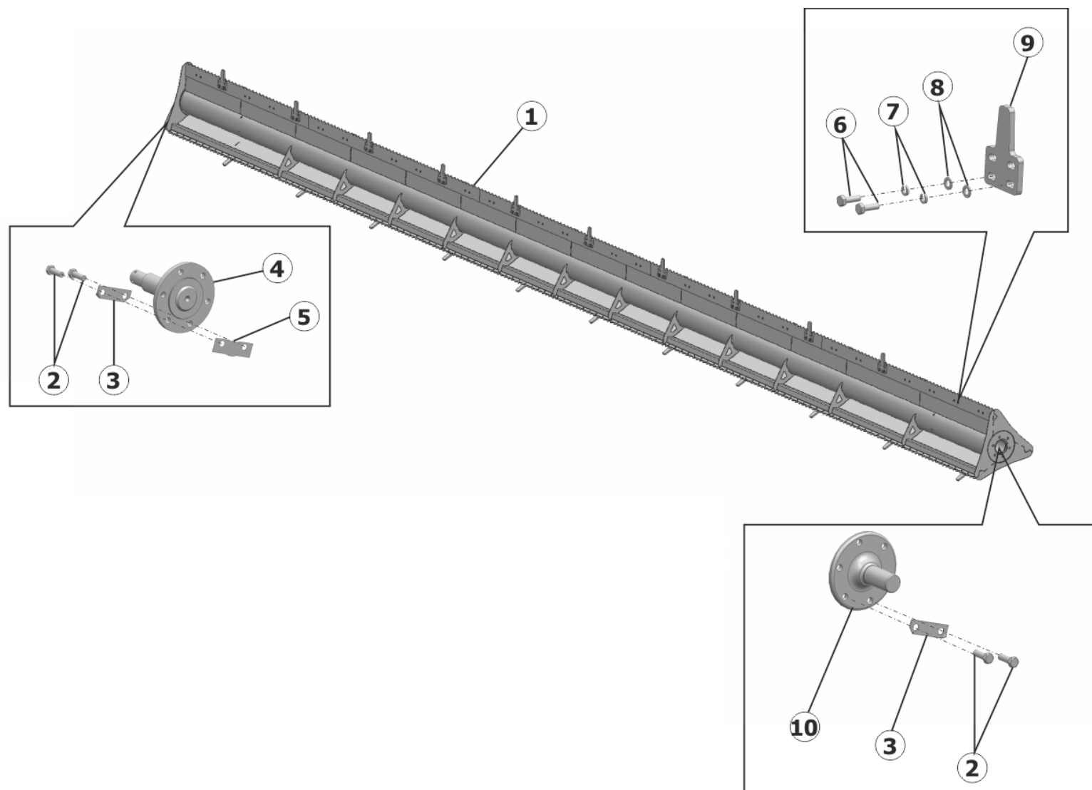
Рисунок 4 – Мотовило SS-780.01.04.000
