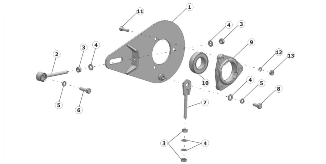
Рисунок 14 – Плита в сборе SS-1050.01.01.490A
