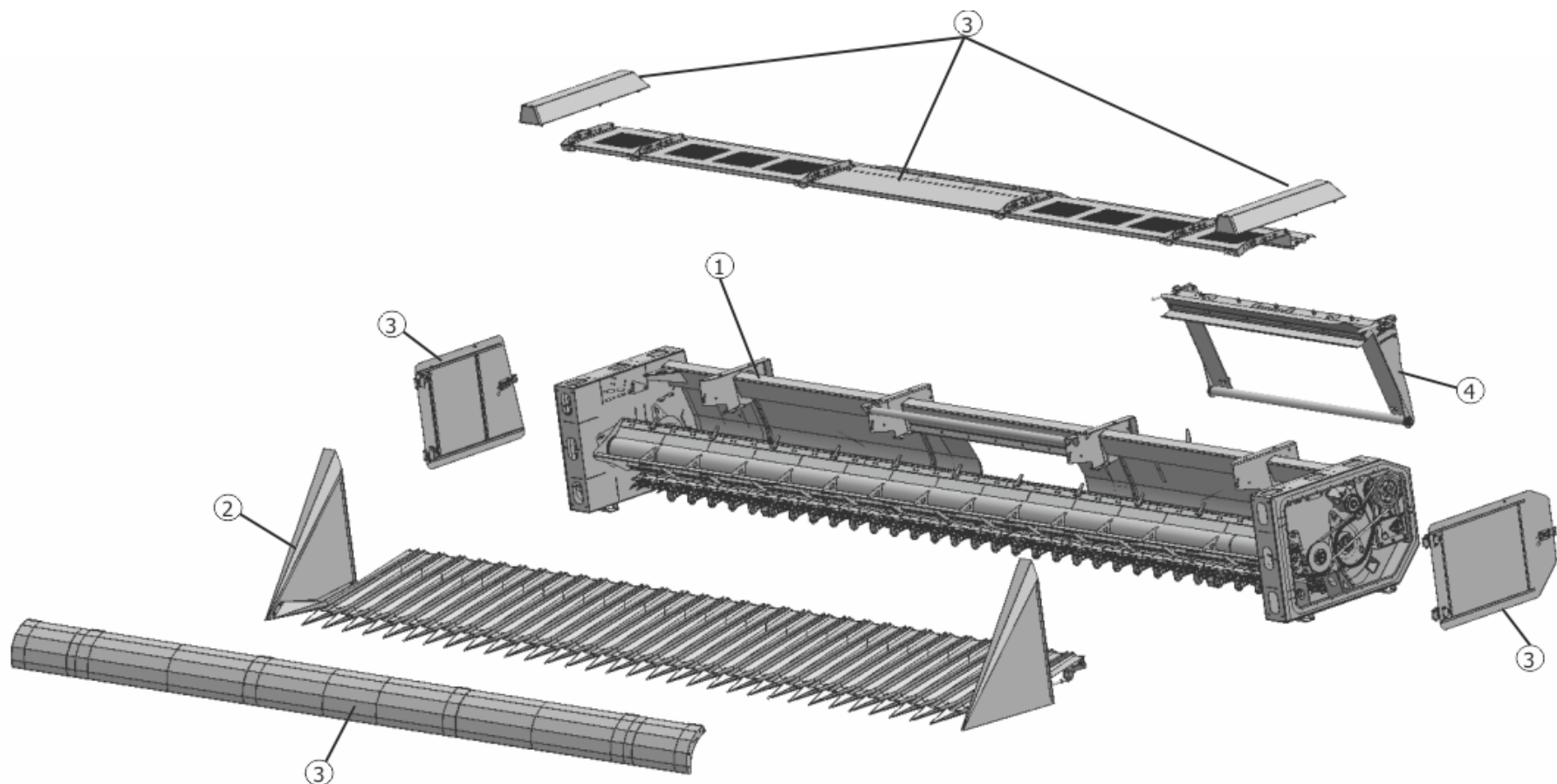
Рисунок 2 – Жатвенная часть SS-780.01.00.000
