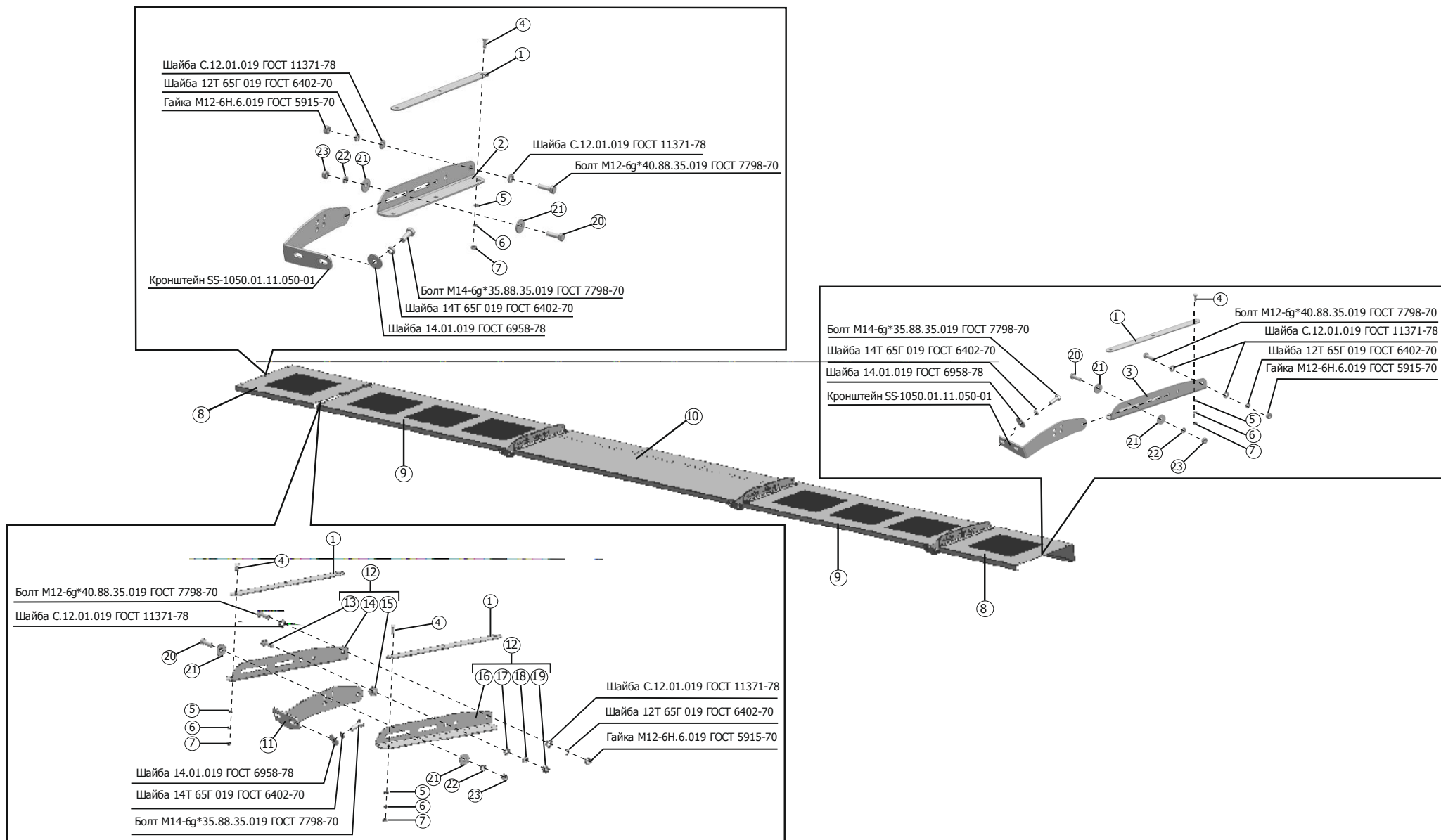
Рисунок 20 – Установка щитов SS-780.01.11.010
