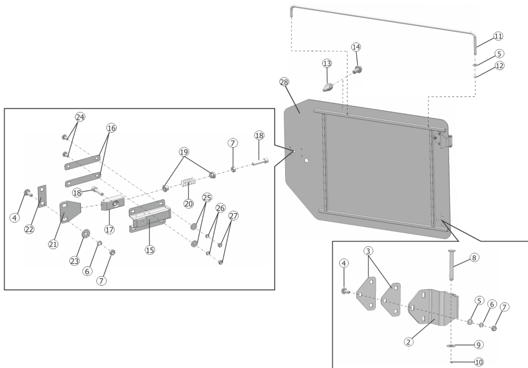
Рисунок 23 – Дверь левая SS-920.01.11.510
