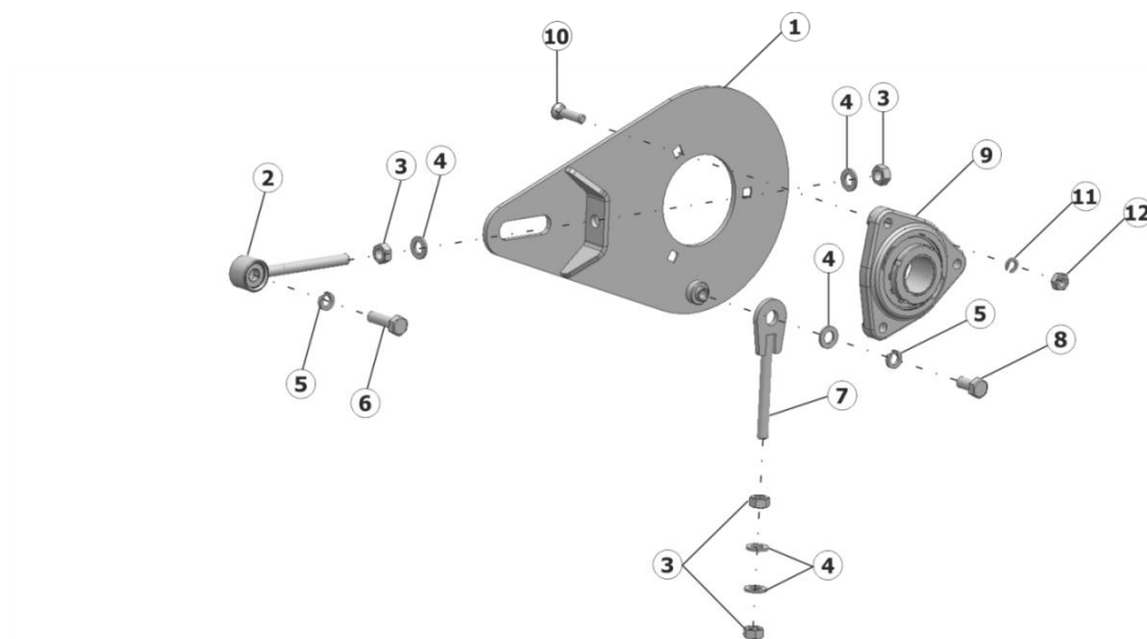
Рисунок 7 – Плита в сборе SS-1050.01.01.490A-01
