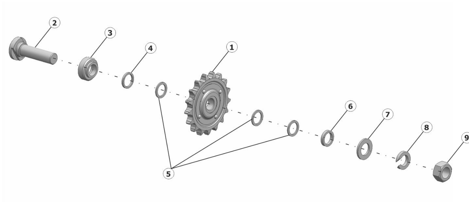
Рисунок 11 – Звездочка натяжная SS-1050.01.01.740
