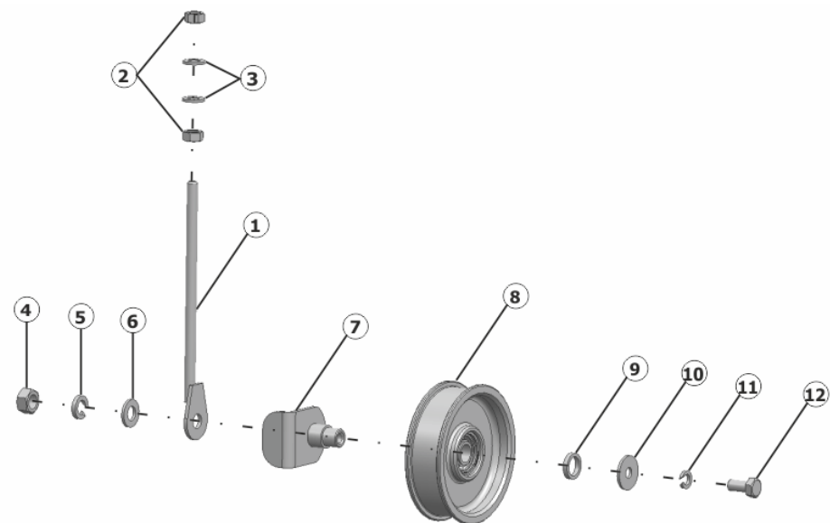
Рисунок 16 – Шкив в сборе SS-1050.01.01.210
