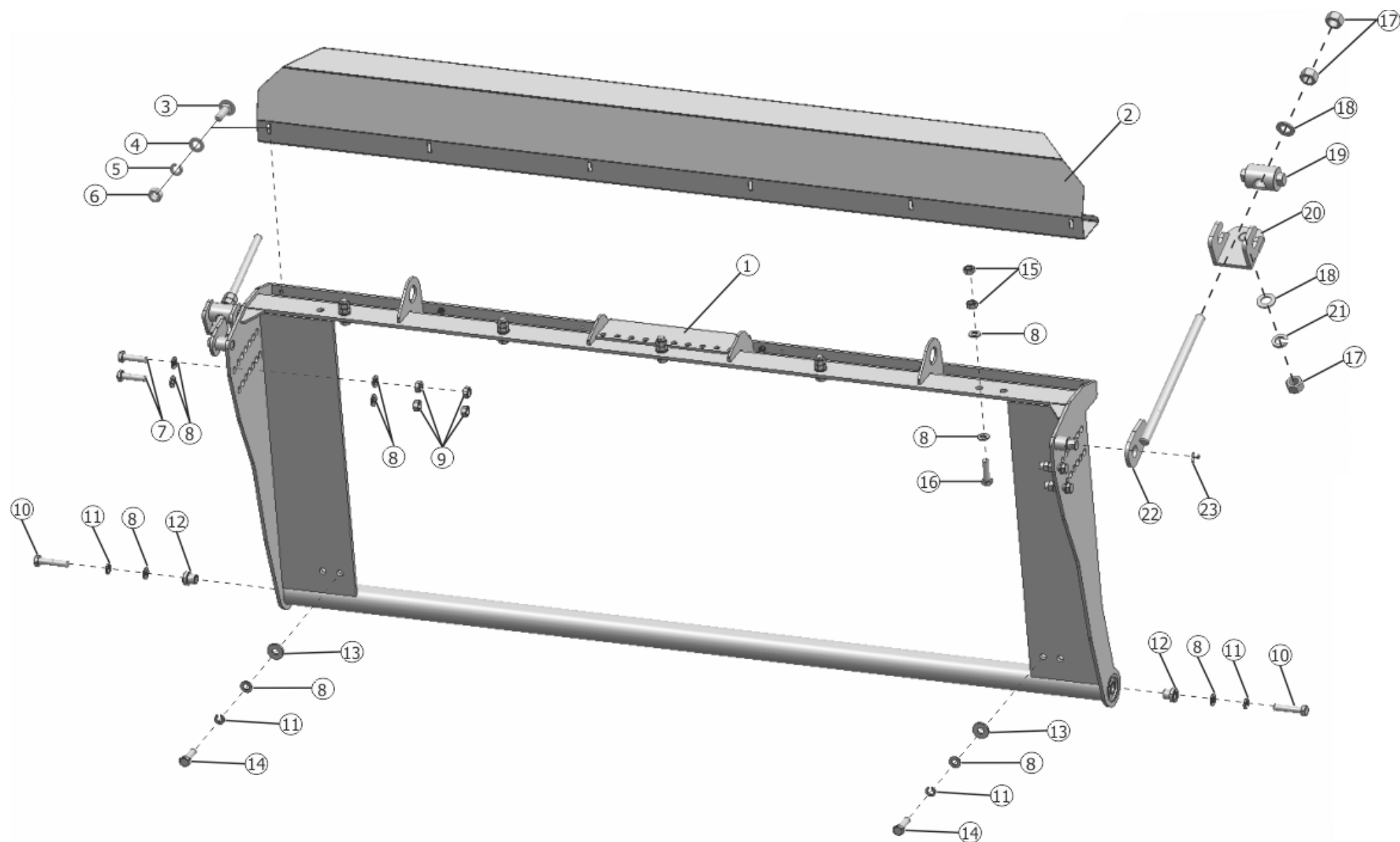
Рисунок 24 – Рамка основная SS-1050.01.00.550
