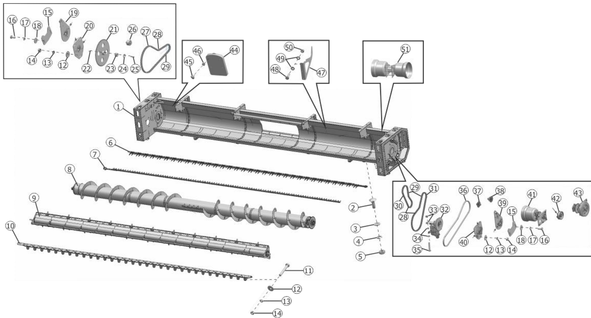
Рисунок 3 – Корпус жатки SS-780.01.01.000
