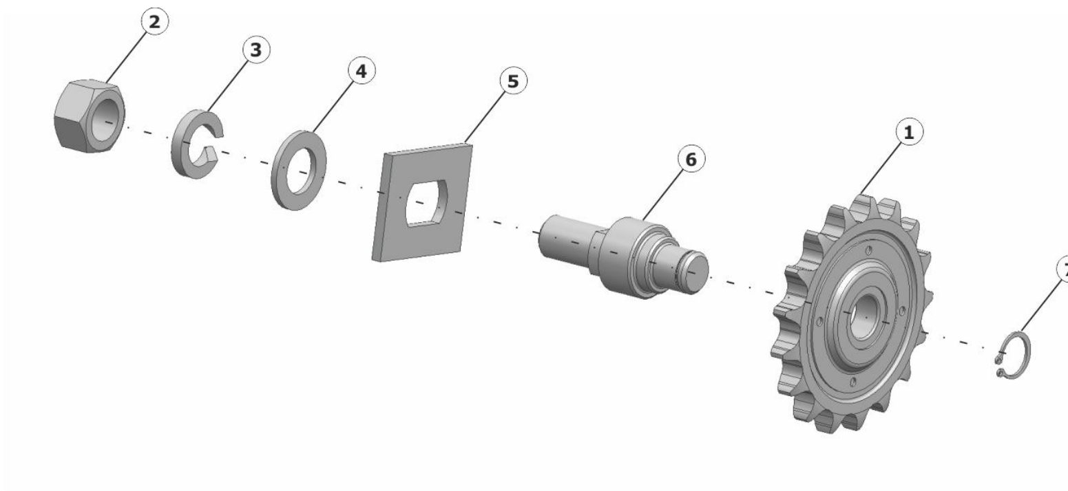
Рисунок 12 – Звездочка натяжная SS-1050.01.01.750
