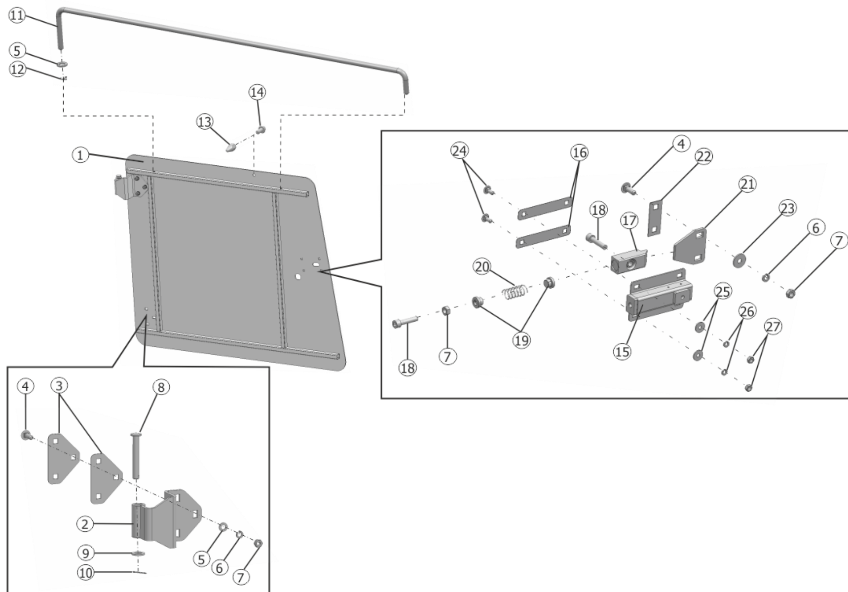
Рисунок 22 – Дверь правая SS-920.01.11.490
