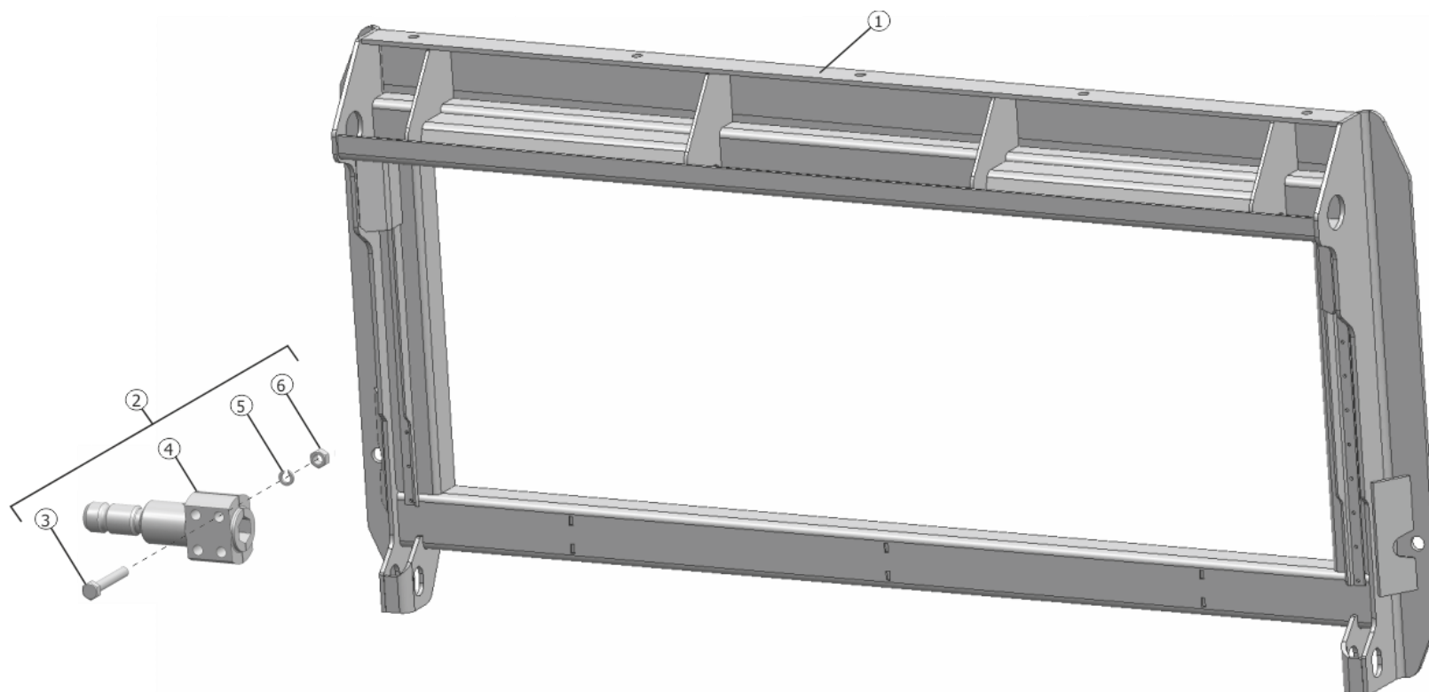
Рисунок 30 – Рамка переходная (John Deere) SS-1050.85.00.000
