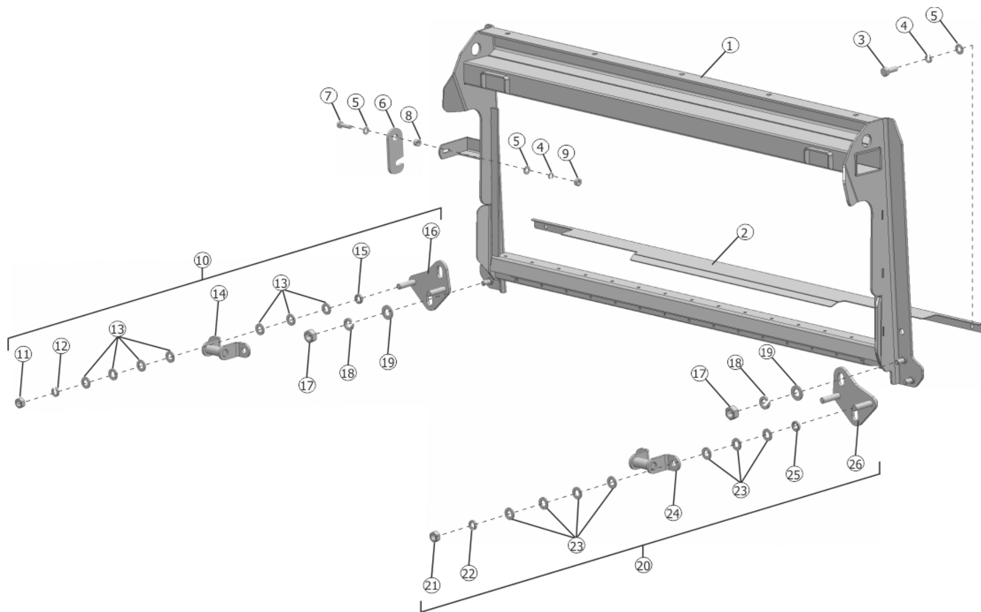
Рисунок 29 – Рамка переходная (New Holland) SS-1050.80.00.000
