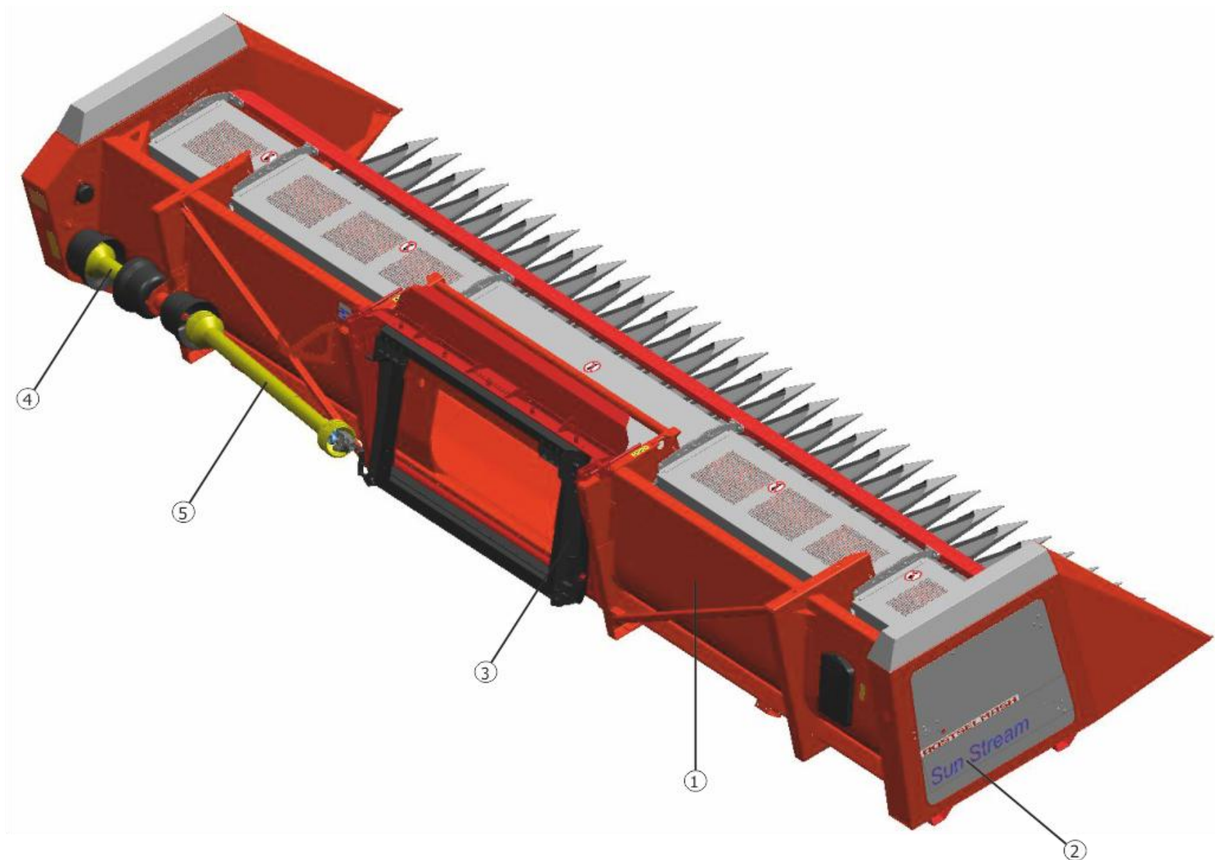
Рисунок 1 – Жатка для уборки подсолнечника безрядковая "Sun Stream" RSM SS-780
