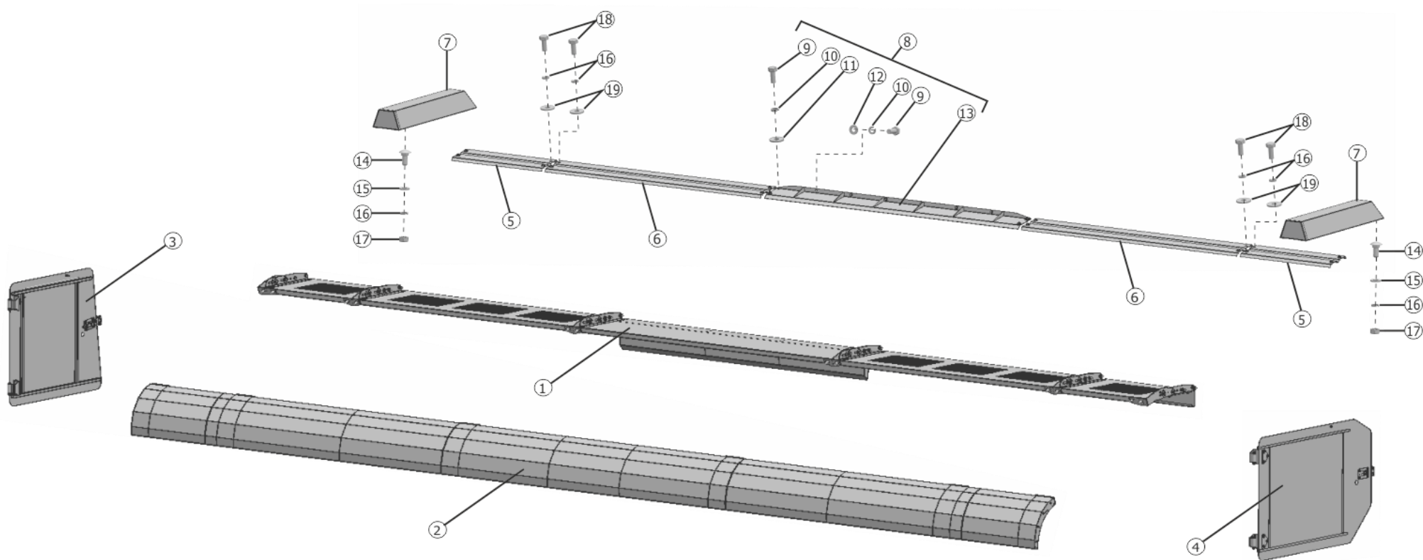
Рисунок 19 – Установка ограждений SS-780.01.11.000
