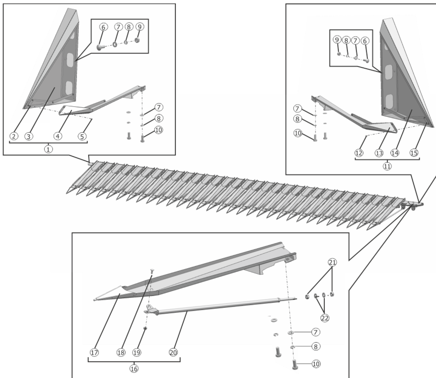
Рисунок 18 – Установка делителей SS-780.01.03.000
