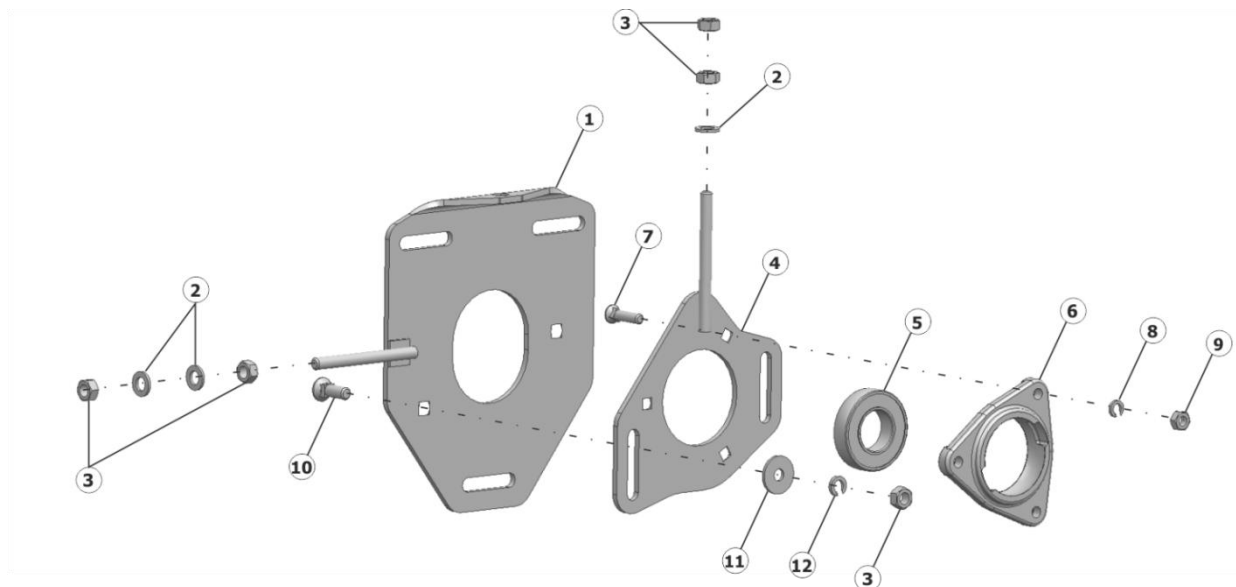
Рисунок 9 – Плита в сборе SS-1050.01.01.690A-01
