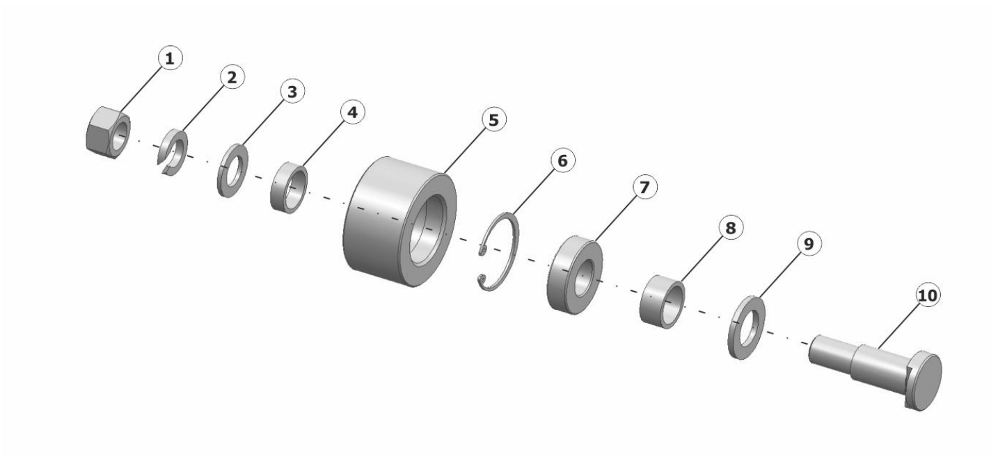
Рисунок 8 – Ролик натяжной SS-1050.01.01.540A
