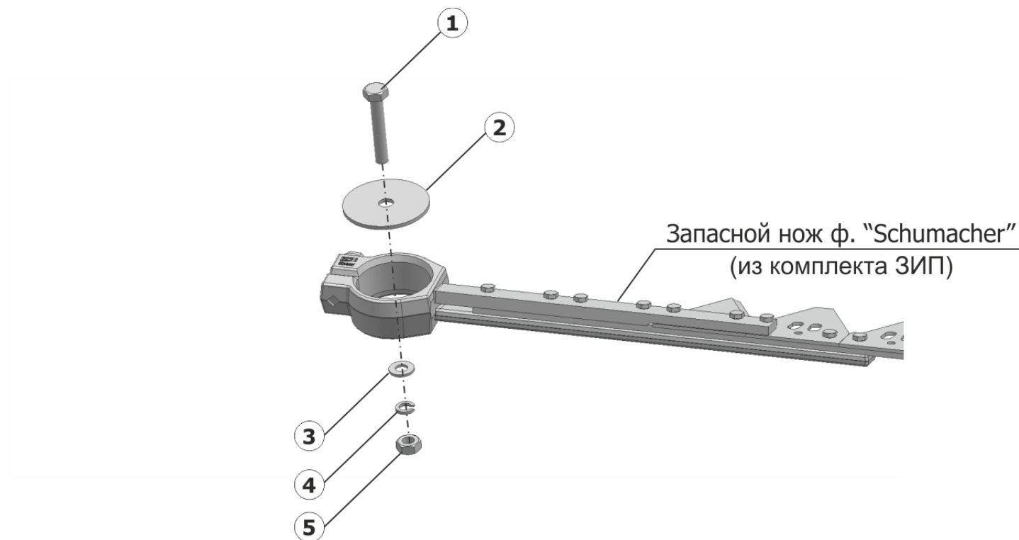
Рисунок 6 - Установка запасного ножа SS-780.12.00.020
